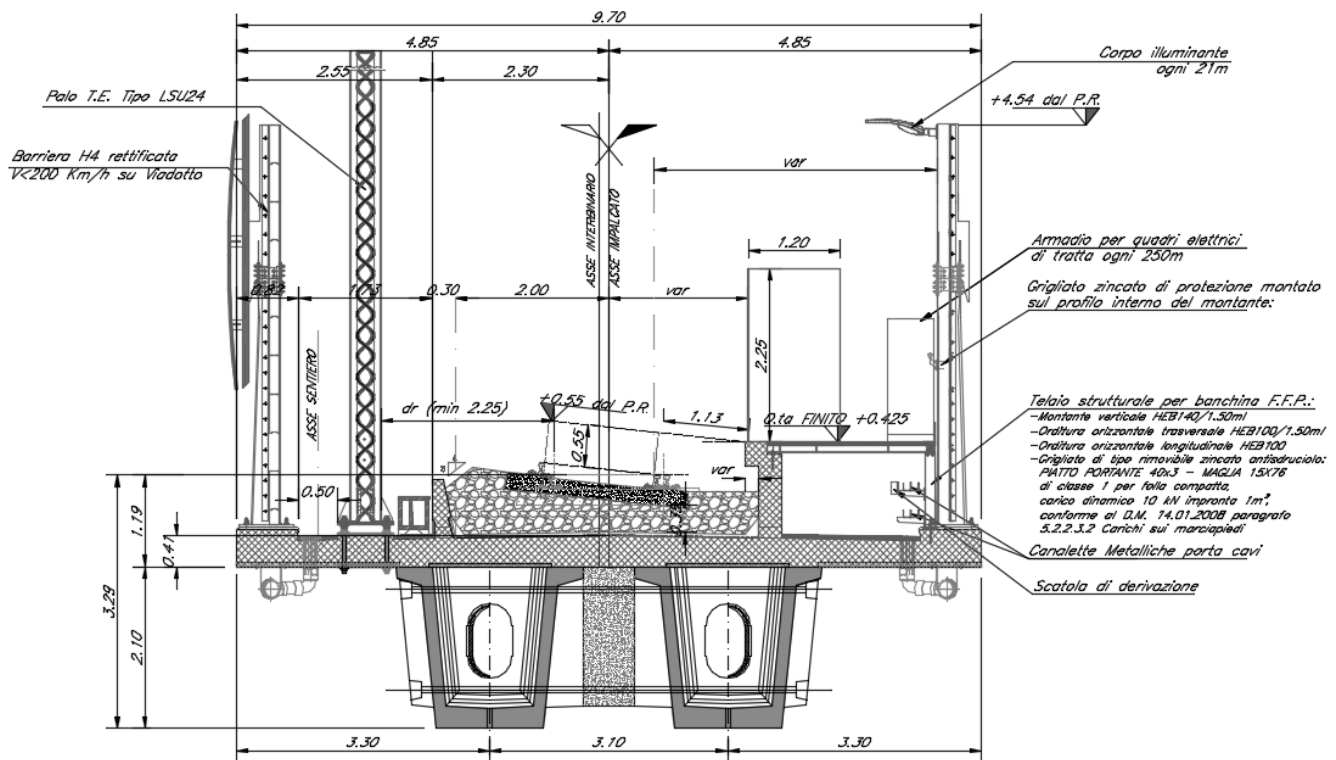
Figura 1 –sezione trasversale
