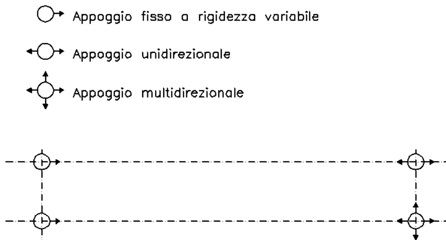
Figura 3 –Schema appoggi
