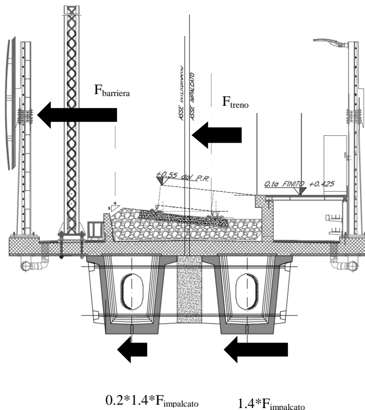
Figura 19 – schema di applicazione dell'azione del vento
