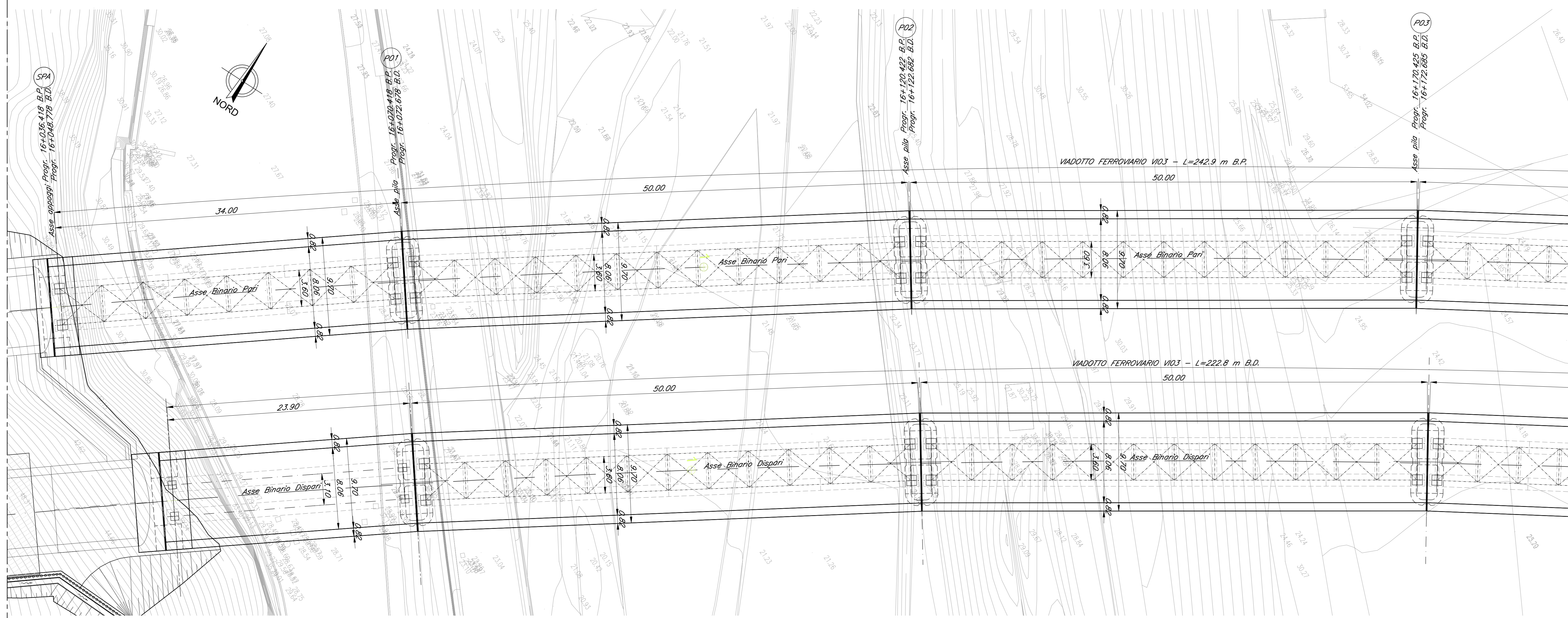
PIANTA TRAVI Scala 1:200
