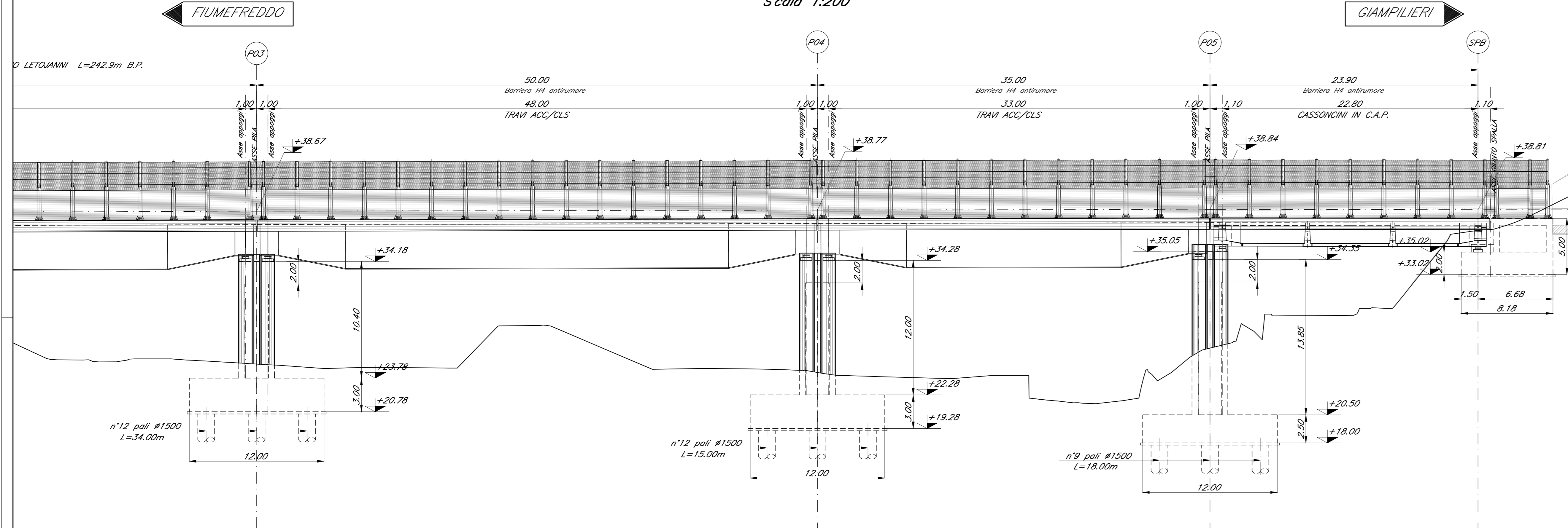
PROSPETTO BINARIO PARI Scala 1:200
