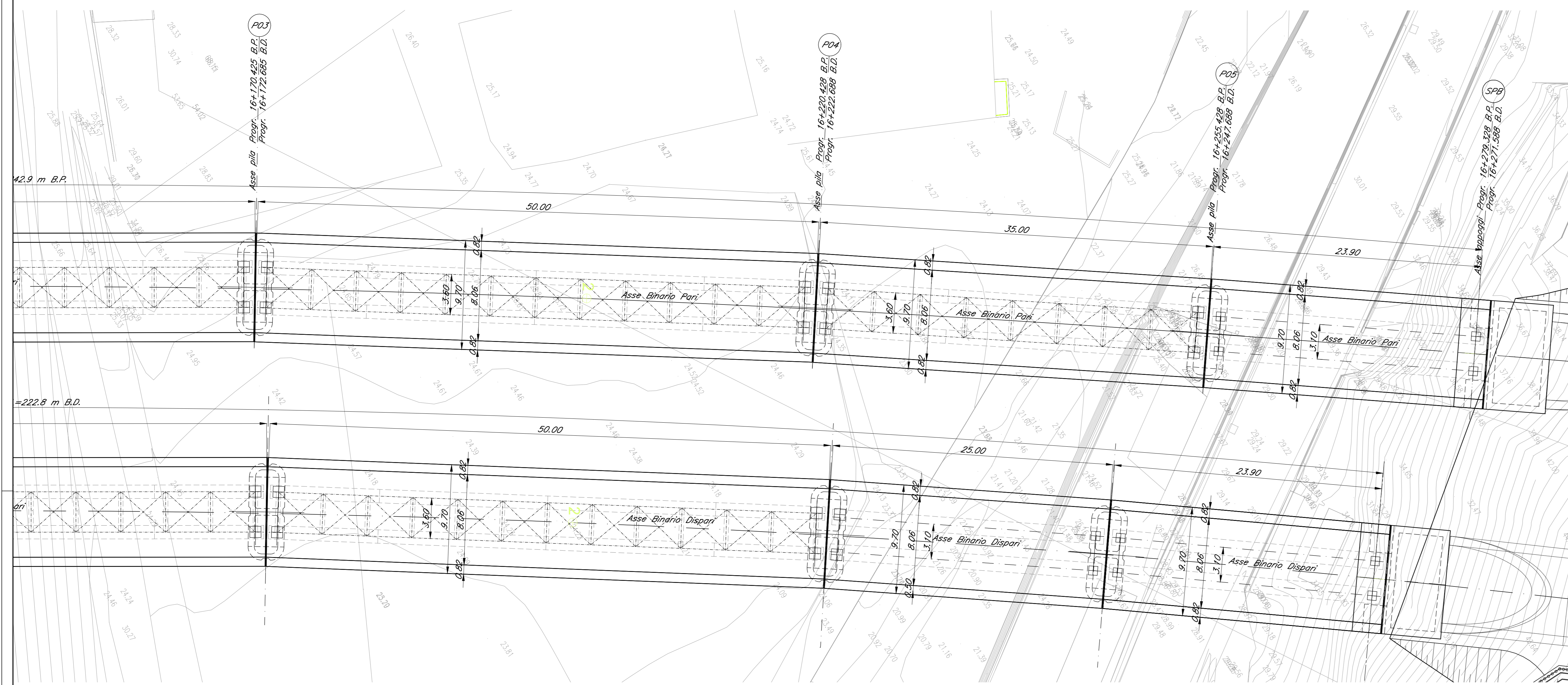
PIANTA TRAVI Scala 1:200
