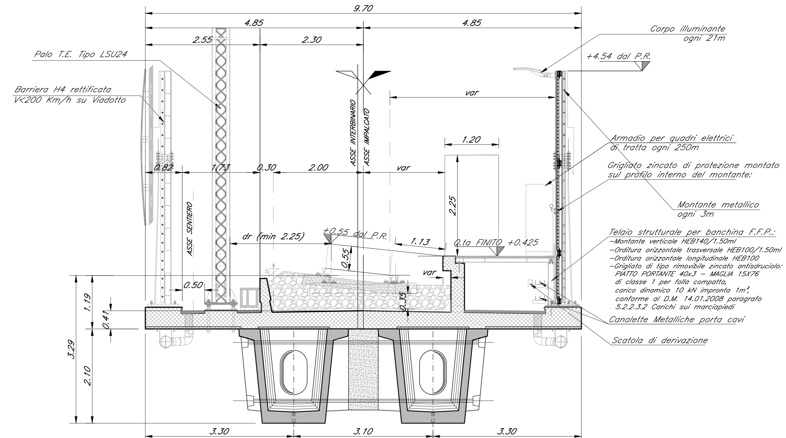
SEZIONE TIPO BINARIO PARI CAMPATA IN C.A.P. Scala 1:50
