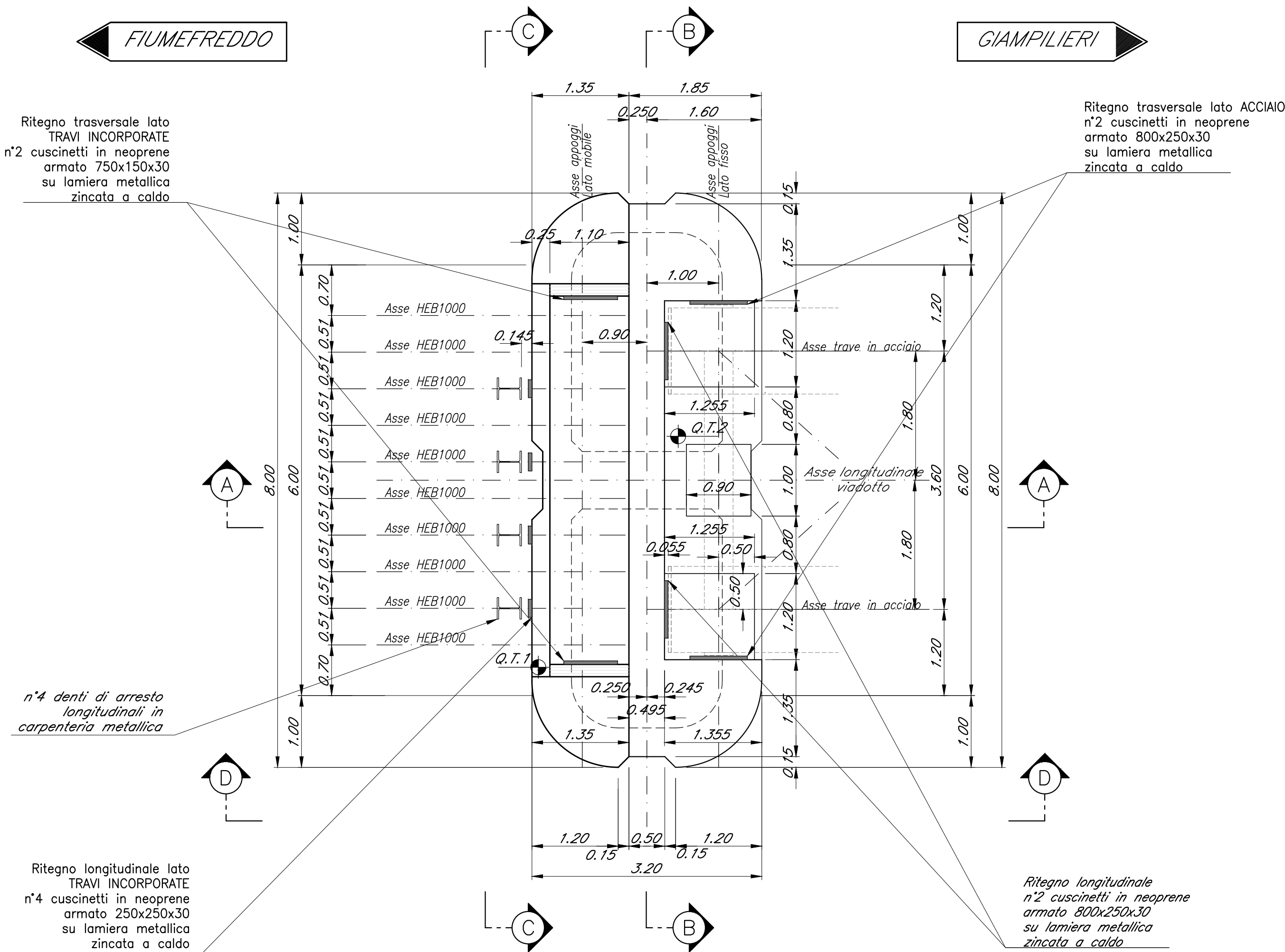
SEZIONE F-F Scala 1:50
