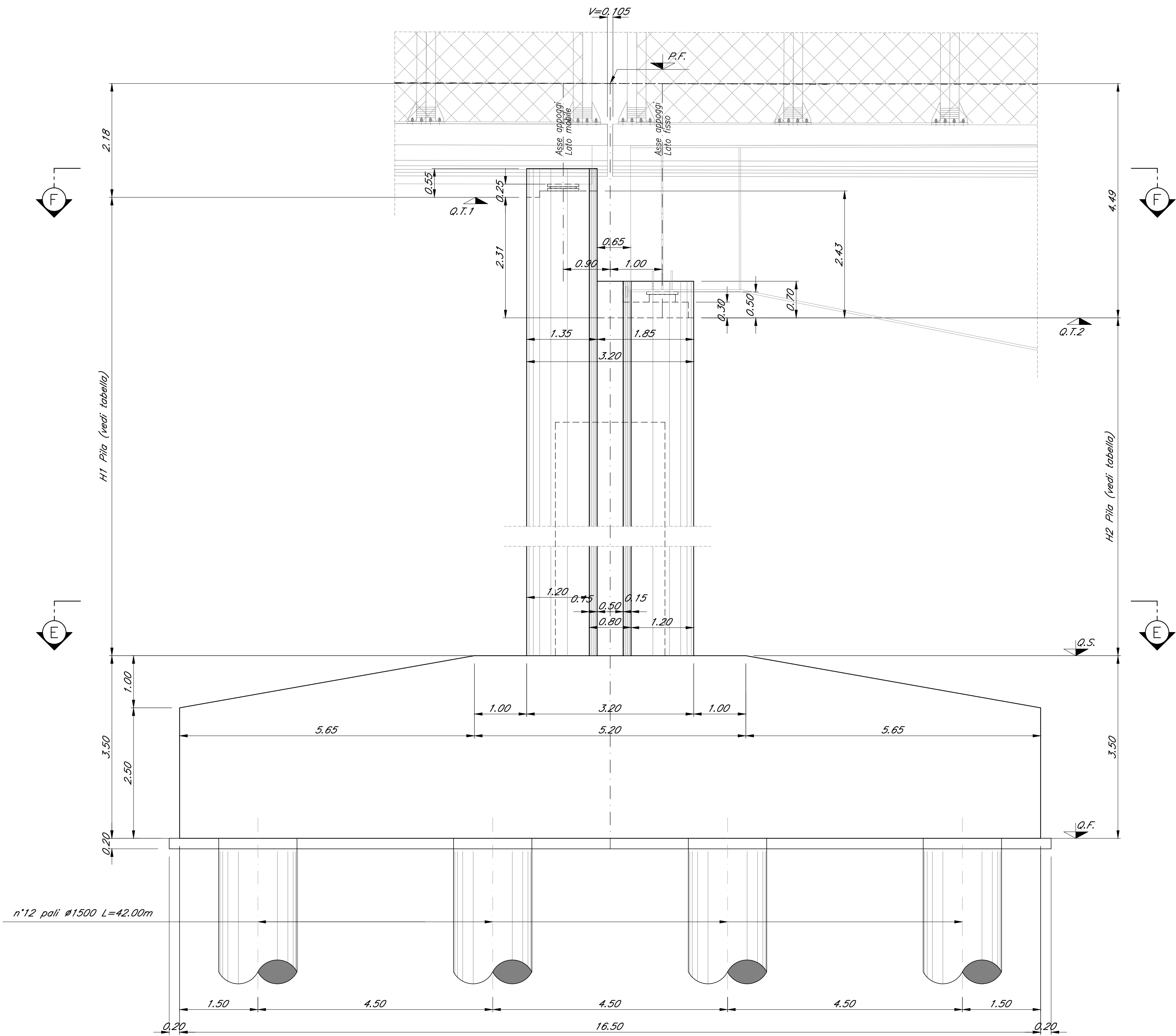
VISTA D-D Scala 1:50
