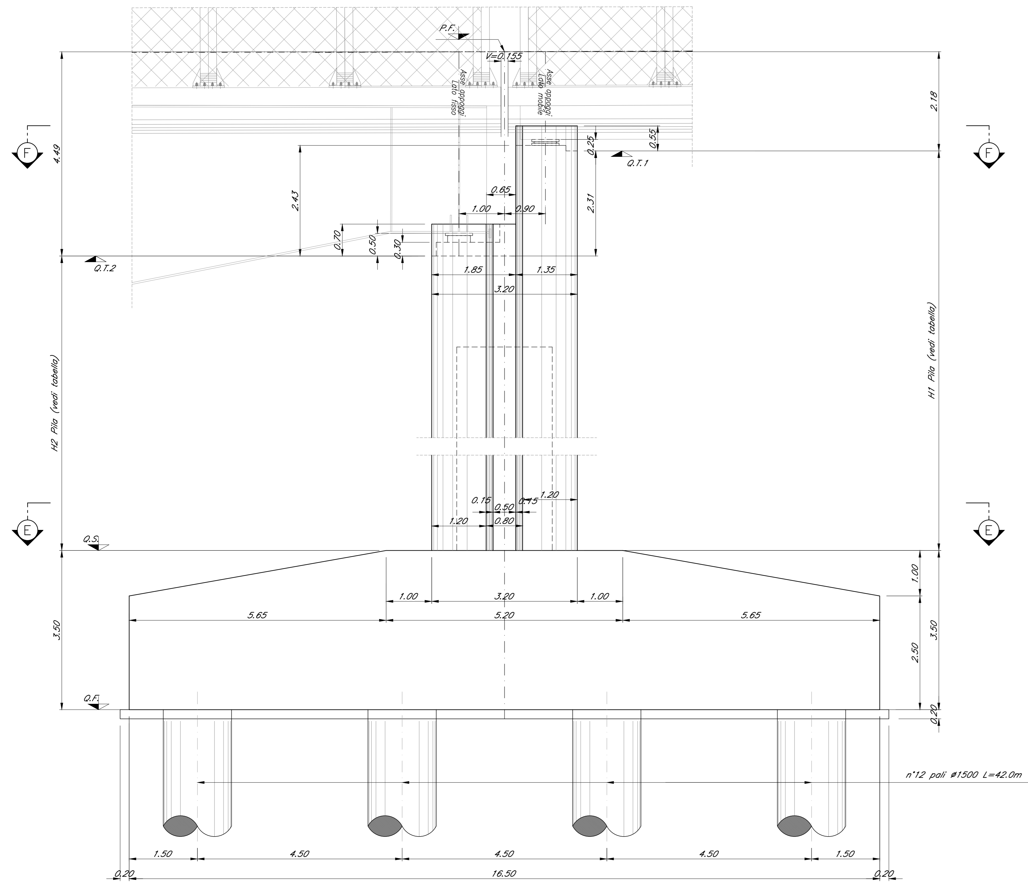
SEZIONE F-F Scala 1:50
