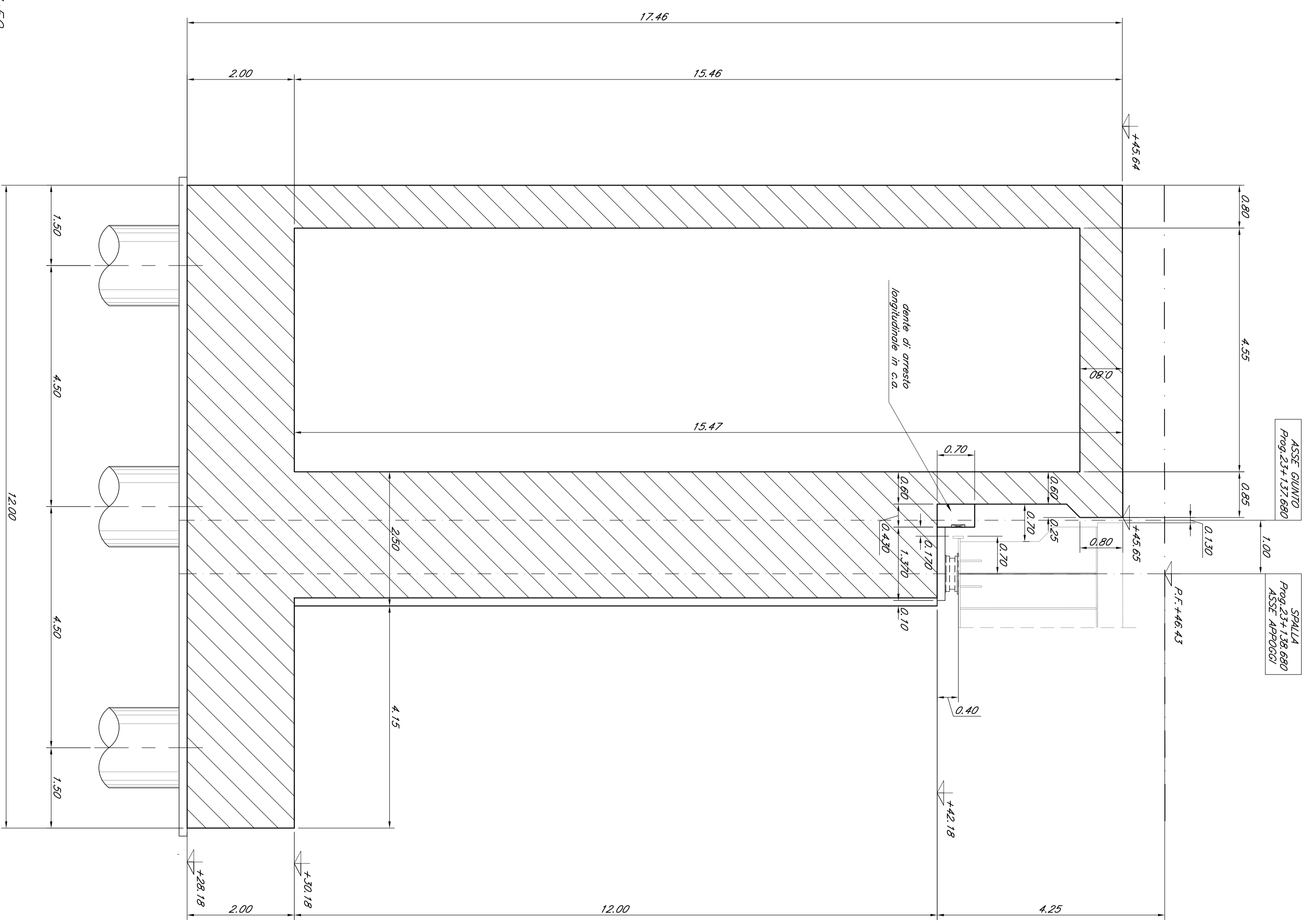
VISTA SUPERIORE E-E Scala 1:50
