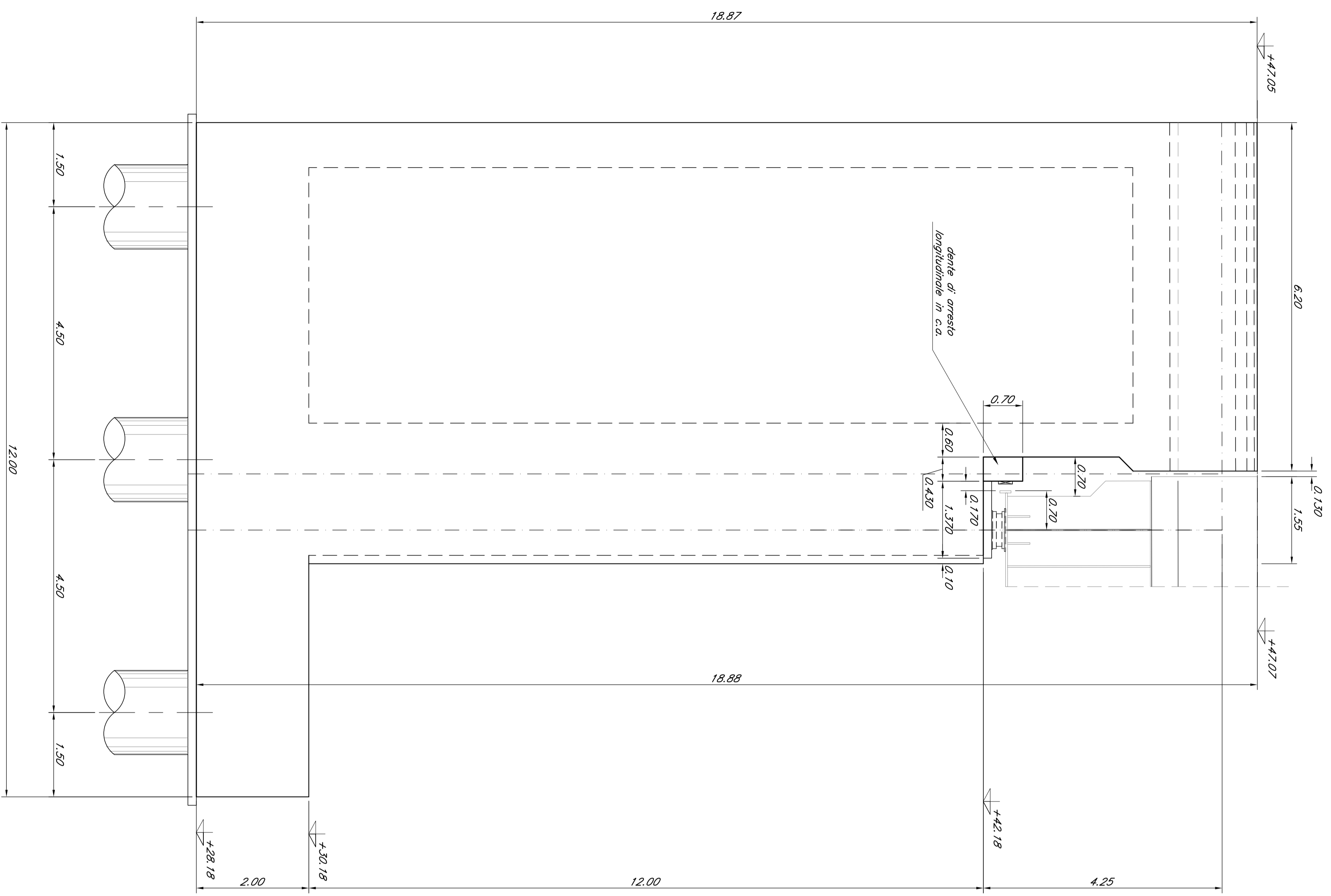
VISTA SUPERIORE E-E Scala 1:50
