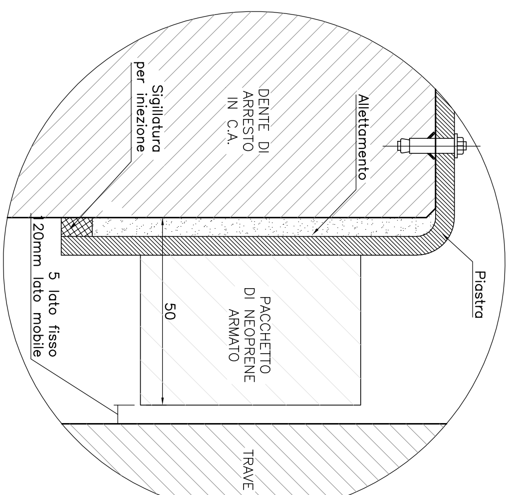
DETTAGLIO RITEGNO LONGITUDINALE
