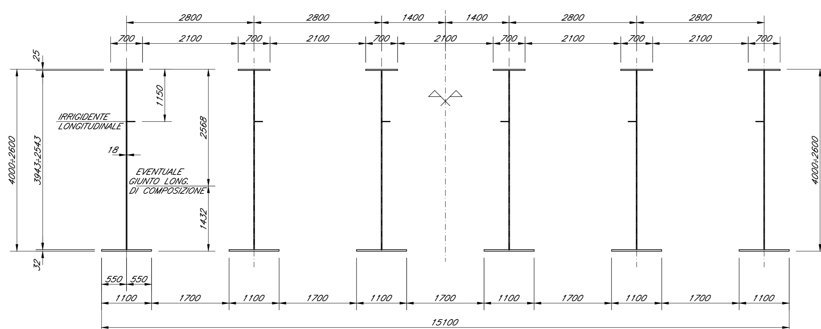
SEZIONE TIPICA TRAVI CONCIO C1 Scala 1:25
