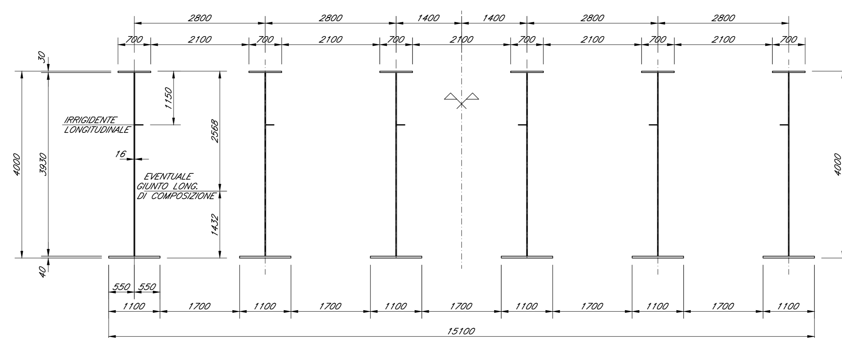
SEZIONE TIPICA TRAVI CONCIO C2 Scala 1:25
