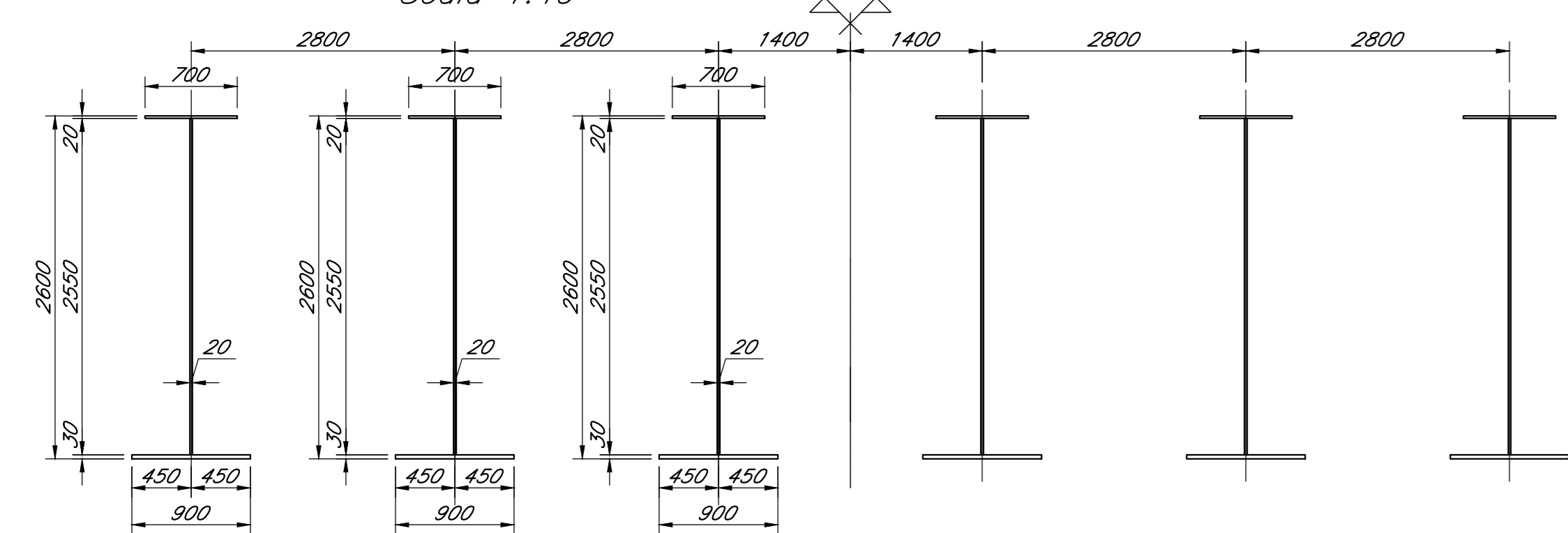
SEZIONE TIPICA TRAVI CONCIO C1 Scala 1:40
