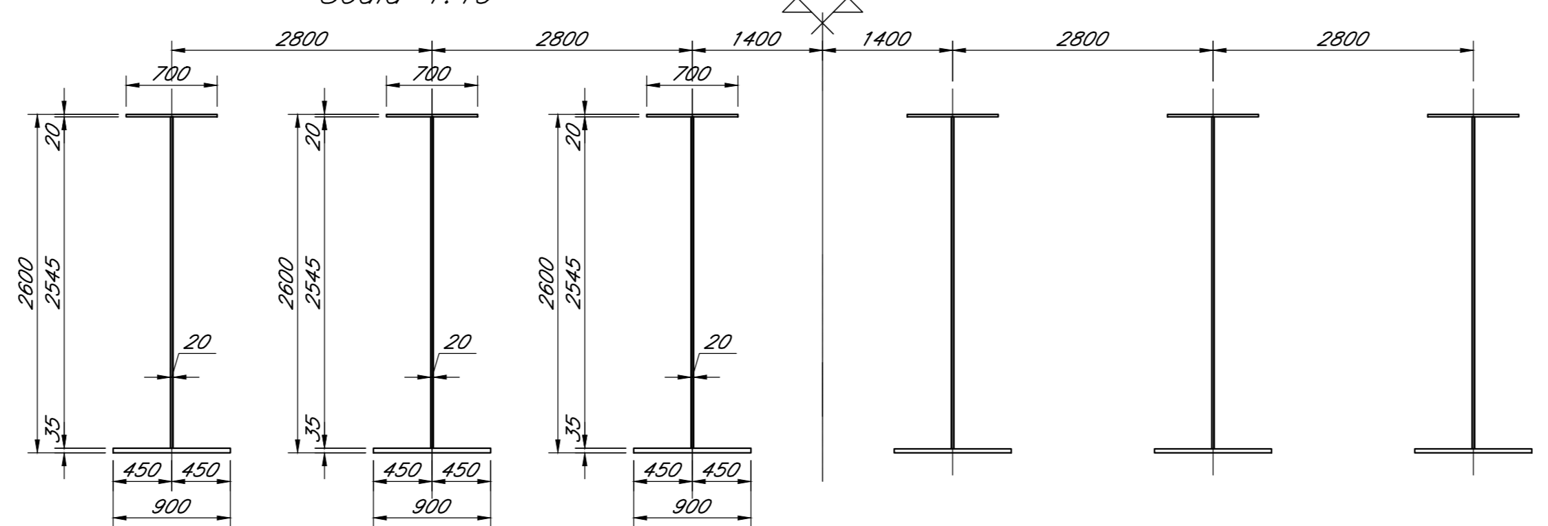
SEZIONE TIPICA TRAVI CONCIO C2 Scala 1:40
