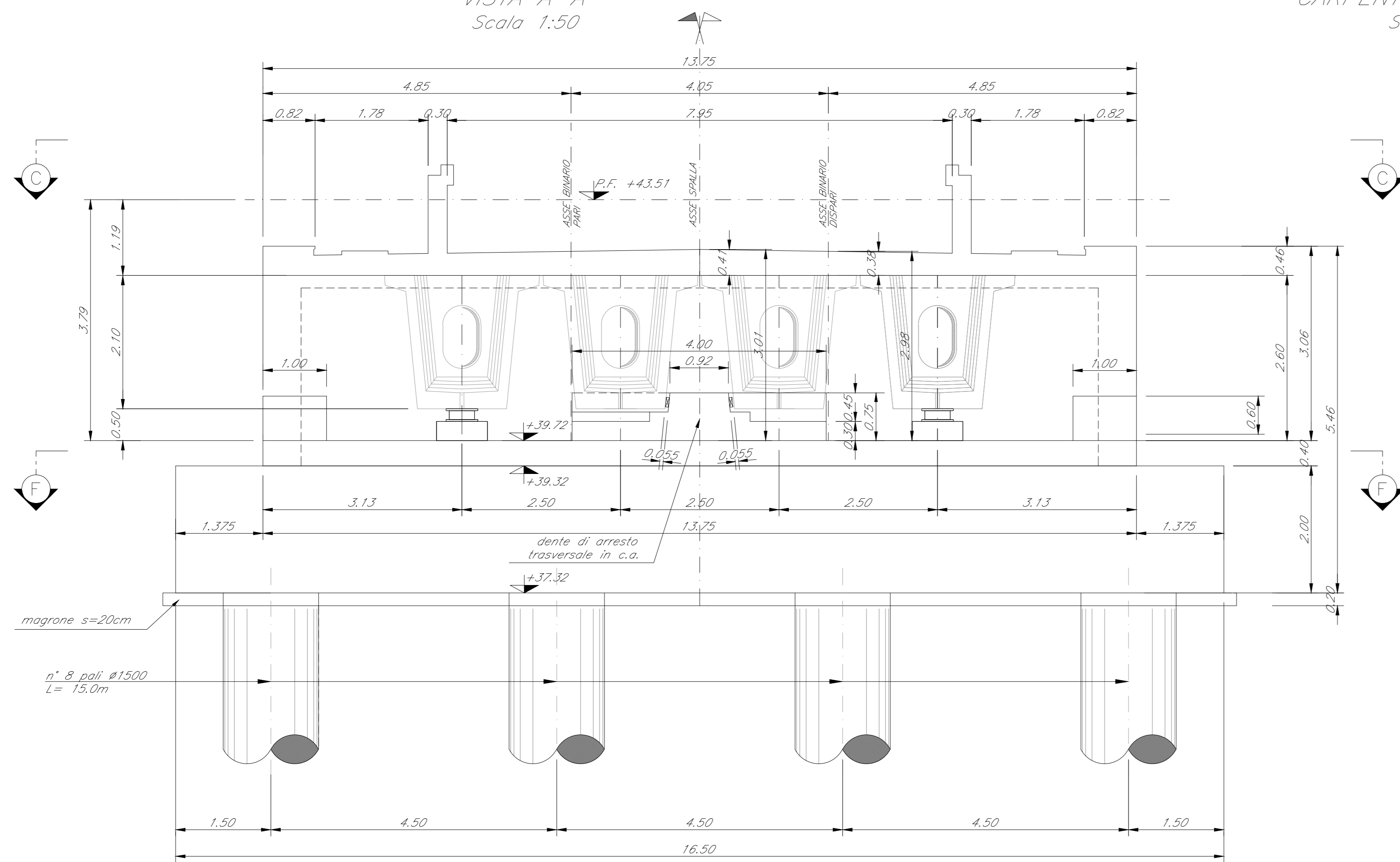
VISTA A-A Scala 1:50
