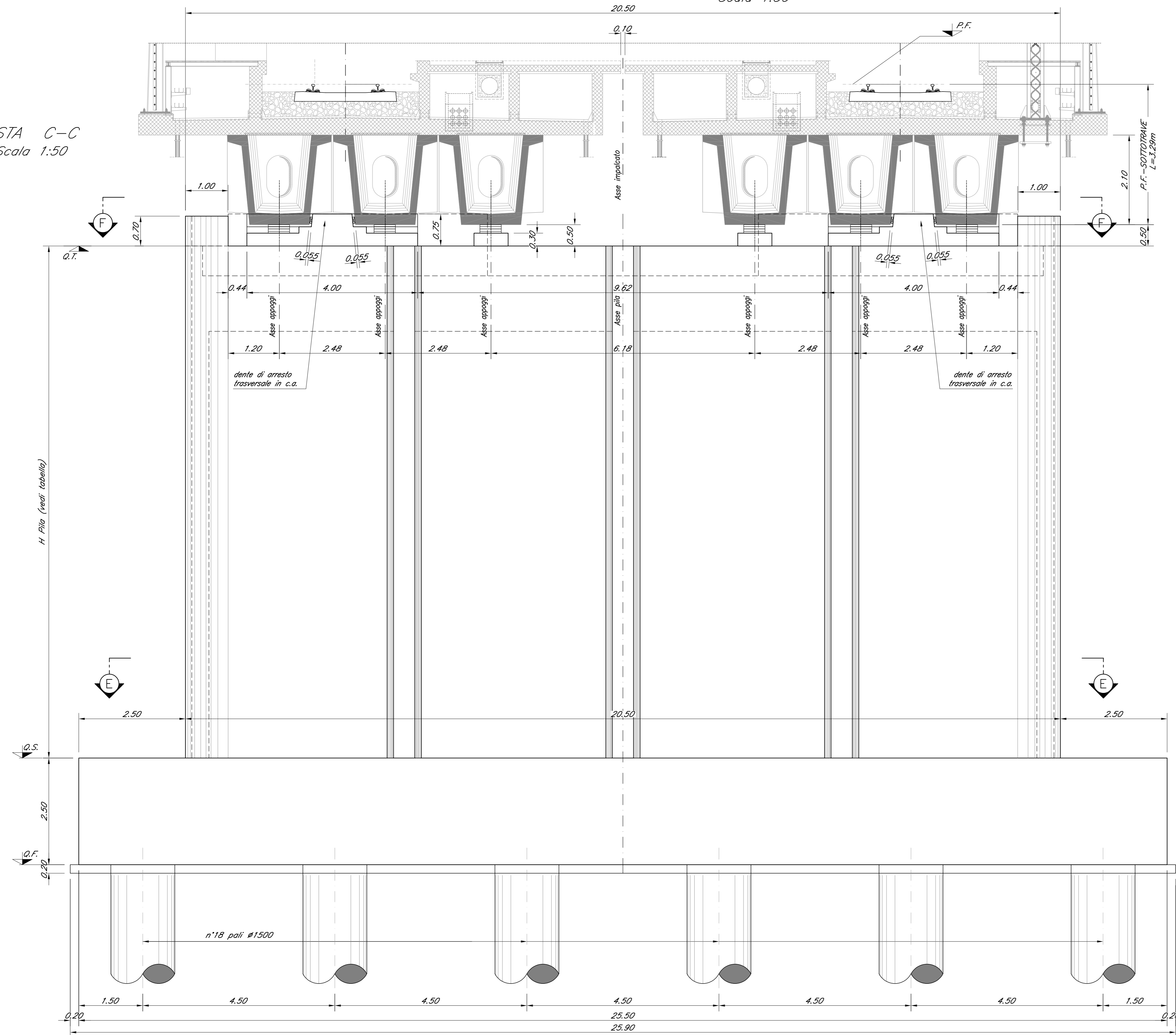
VISTA C-C Scala 1:50
