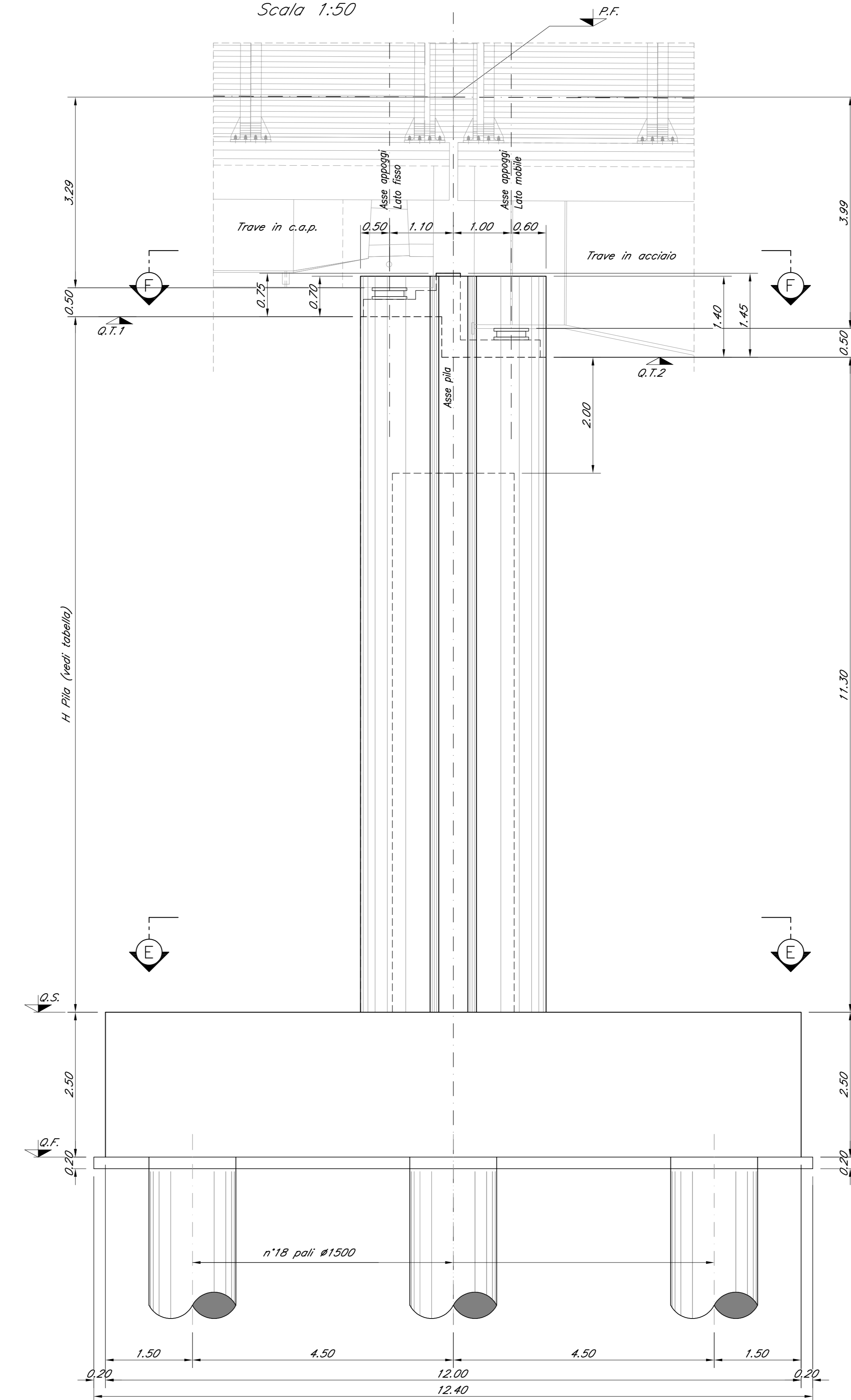
VISTA D-D Scala 1:50
