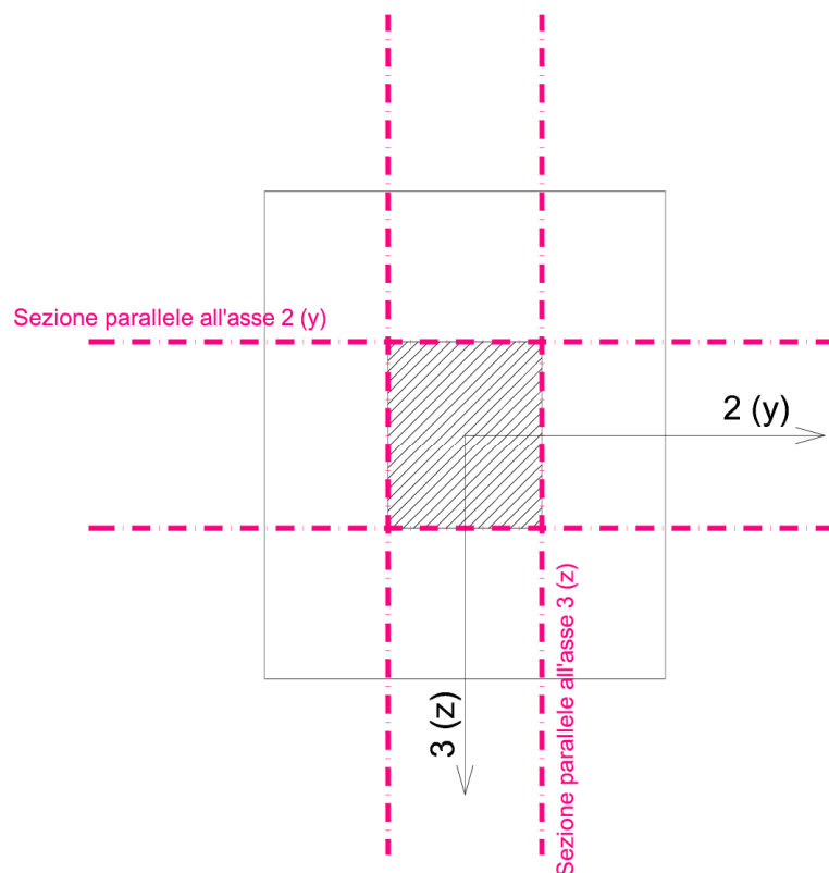
Figura 26: Sezioni in cui sono state determinate le sollecitazioni flessionali e di taglio.
