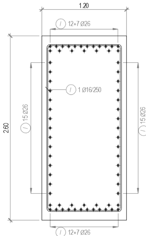
Figura 23: Armatura diaframmi.
