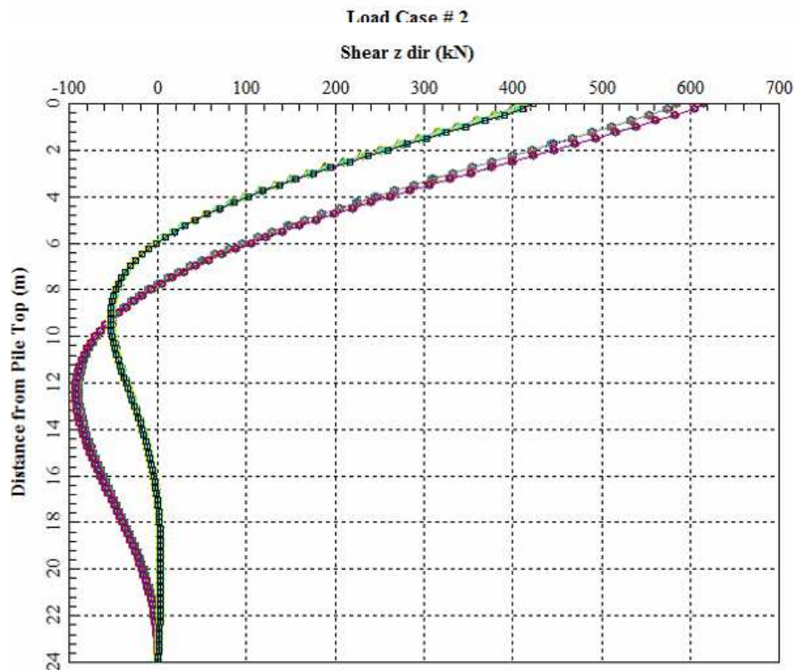
Figura 22: Combinazione sismica SLV: Andamento con la profondità del taglio.
