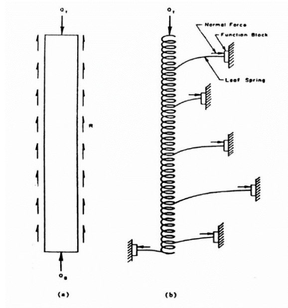
Figura 7: Meccanismo di trasferimento del carico assiale
