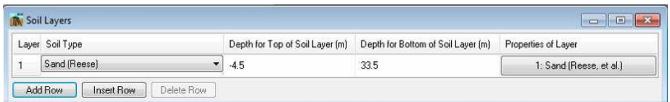
Figura 14: Stratigrafia modello GROUP-v2016.
