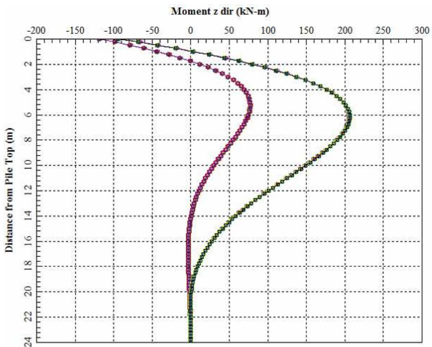
Figura 19: Combinazione statica SLU: Andamento con la profondità del momento.
