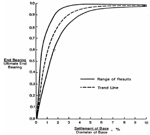
Figura 9: Argille. Curva di trasferimento base
