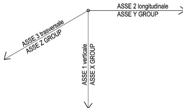
Figura 1. Figura 2: Sistema di riferimento per le azioni ad intradosso plinto.
