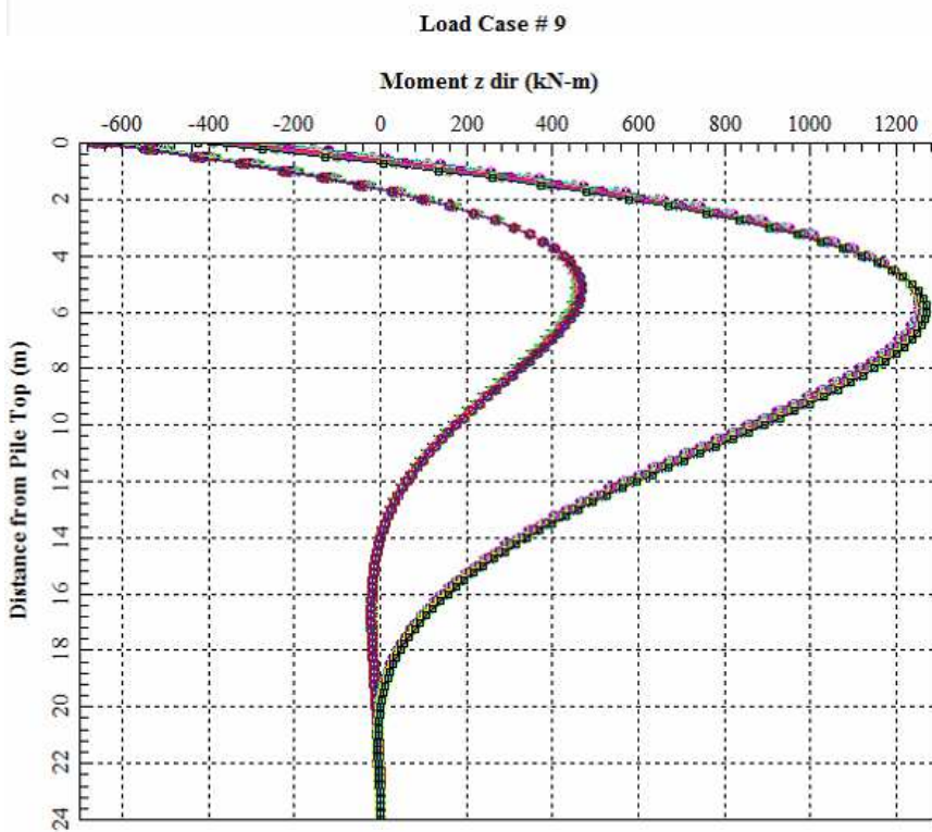
Figura 21: Combinazione sismica SLV: Andamento con la profondità del momento
