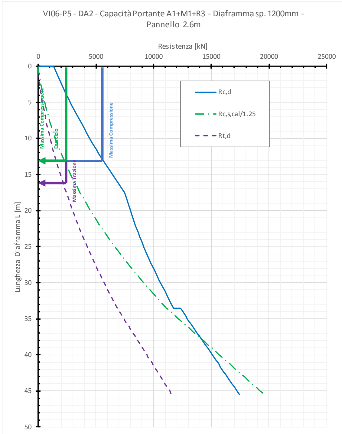
Figura 24: Capacità portante del diaframma singolo
