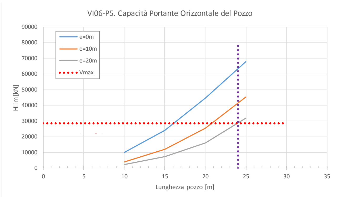
Figura 25: Diagrammi di capacità portante orizzontale del Pozzo.
