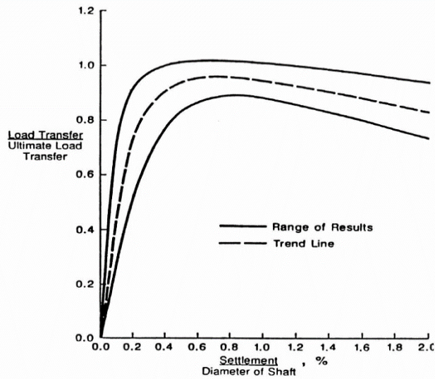
Figura 8: Argille. Curva di trasferimento laterale
