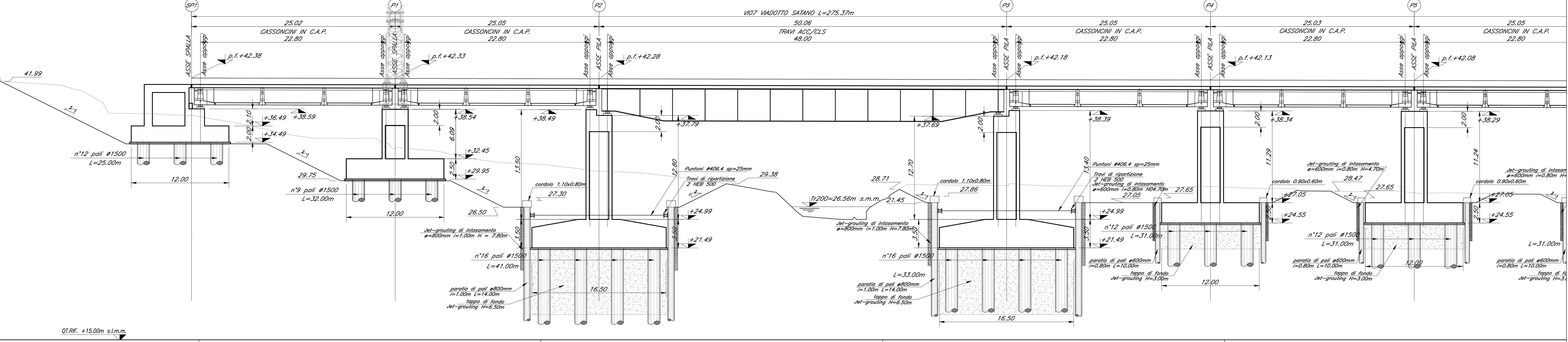
SEZIONE LONGITUDINALE BINARIO DISPARI Scala 1:200
