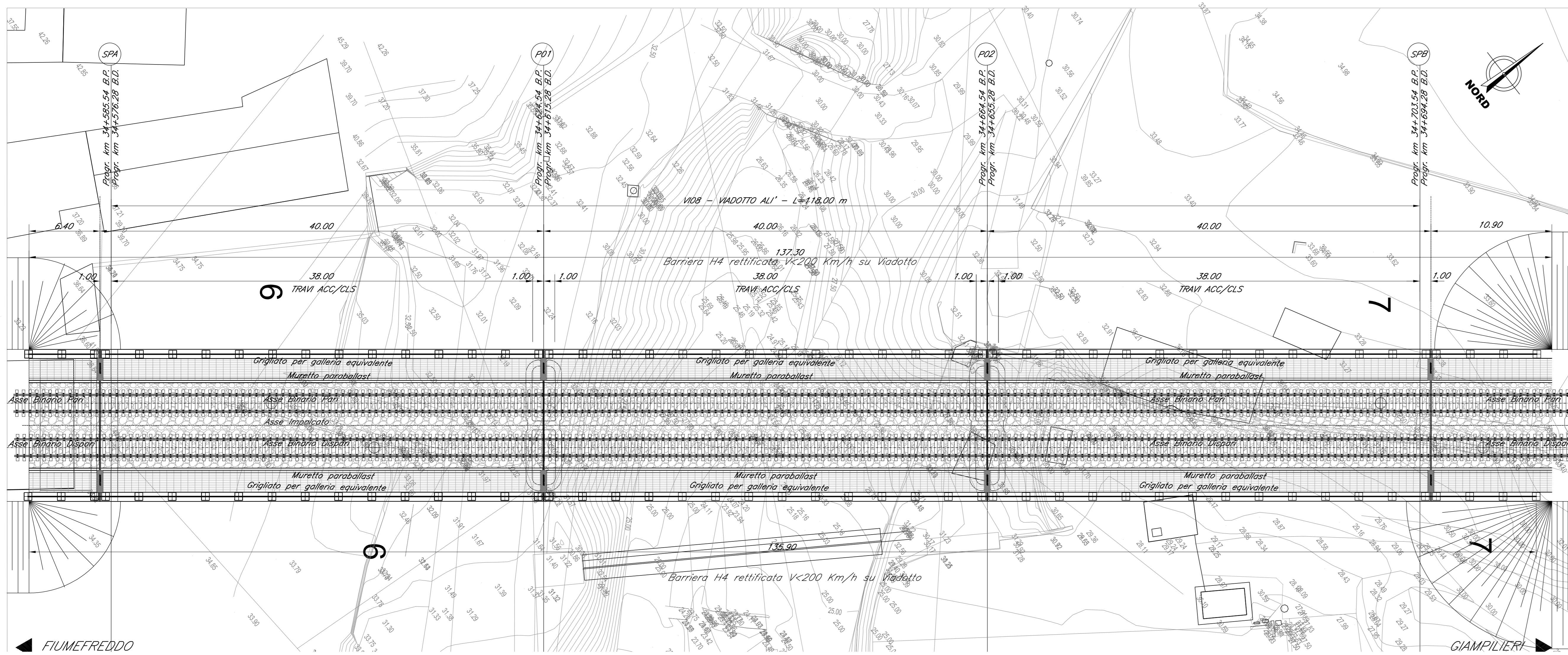
PIANTA IMPALCATO Scala 1:200
