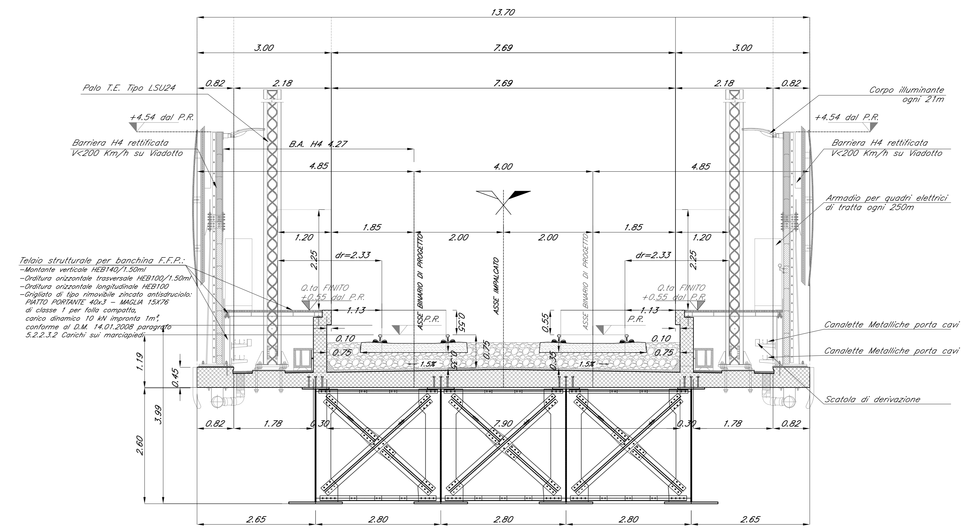
SEZIONE TIPO Scala 1:50
