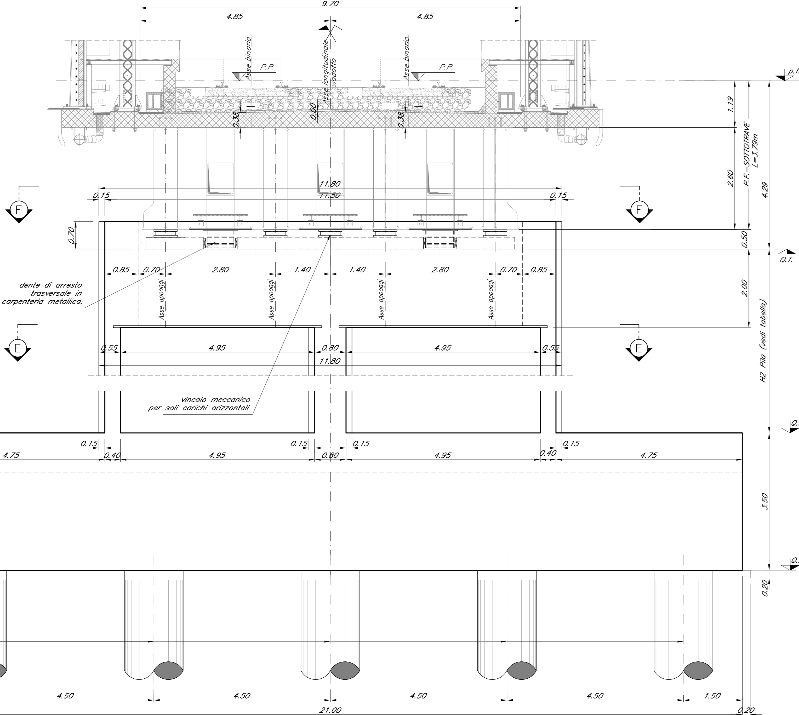
SEZIONE B-B Scala 1:50
