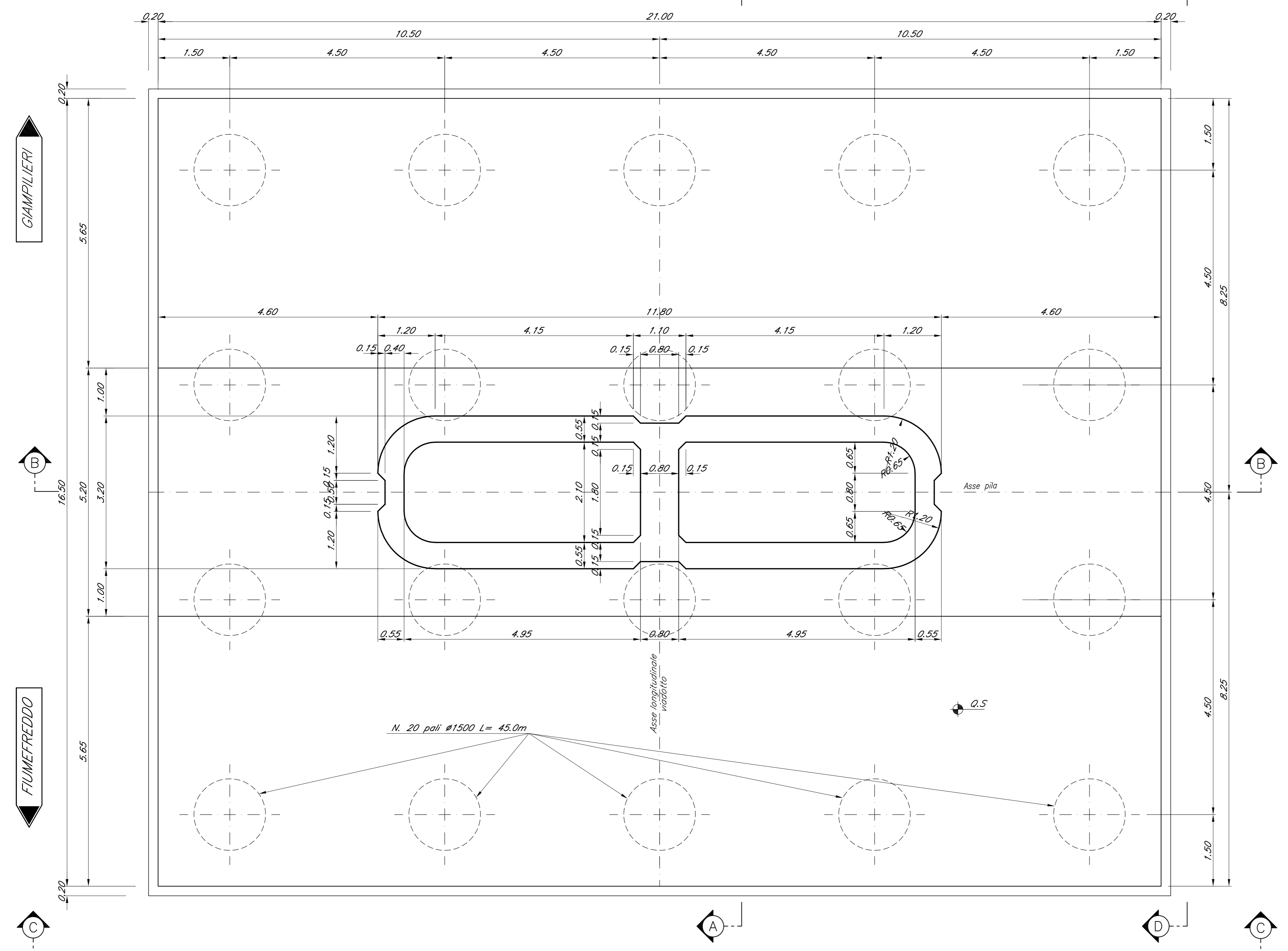
SEZIONE E-E Scala 1:50
