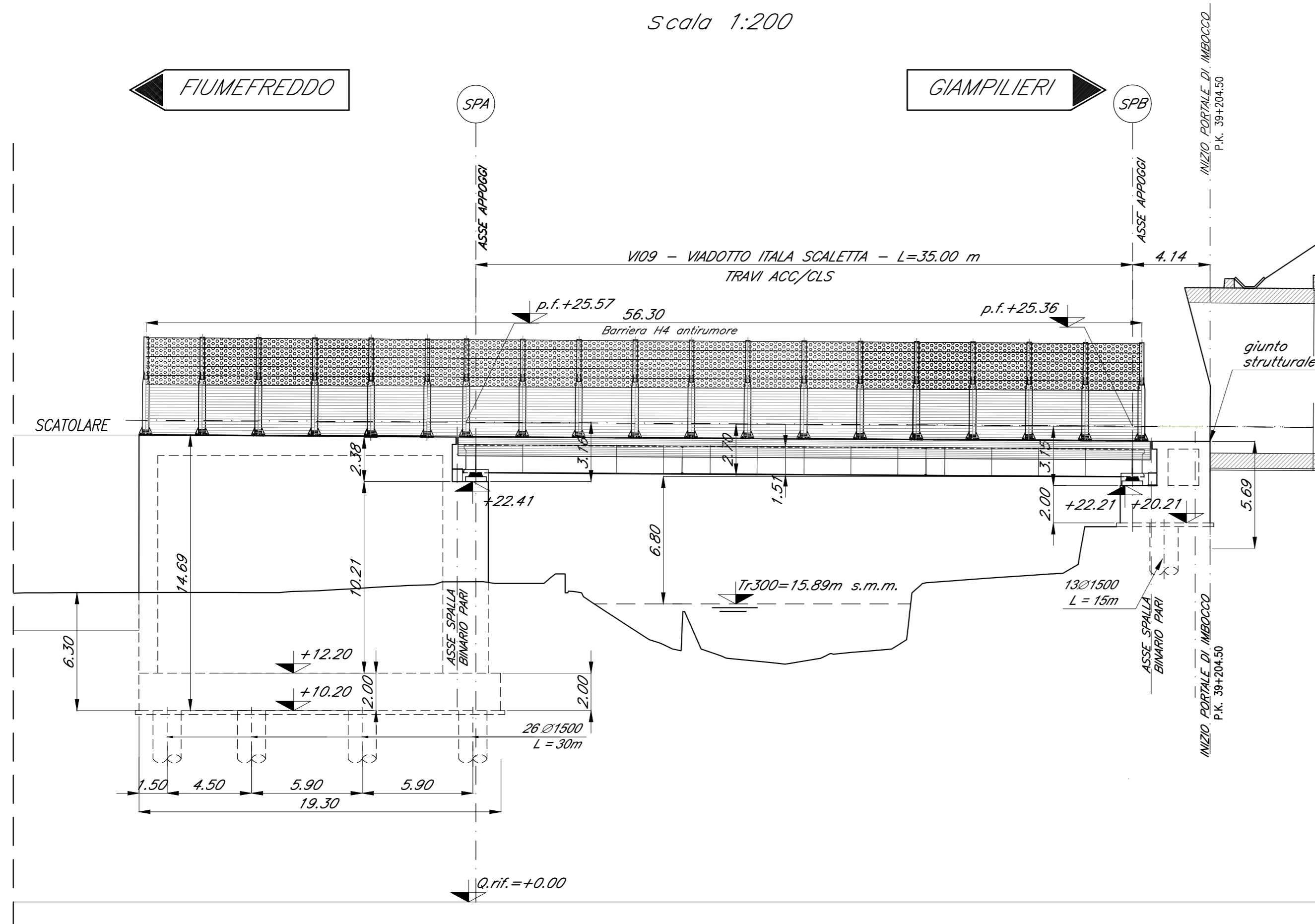
PROSPETTO BINARIO PARI Scala 1:200
