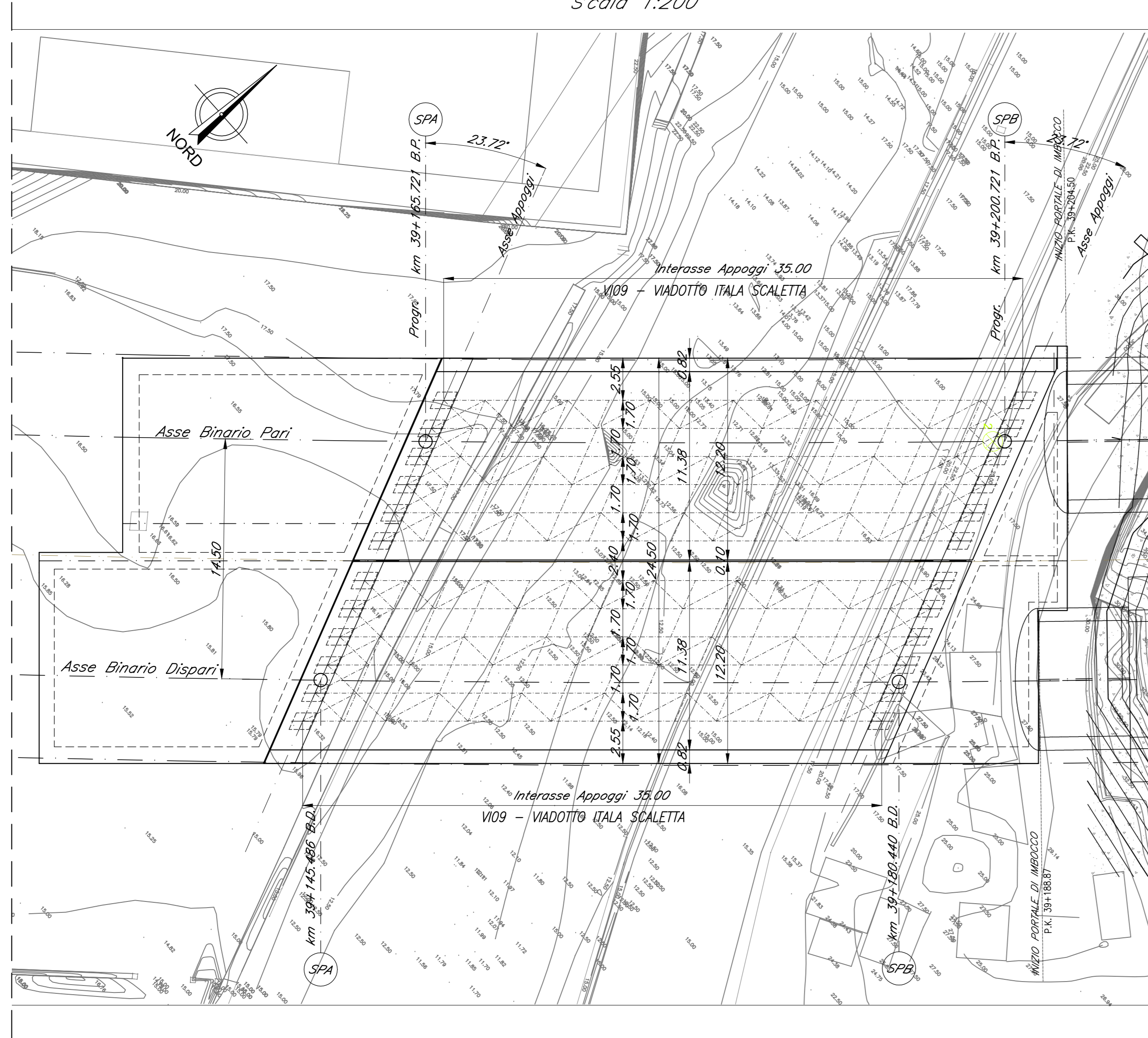
PIANTA TRAVI Scala 1:200
