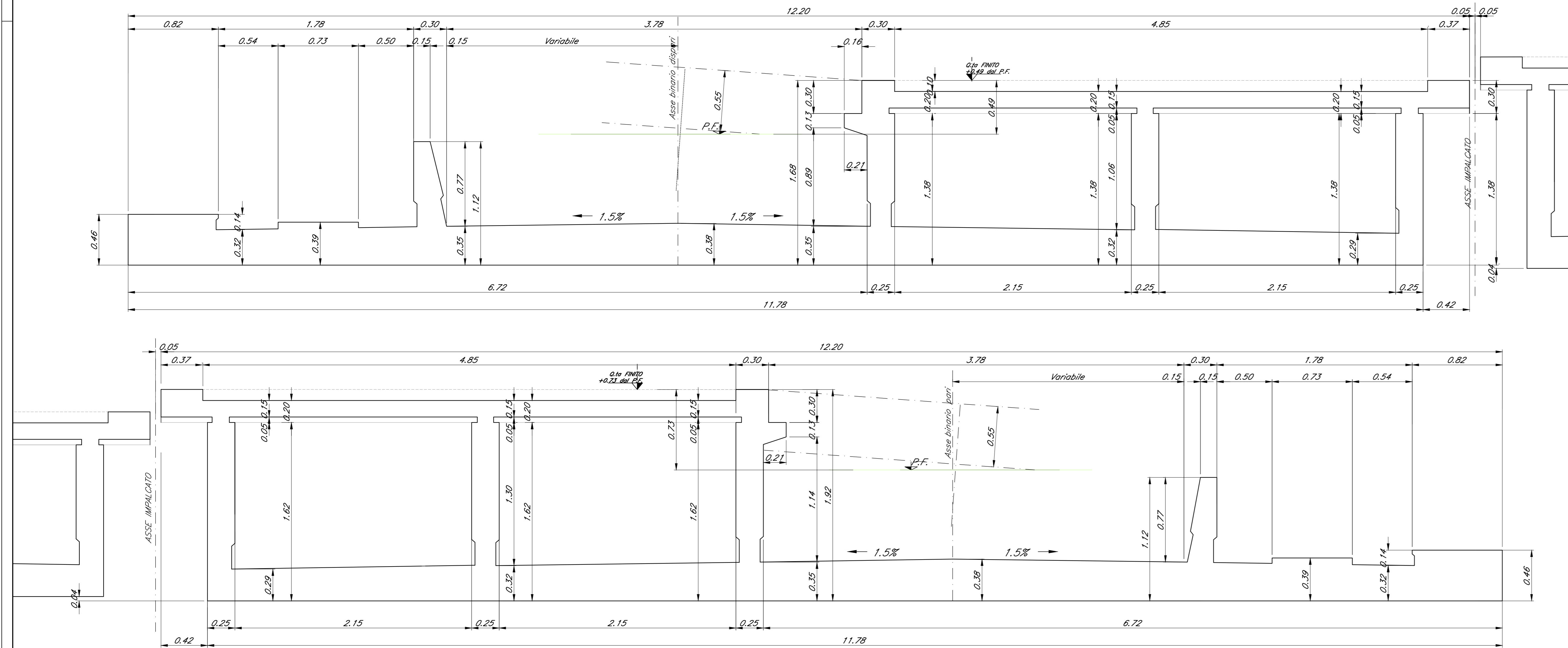
DETTAGLIO DEI MURETTI PARABALLAST IN ASSE APOGGIO Scala 1:20
