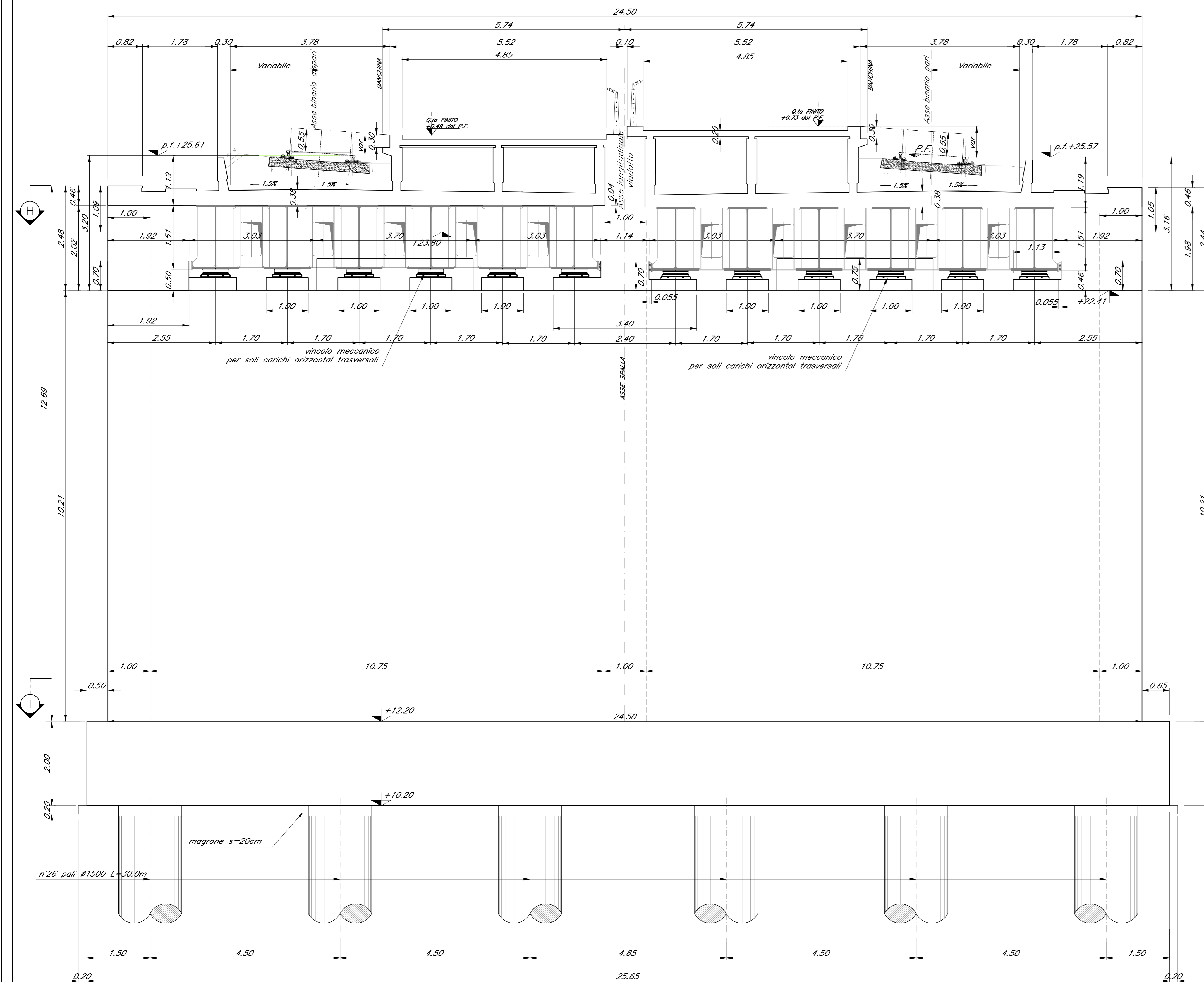
DETTAGLIO DEI MURETTI PARABALLAST IN ASSE APOGGIO Scala 1:20
