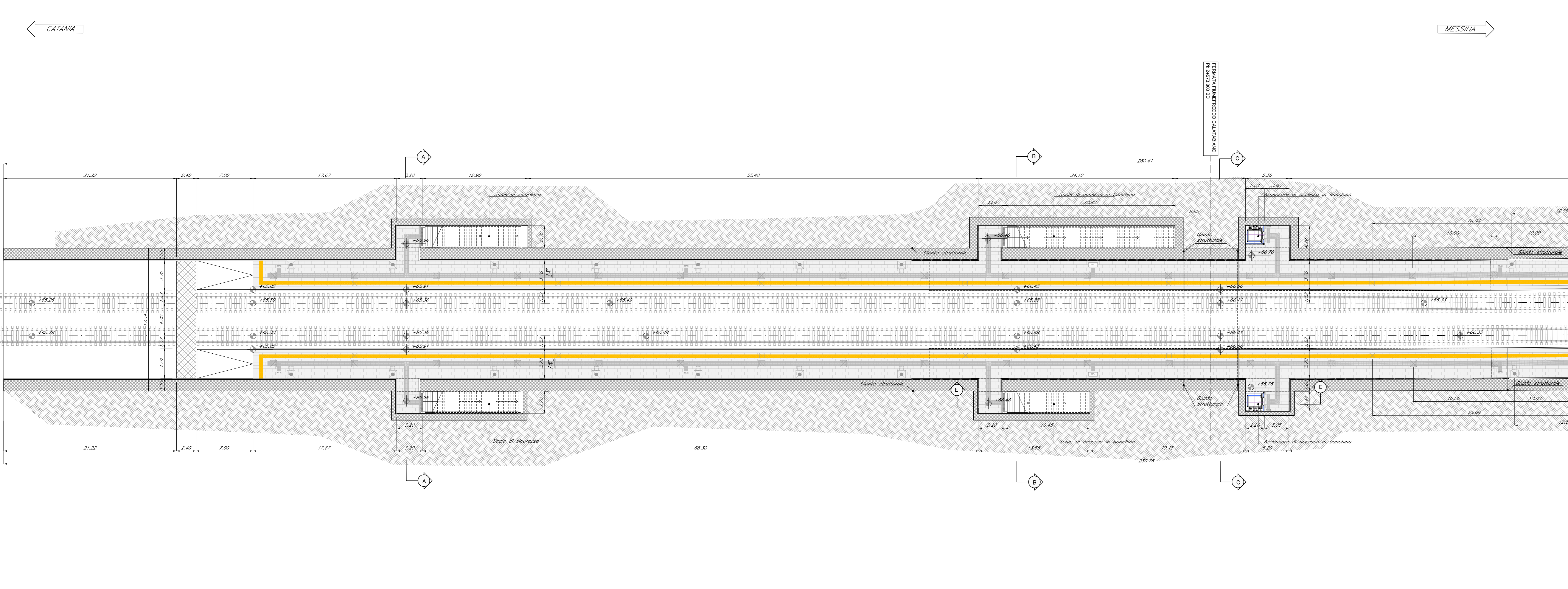
PIANTA QUOTA BANCHINA - stralcio 1 scala 1:200
