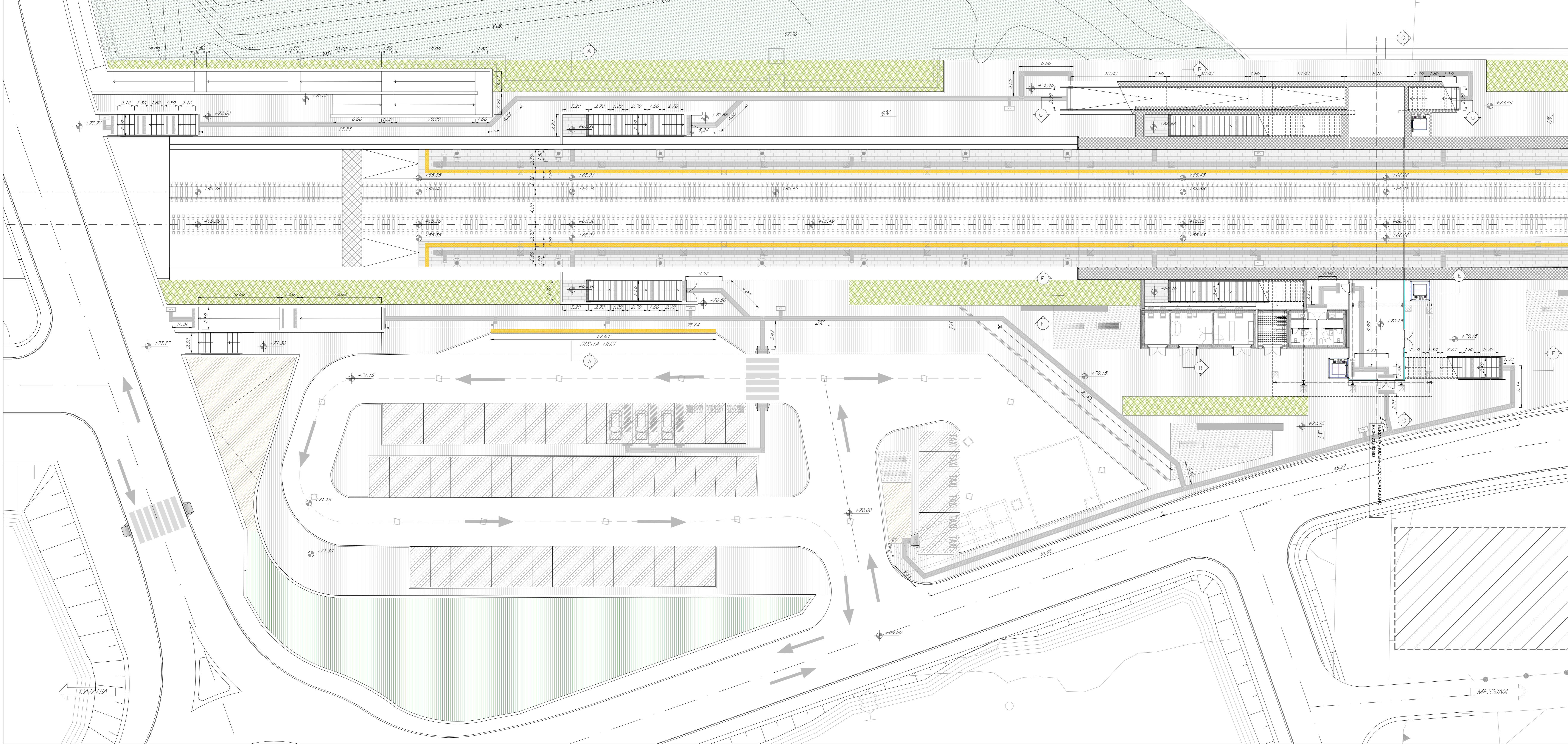
PIANTA FABBRICATO VIAGGIATORI - stralcio 1 scala 1:200
