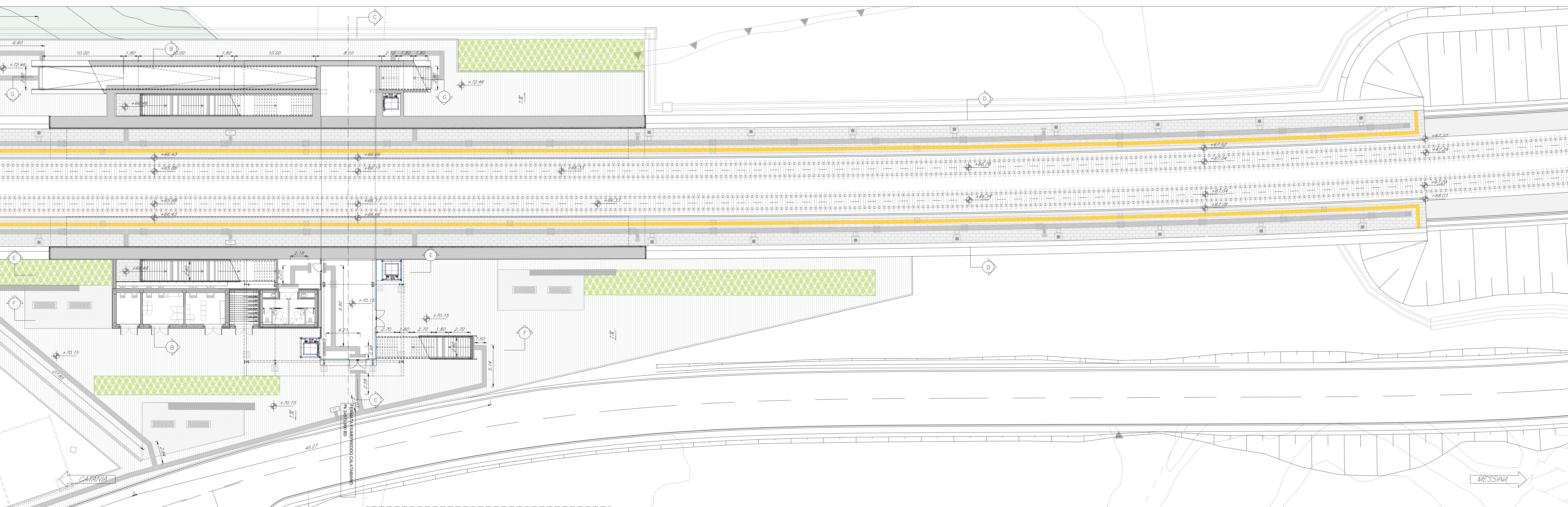
PIANTA FABBRICATO VIAGGIATORI - stralcio 2 scala 1:200
