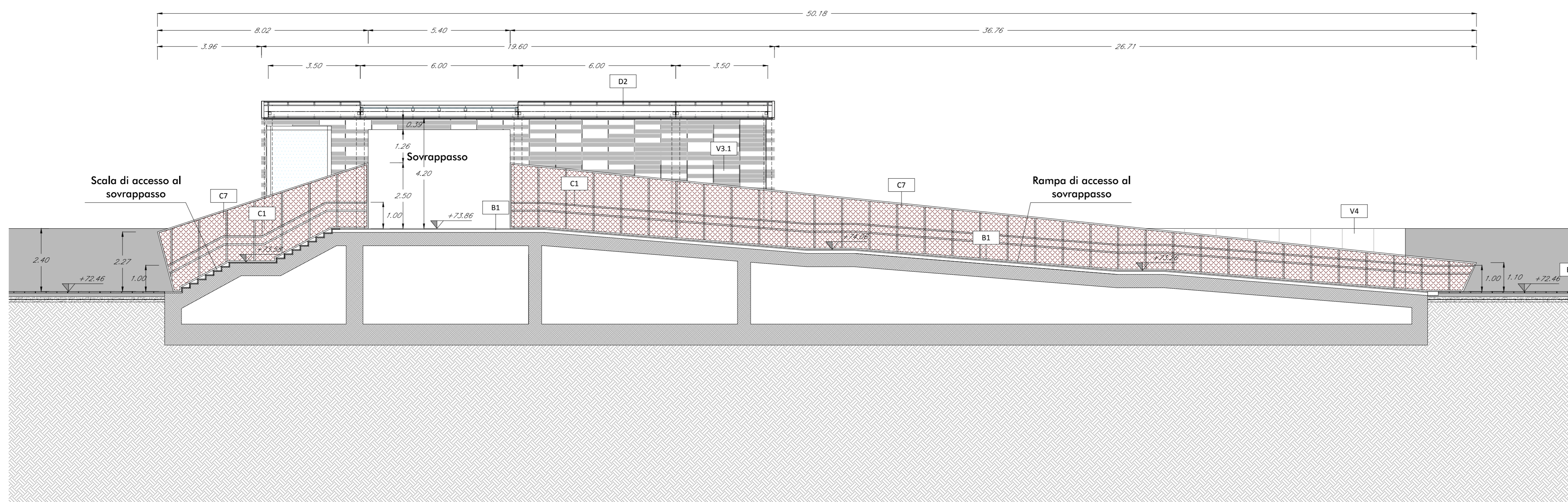
SEZIONE GG' scala 1:100
