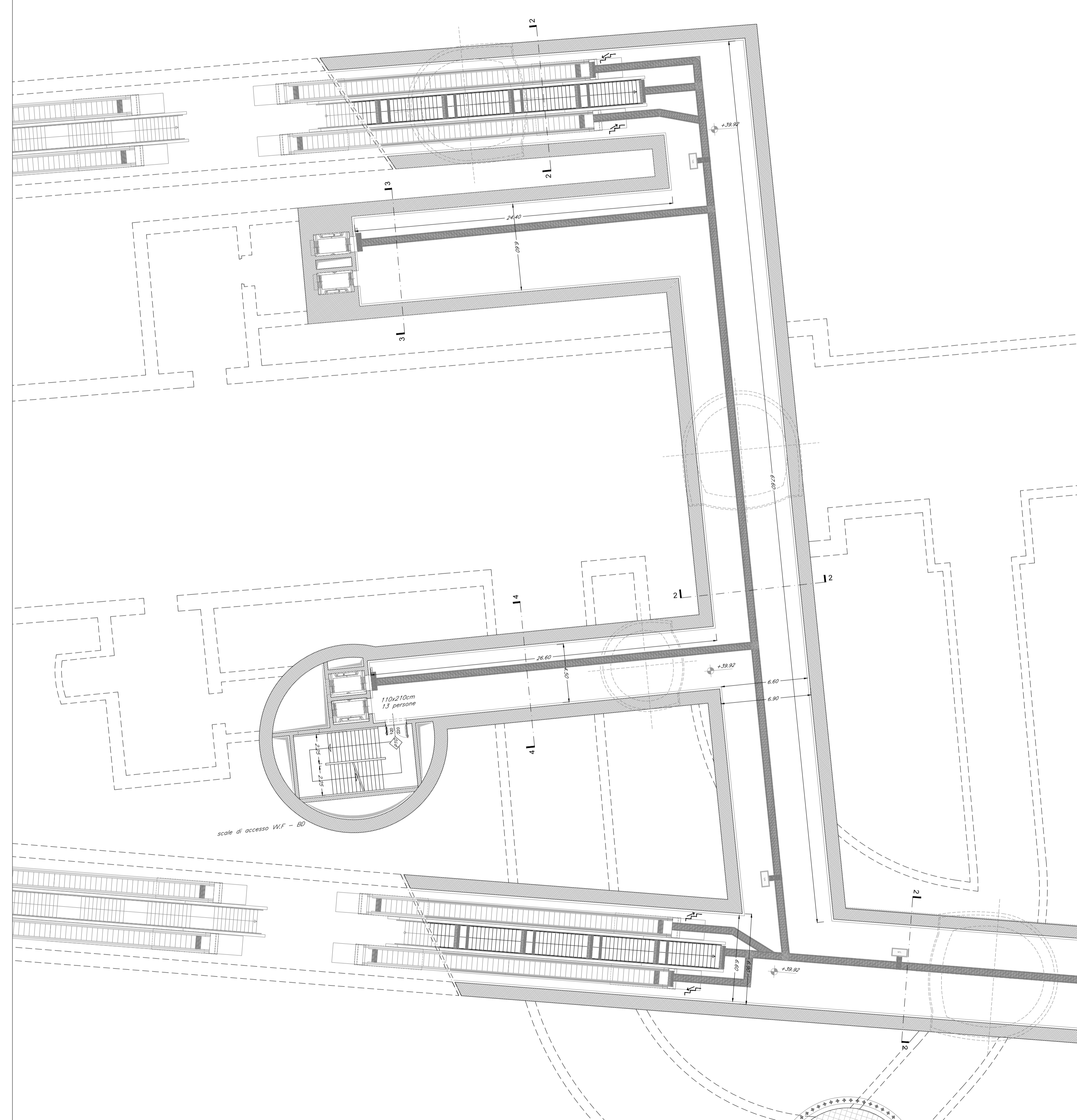
STRALCIO "1" - PIANTA QUOTA MEZZANINO - lato ME scala 1:200
