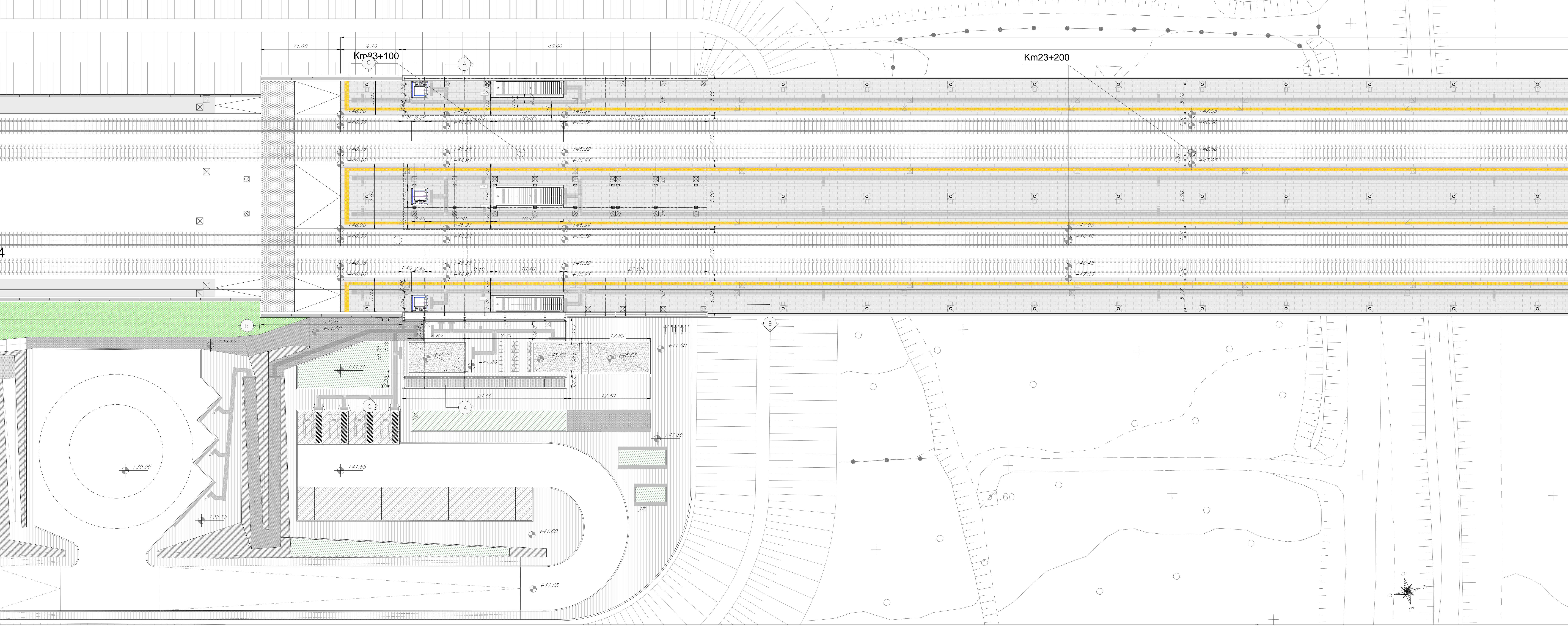
01 PIANTA QUOTA BANCHINA - stralcio 1 scala 1:200
