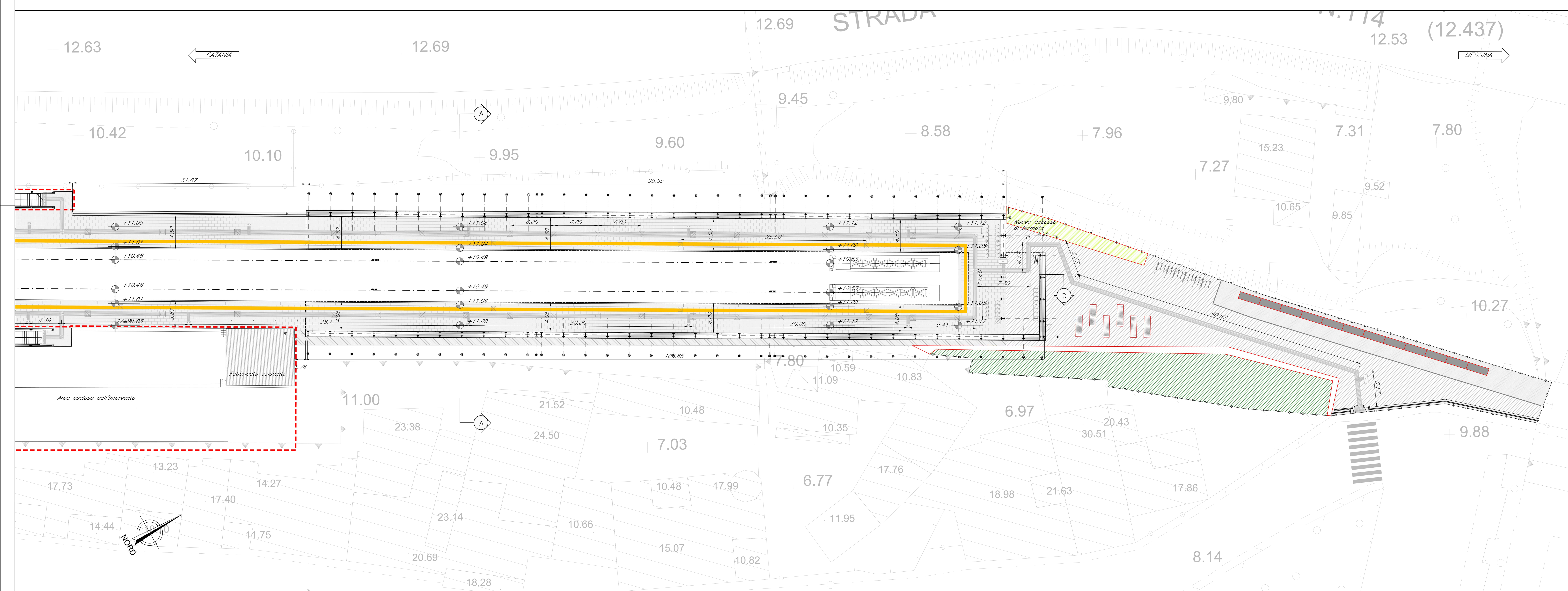
PIANTA QUOTA BANCHINA stralcio B scala 1:200
