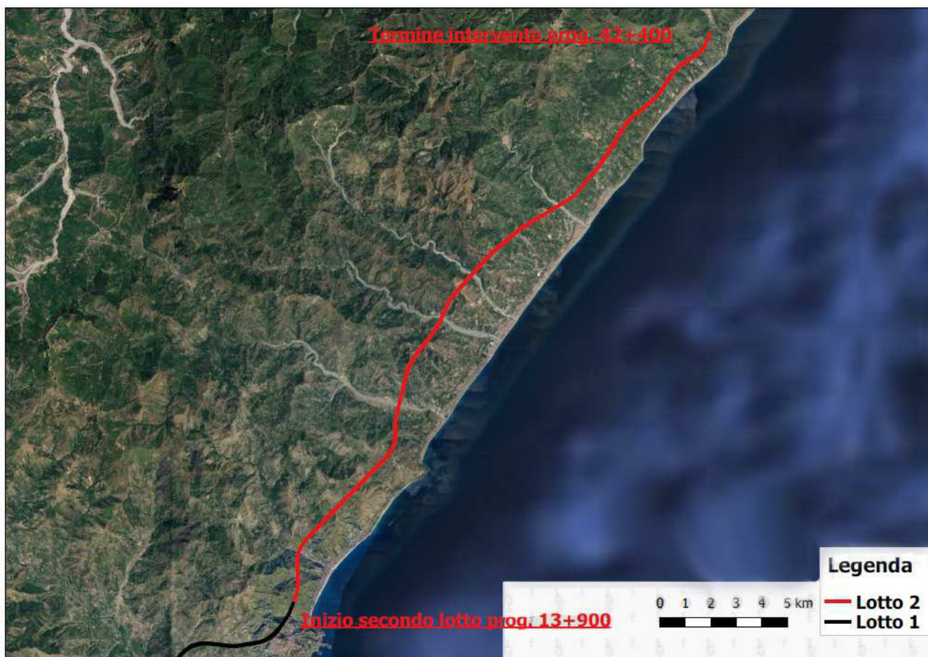
Figura 2-1 - Inserimento del progetto su foto aerea. Il Lotto 2 è evidenziato in rosso.
