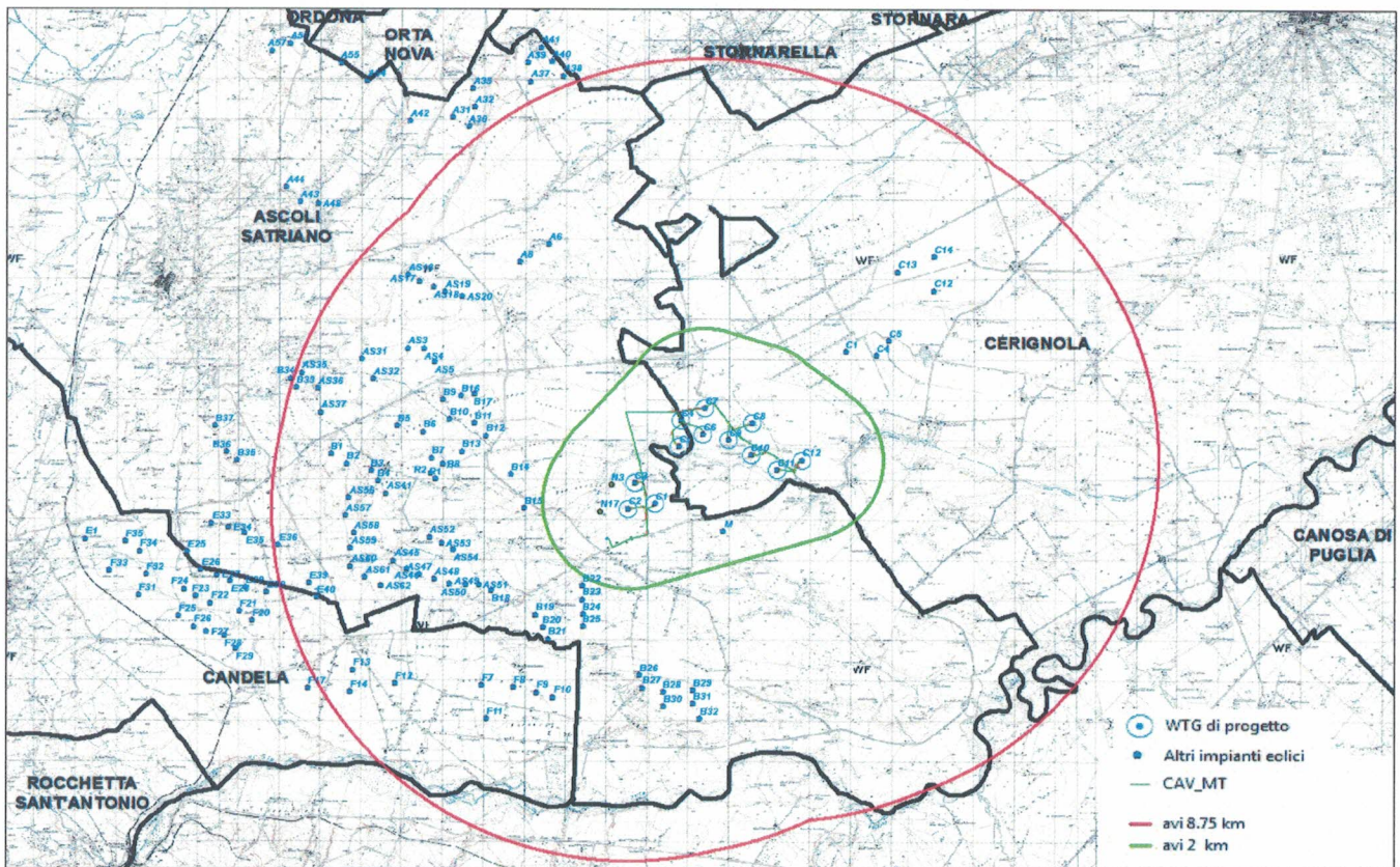
FIG. 20 - Planimetria degli impianti eolici nella AVI (8,75 km dal sito proposto) su cartografia IGM.
