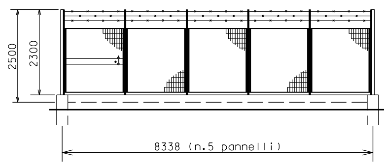
PROSPETTO A
