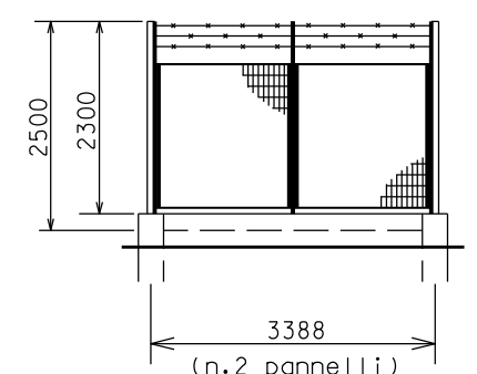
PROSPETTO B
