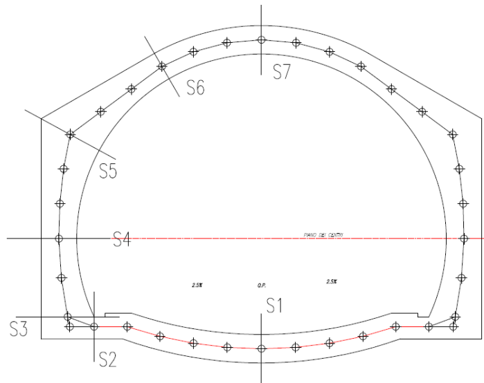
Sezioni di verifica per la galleria artificiale
