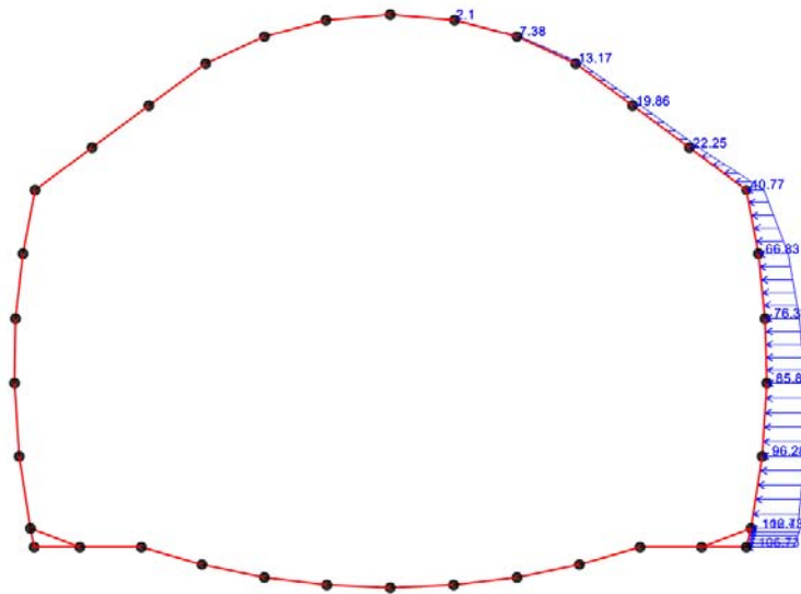
Spinta a riposo in destra
