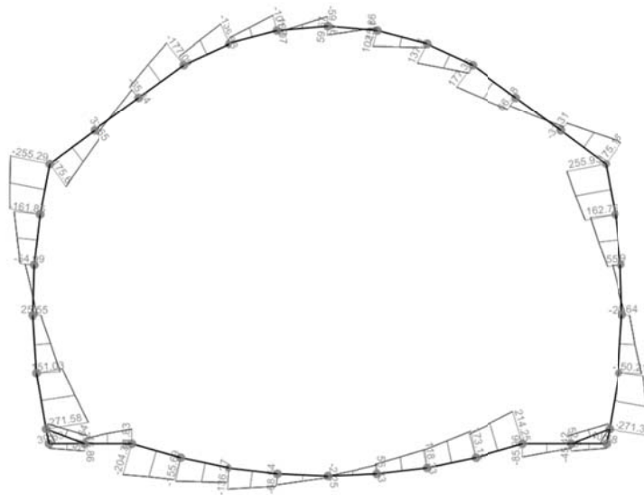
Diagramma dello sforzo flettente per la combinazione involuppo
