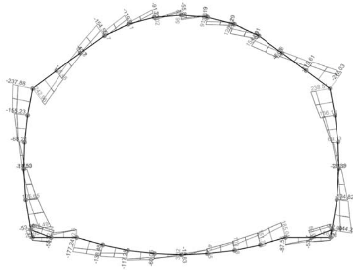
Diagramma dello sforzo flettente per la combinazione inviluppo
