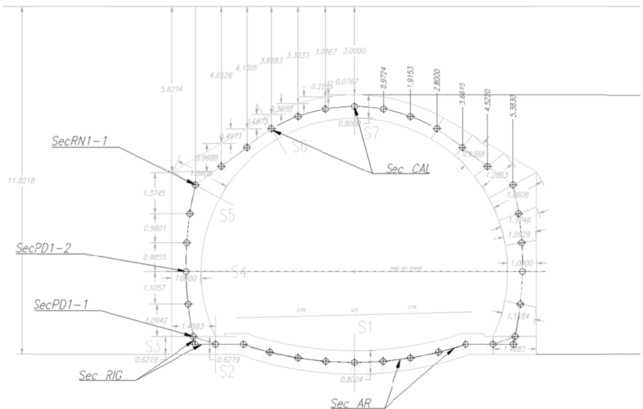
Modello di calcolo adottato per le analisi
