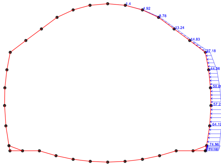
Spinta attiva in sinistra
