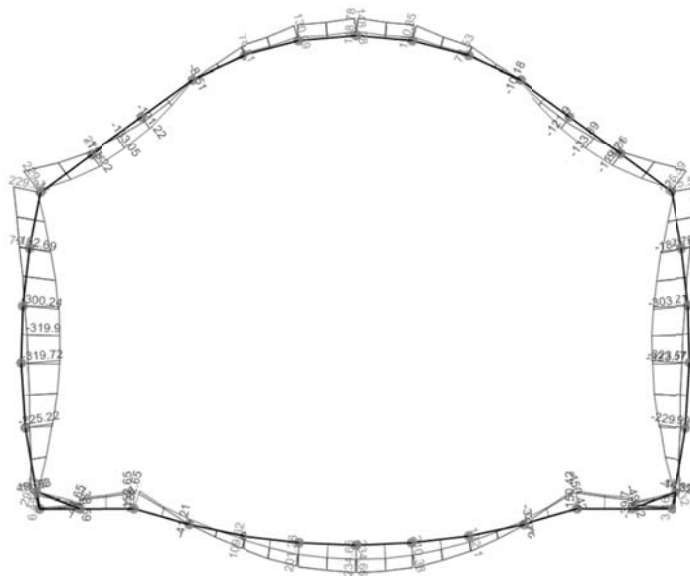
Diagramma dello sforzo flettente per la combinazione involuppo
