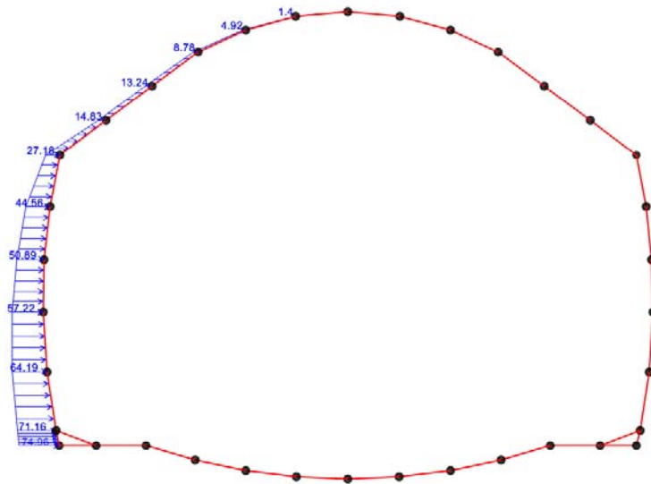
Spinta attiva in sinistra
