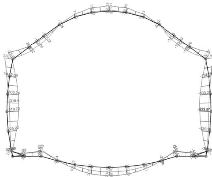
SLE –Frequente (SLE_FR_ENVE)
