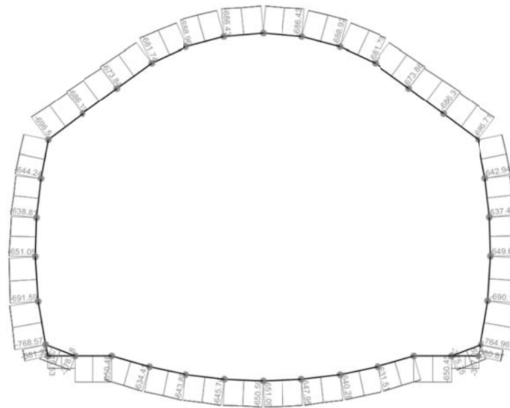
Diagramma dello sforzo di taglio per la combinazione involuppo
