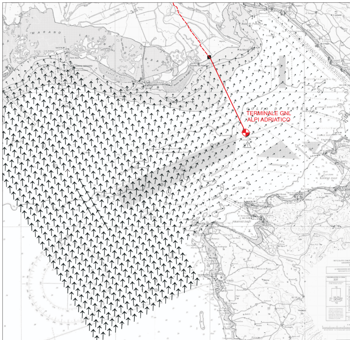
RISULTATO DELLA SIMULAZIONE DELLA PROPAGAZIONE DEL MOTO ONDOSO ALL'INTERNO DEL GOLFO. ONDA CON PERIODO DI RITORNO 100 ANNI E DIREZIONE DI PROVENIENZA 180°N.
