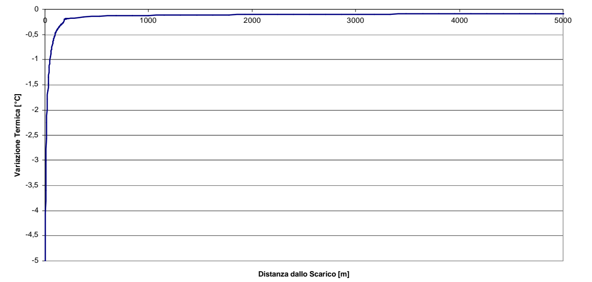
ANDAMENTO DEL GRADIENTE TERMICO IN RELAZIONE ALLA DISTANZA
