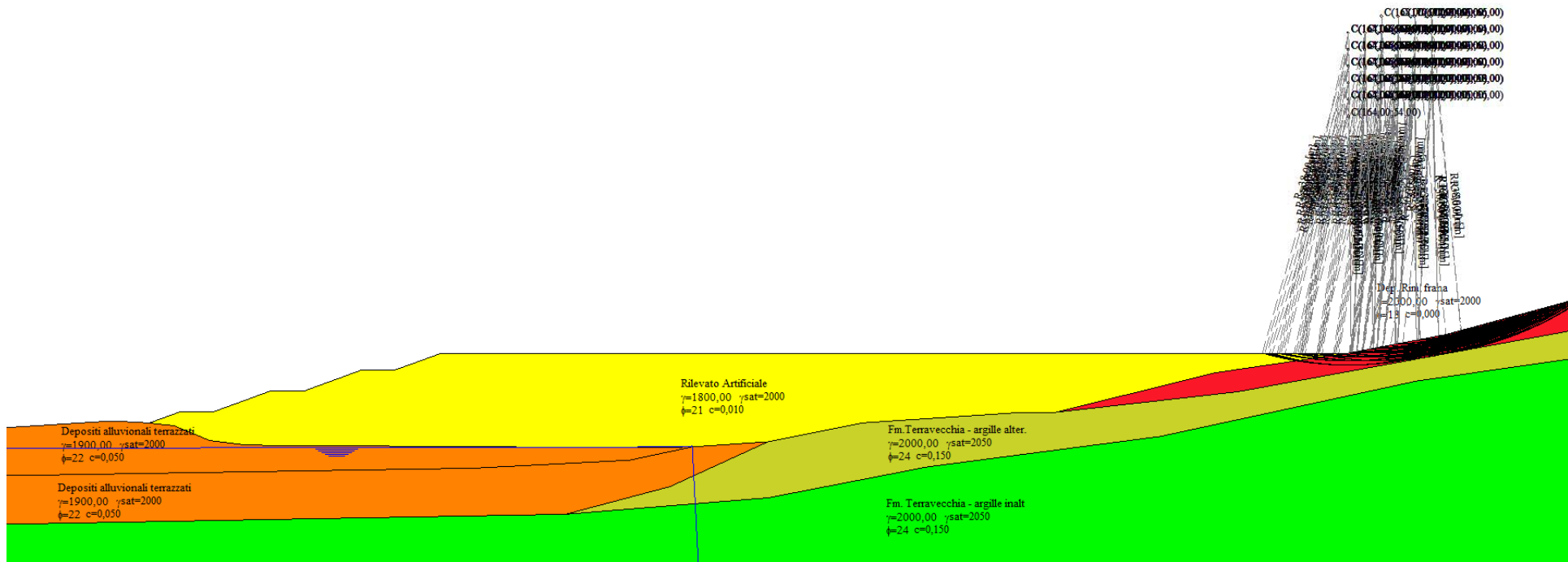
Superfici di scivolamento con F < 1,1
