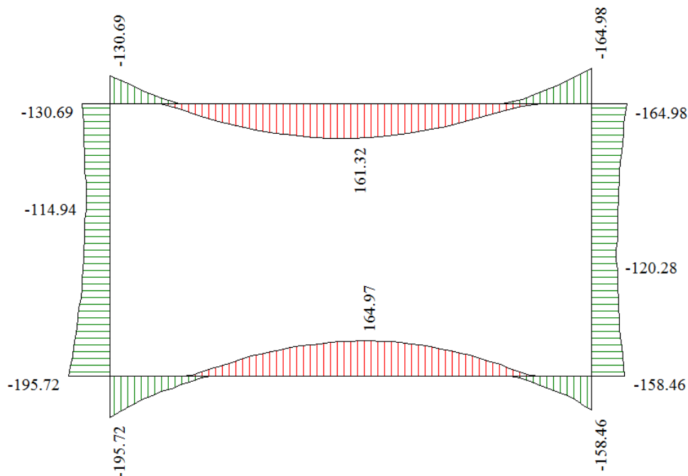
Involuppo diagrammi del momento flettente – SLE
