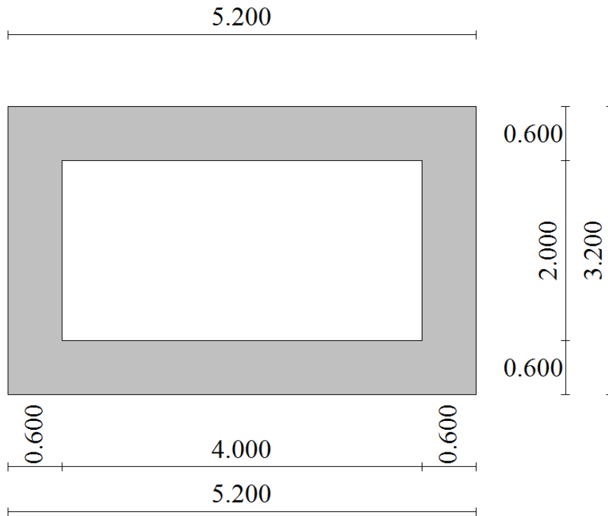
Modello Geometrico Geotecnico di Riferimento – 2/2
