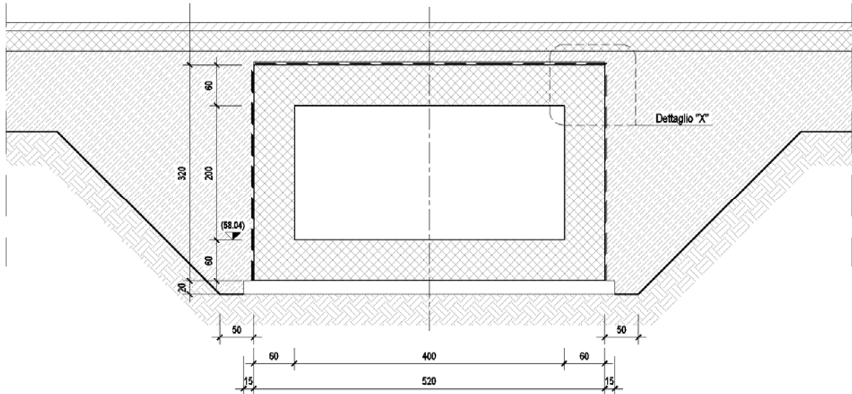
Figura 1 – Sezione trasversale
