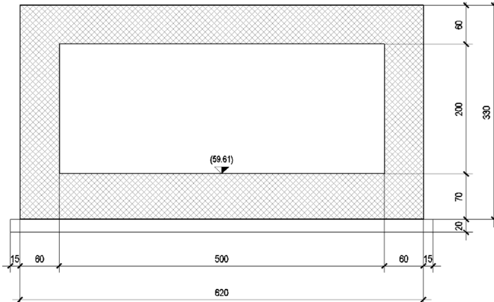
Figura 1 – Sezione trasversale
