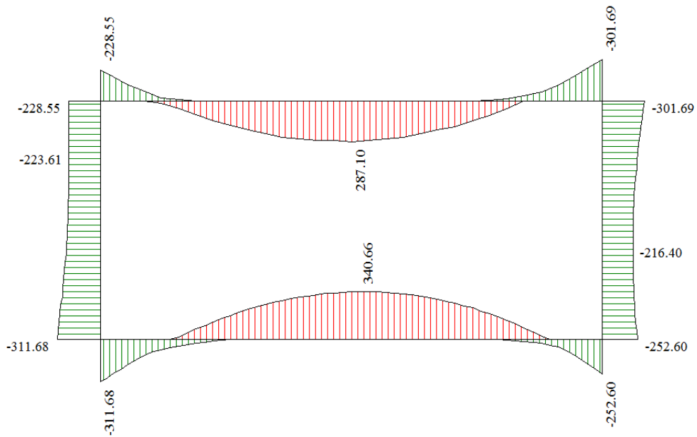
Involuppo diagrammi del momento flettente – SLU statico e sismico
