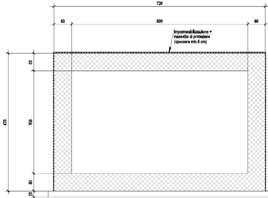
Figura 1 – Sezione trasversale
