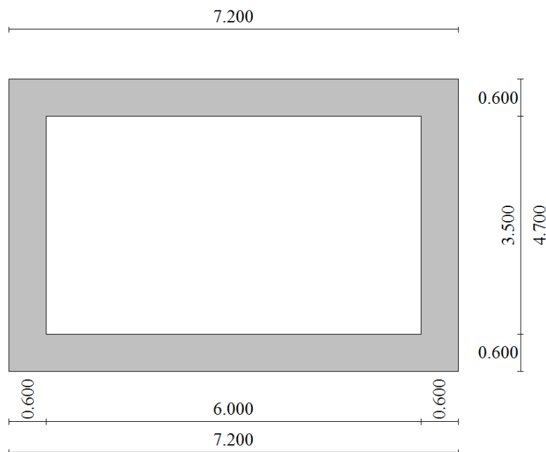
Modello Geometrico Geotecnico di Riferimento – 2/2
