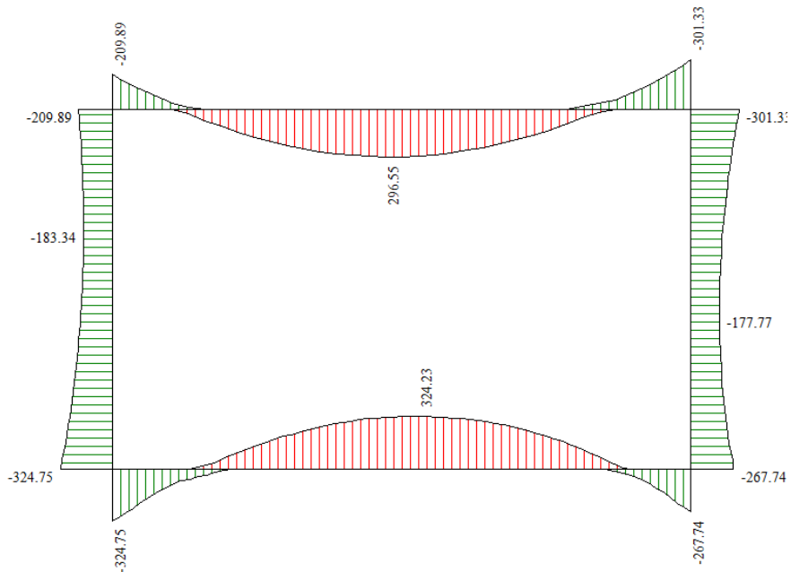
Involuppo diagrammi del momento flettente – SLE
