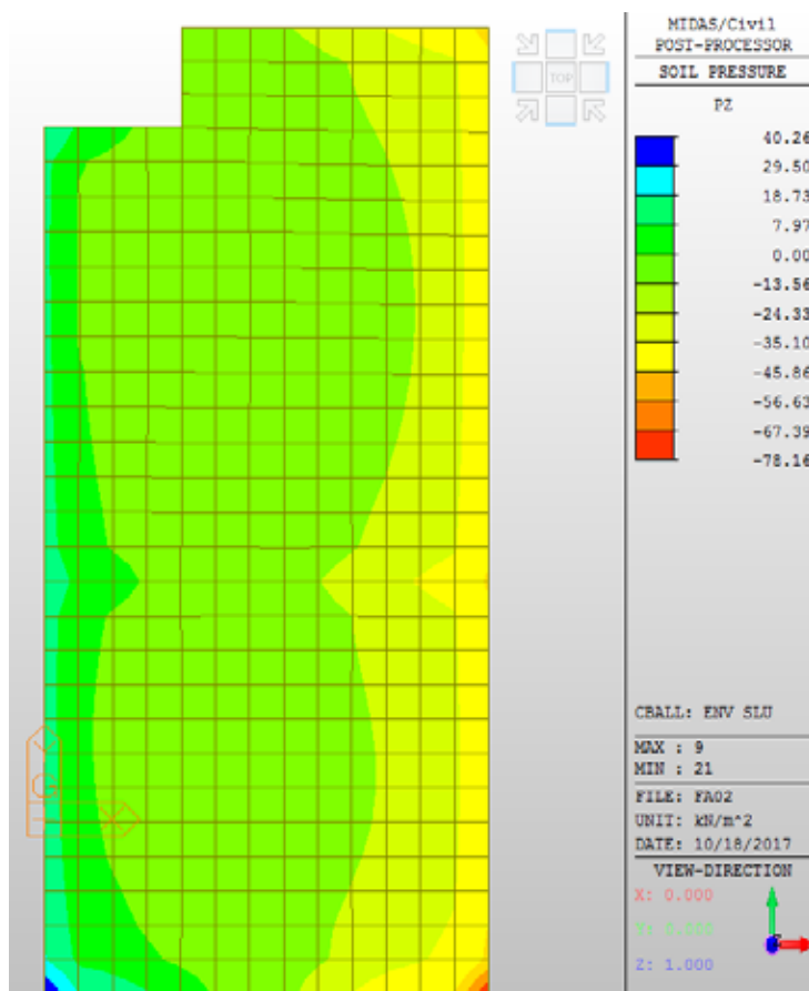
Figura 19 – Myy: Pressioni terreno
