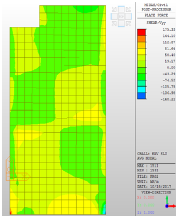
Figura 15 – Vyy: Inviluppo SLU
