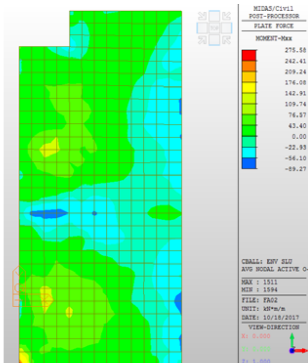
Figura 14 – Mxx: Inviluppo SLU
