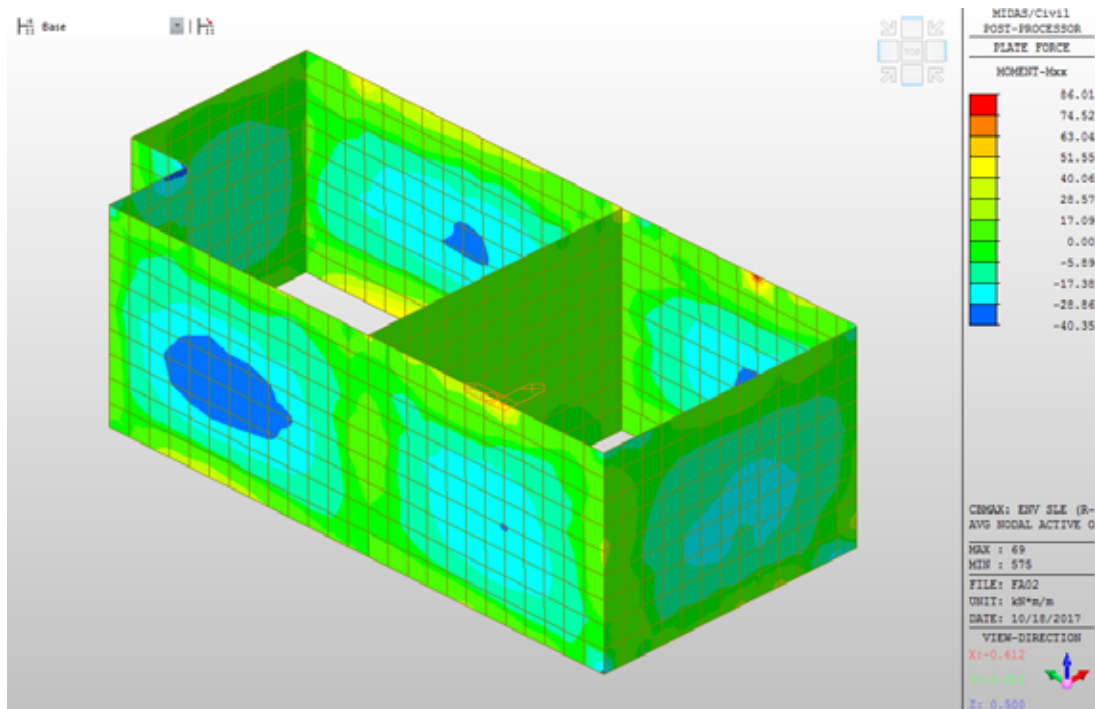
Figura 11 – Mxx: Inviluppo SLE
