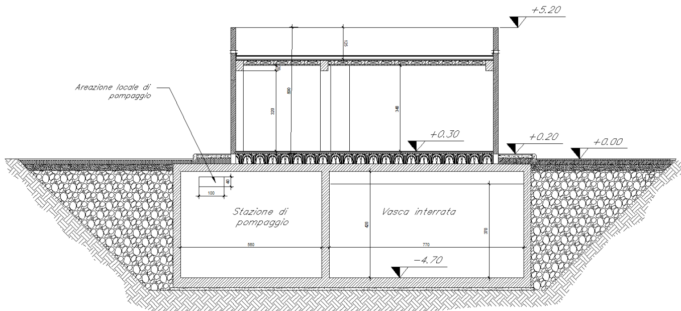
Figura 1 – Sezione Longitudinale
