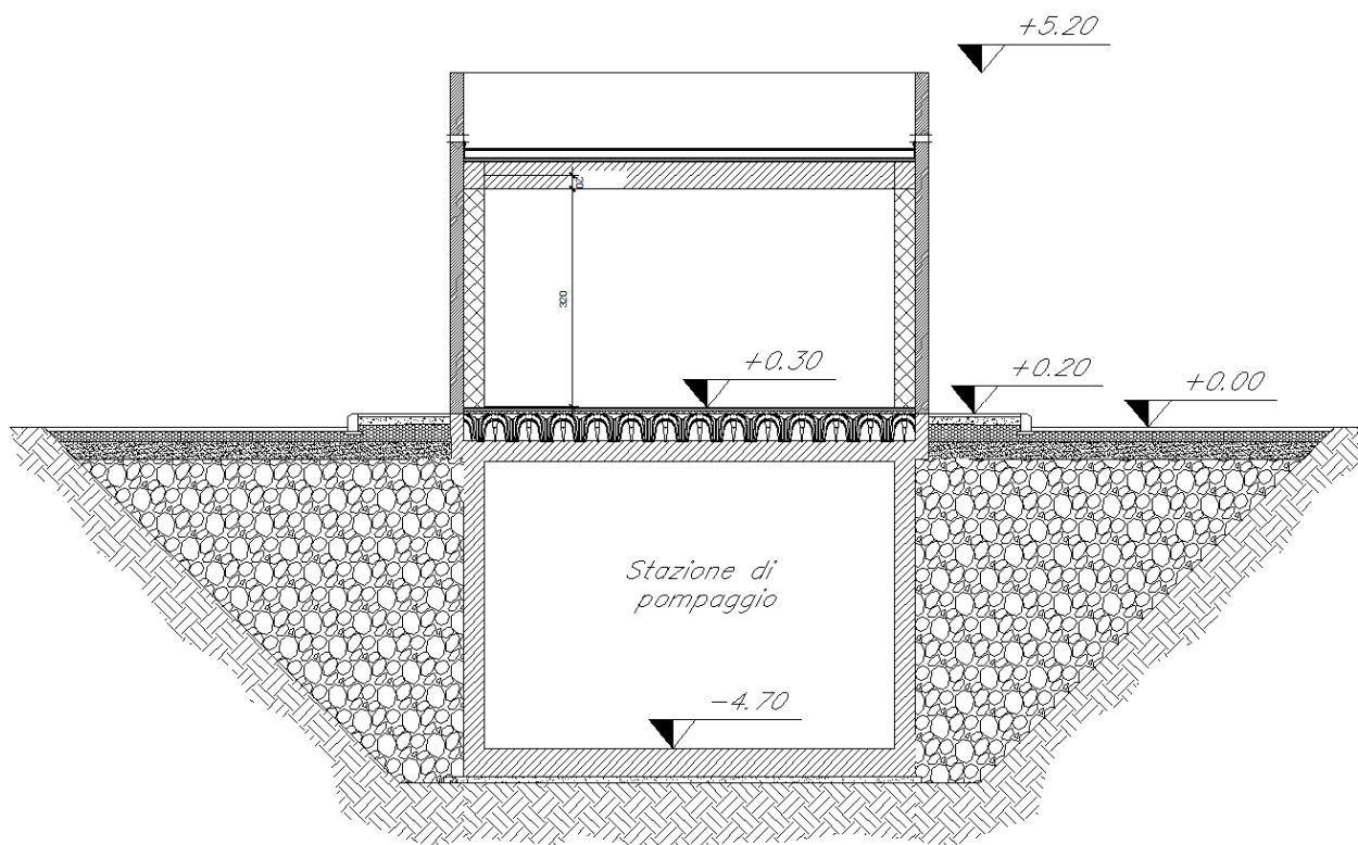
Figura 2 – Sezione Trasversale
