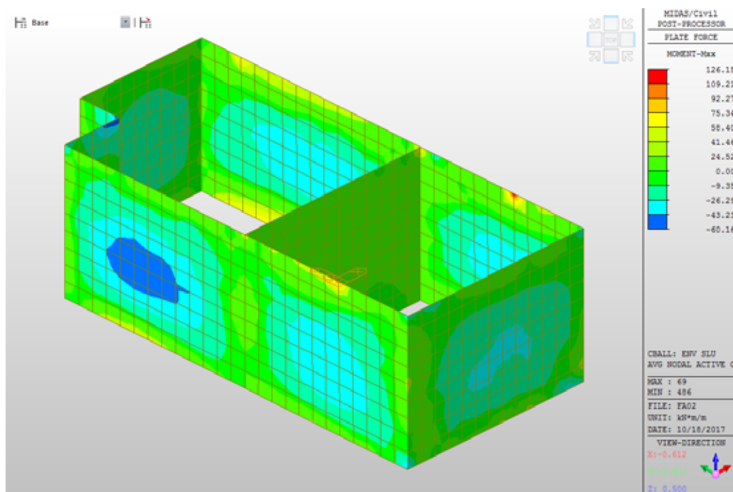
Figura 7 – Mxx: Involuppo SLU
