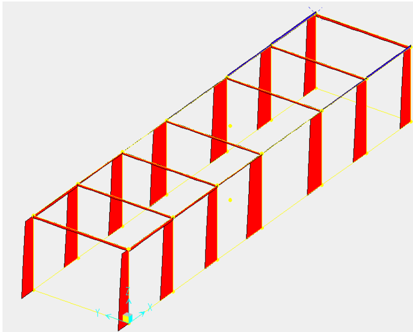
Figura 7-7 Diagramma del taglio N – COMB_INV_SLU.
