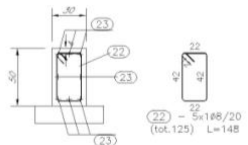
SEZIONE D-D
