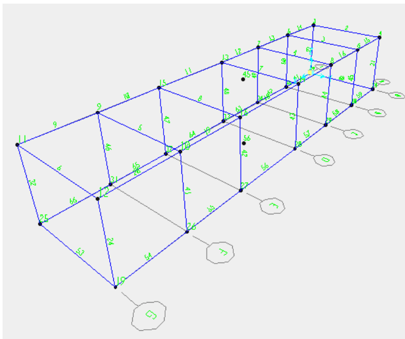
Figura 7-2 Numerazione frames e nodi
