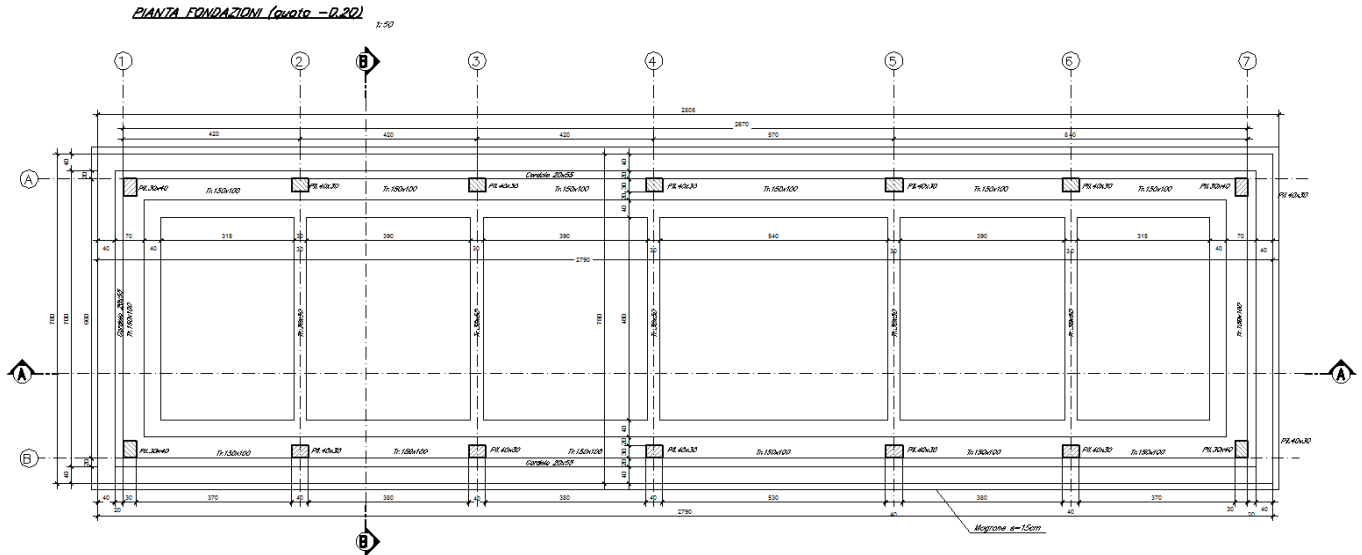
Figura 1 – Carpenteria Fondazione
