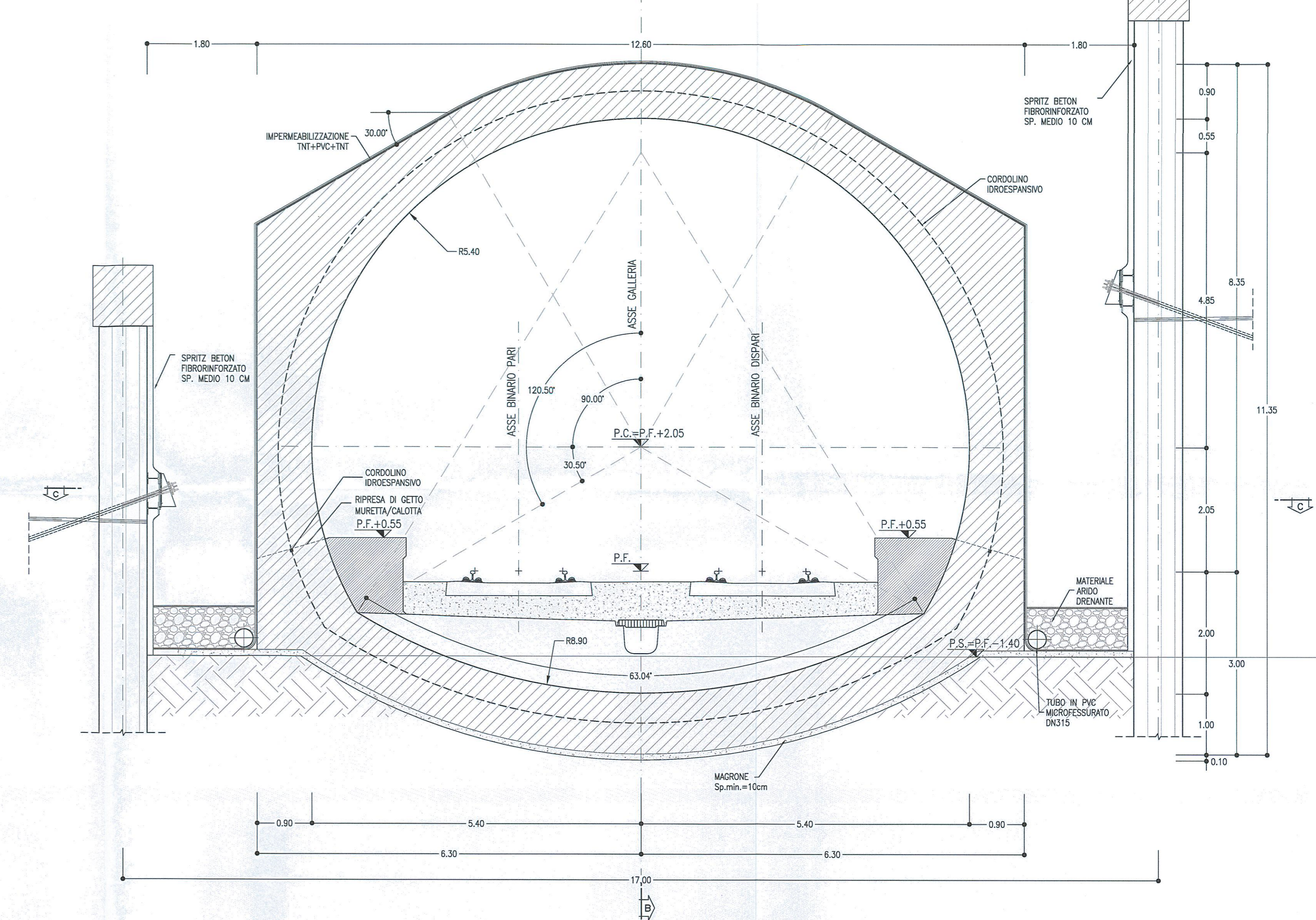
GALLERIA ARTIFICIALE POLICENTRICA SCALA 1:50 SEZIONE A-A
