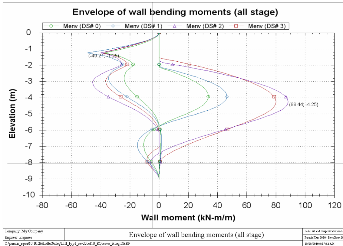
Figura 9.10 – Momento flettente - sezione tipo 1 – H_{scavo} = 4,5m
