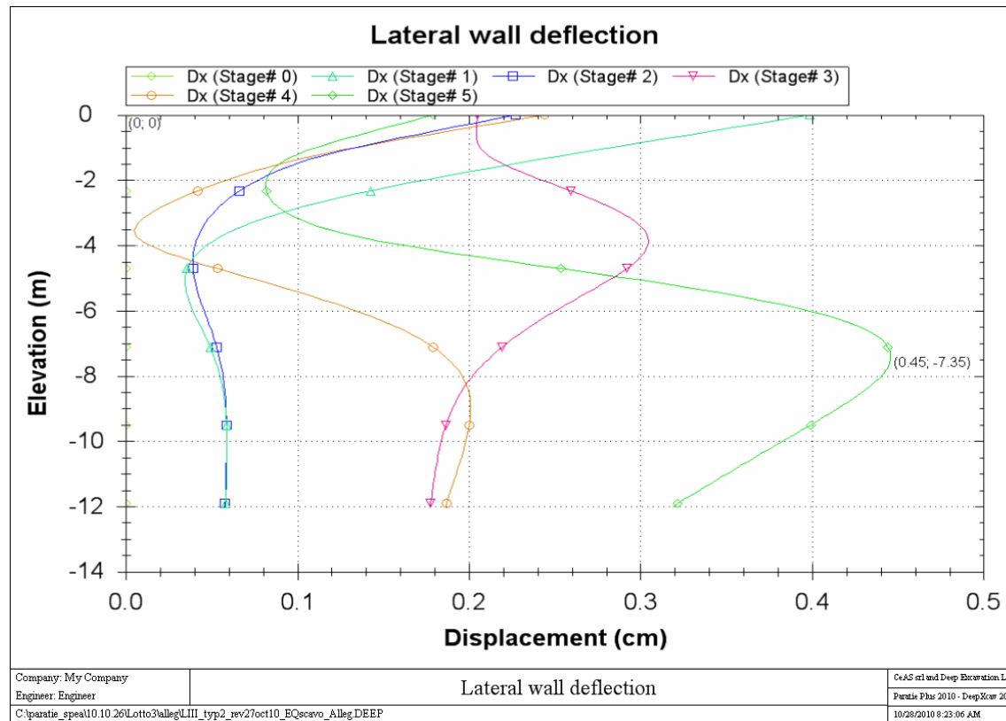
Figura 9.13 – Spostamento orizzontale - sezione tipo 2 – H_{scavo} = 6m
