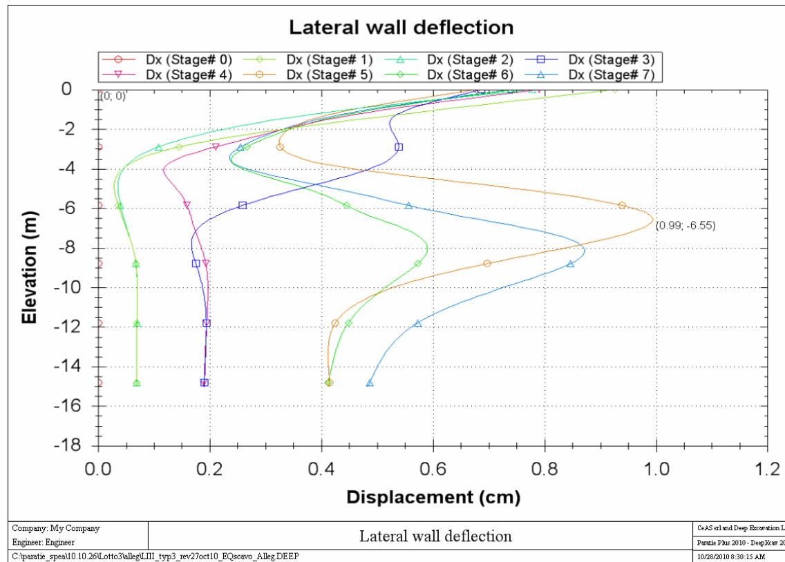
Figura 9.18 – Spostamento orizzontale - sezione tipo 3 – H_{scavo} = 7,5m
