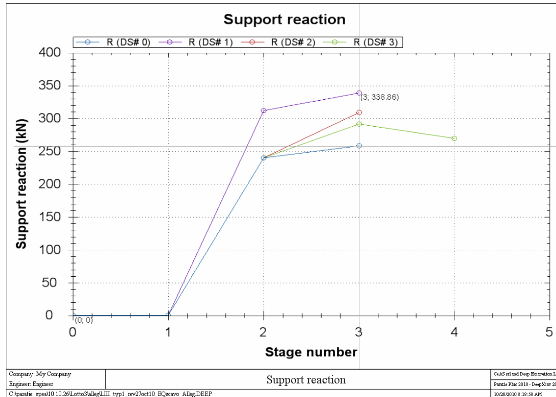
Figura 9.12 – Storia di carico nei tiranti - sezione tipo 1 – H_{\text{scavo}} = 4,5\text{m}
