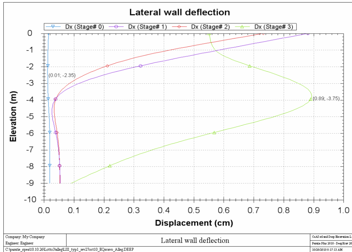
Figura 9.9 – Spostamento orizzontale - sezione tipo 1 – H_{scavo} = 4,5m
