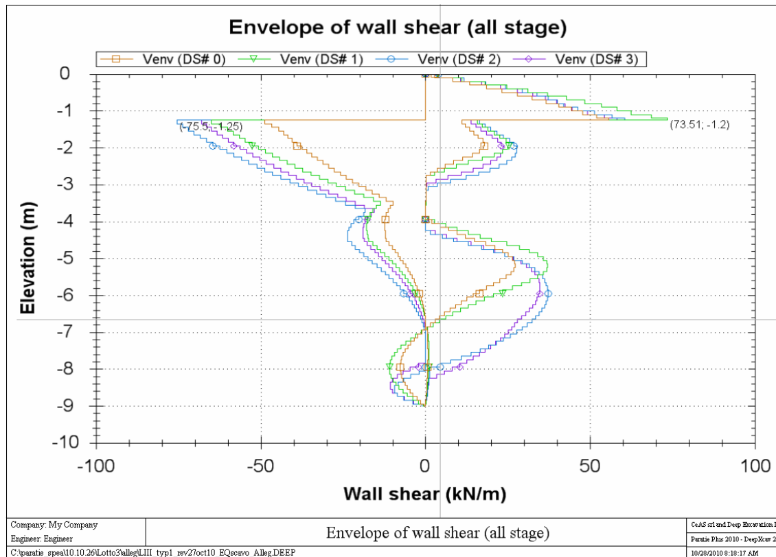
Figura 9.11 – Taglio - sezione tipo 1 – H_{scavo} = 4,5m
