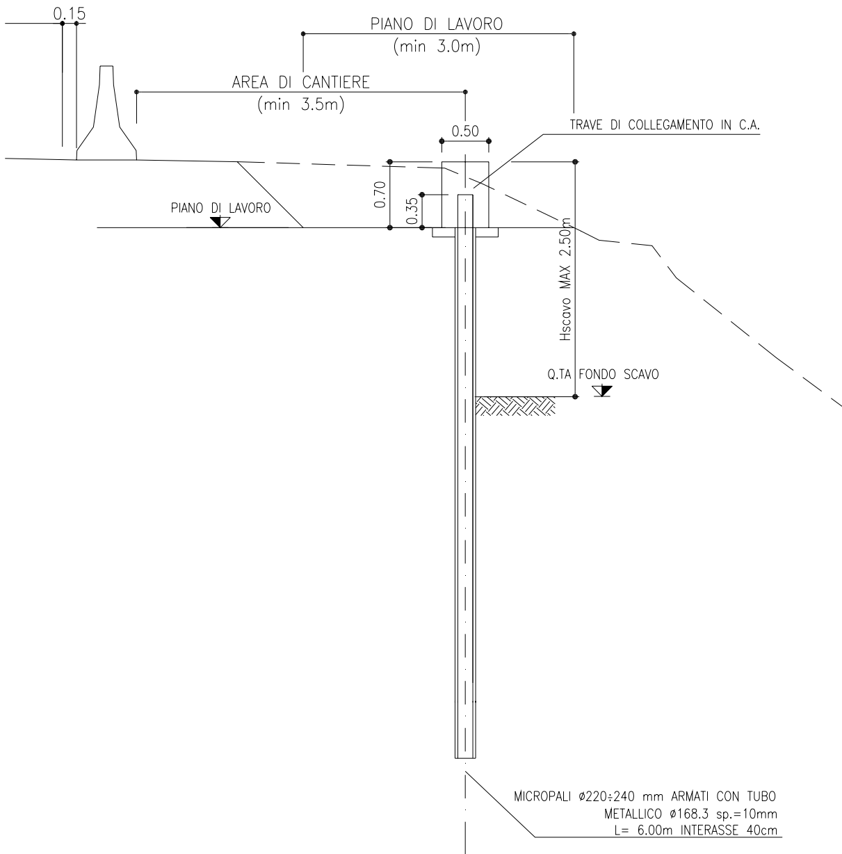
Figura 9.1 – Sezione trasversale paratia tipo 0 – H_{scavo} = 2,5m
