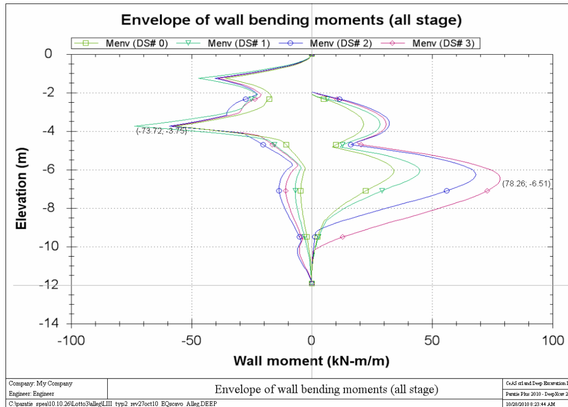
Figura 9.14 – Momento flettente - sezione tipo 2 – H_{scavo} = 6m
