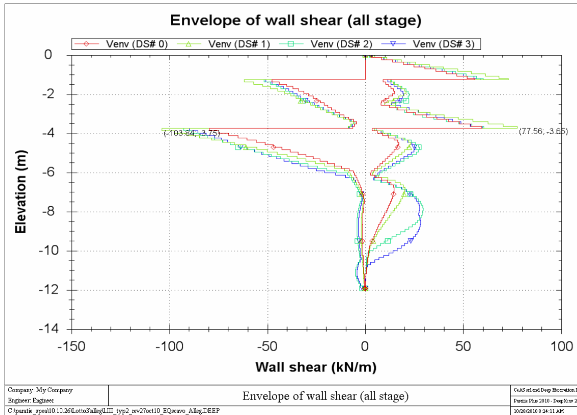
Figura 9.15 – Taglio - sezione tipo 2 – H_{scavo} = 6m
