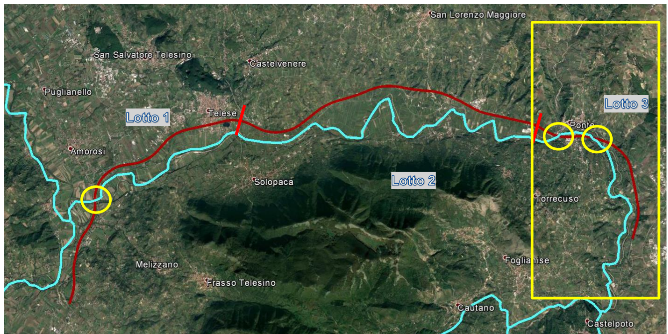
Figura 4-11 – Sezioni di attraversamento della linea ferroviaria sul Fiume Calore.
