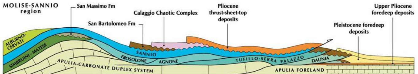
Figura 4-9 – Rappresentazione schematica dei rapporti geometrici tra le varie unità tettoniche dell'Appennino nella zona Molise-Sannio (da Patacca & Scandone 2007).
