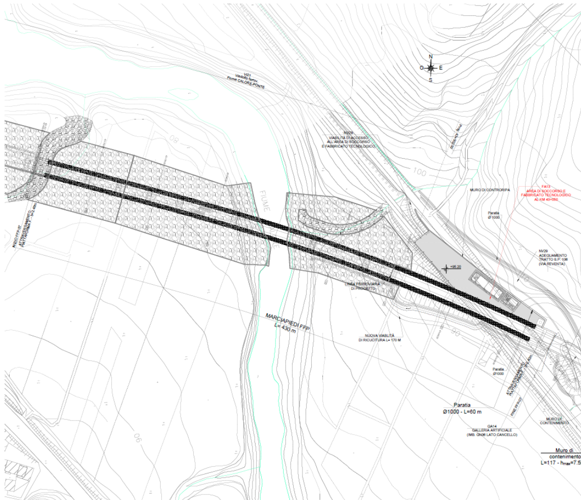
Figura 3-2 – Planimetria generale_FA13 – pk. 43+050
