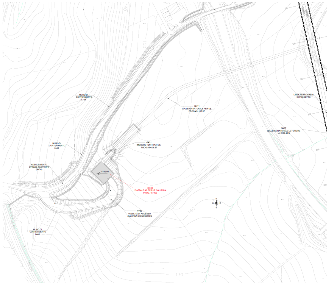
Figura 3-4 - Planimetria generale_RI106 – pk. 45+100
