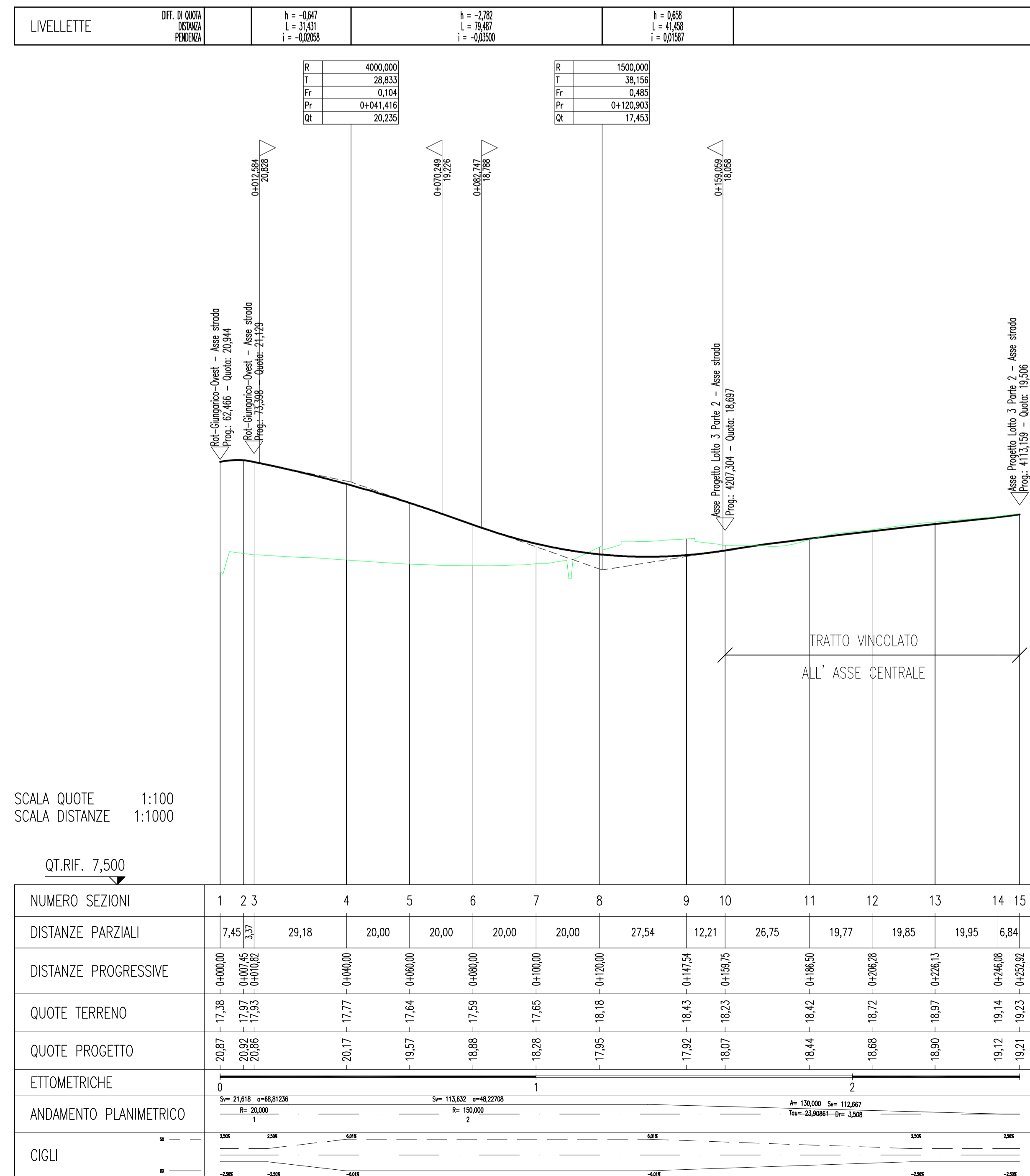
PROFilo LONGITUDINALE RAMPA RS13
