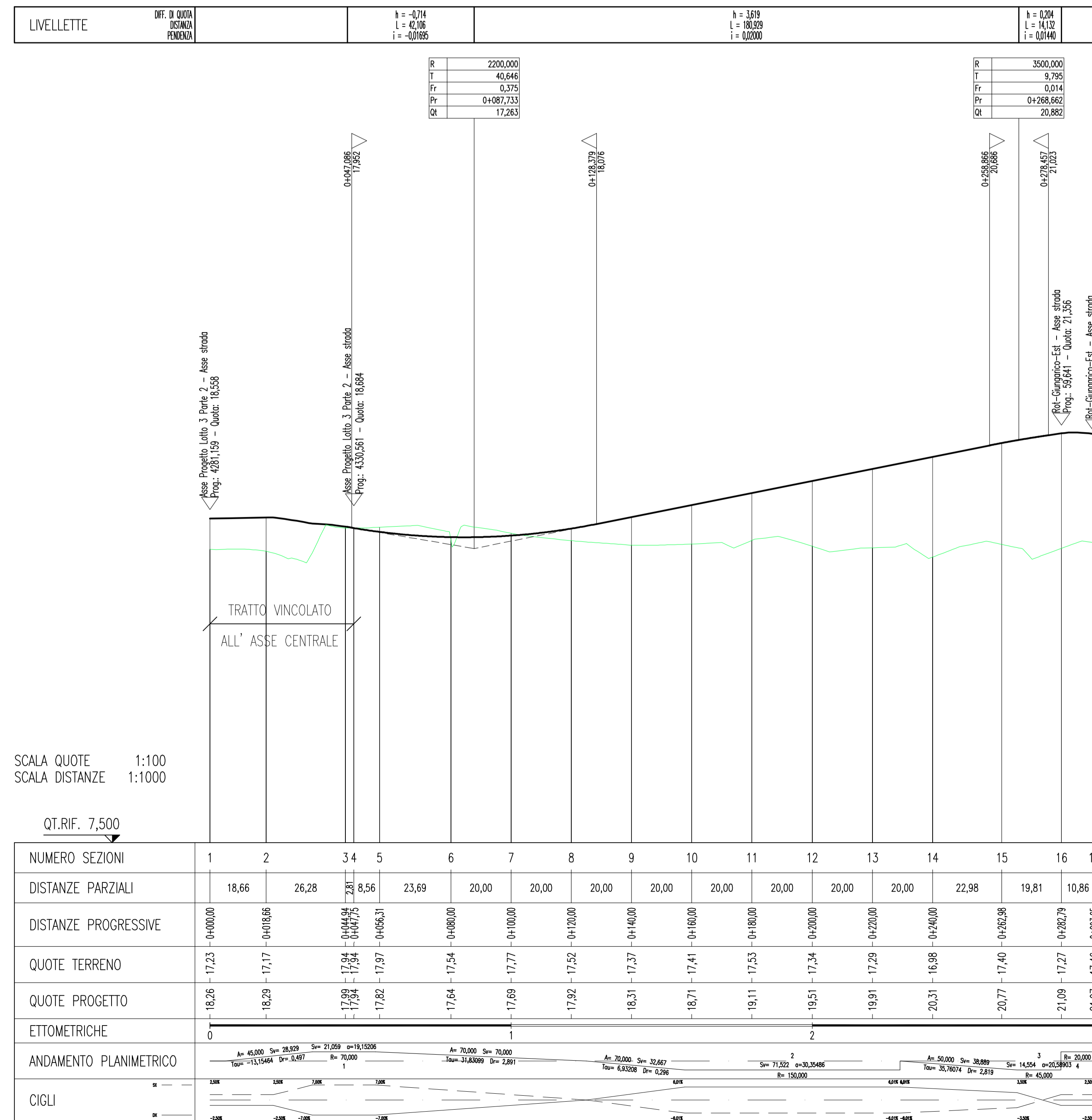
PROFilo LONGITUDINALE RAMPA RS14
