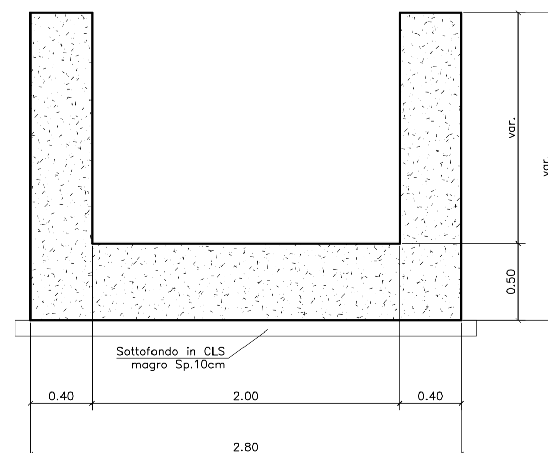
SEZIONE C-C SCALA 1:25
