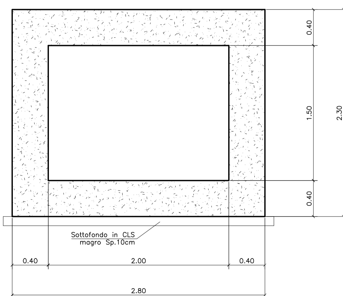
SEZIONE B-B SCALA 1:25
