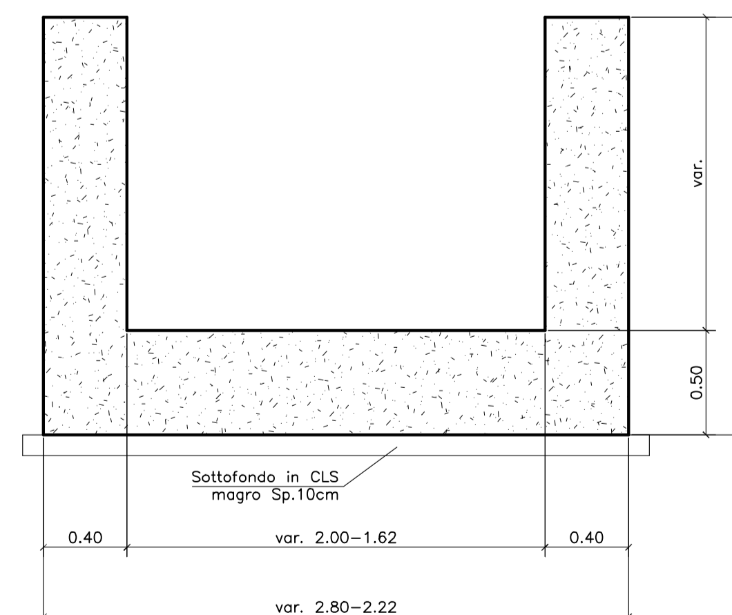
SEZIONE D-D SCALA 1:25
