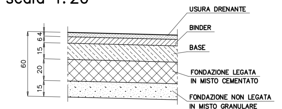
PARTICOLARE PAVIMENTAZIONE scala 1:20
