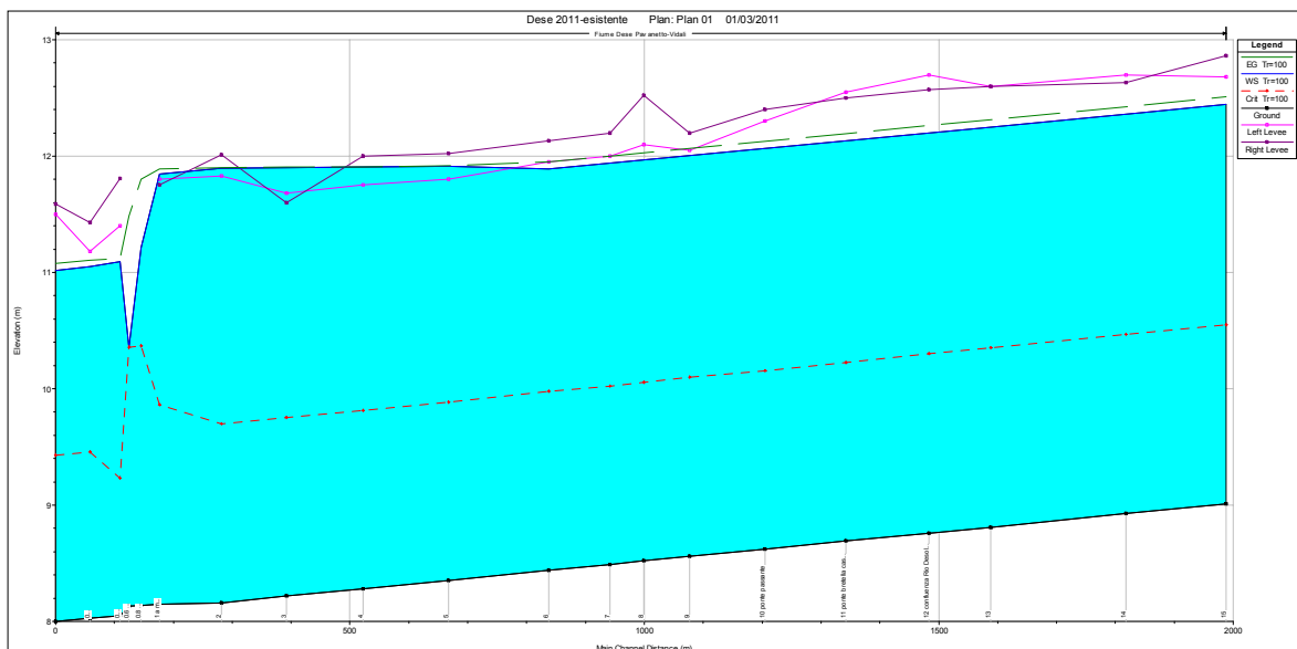
Figura 29- Profilo idraulico piena centenaria nelle condizioni attuali (è evidente il rigurgito causato dalla strettoia del mulino Vidali e l'esonazione in sx)
