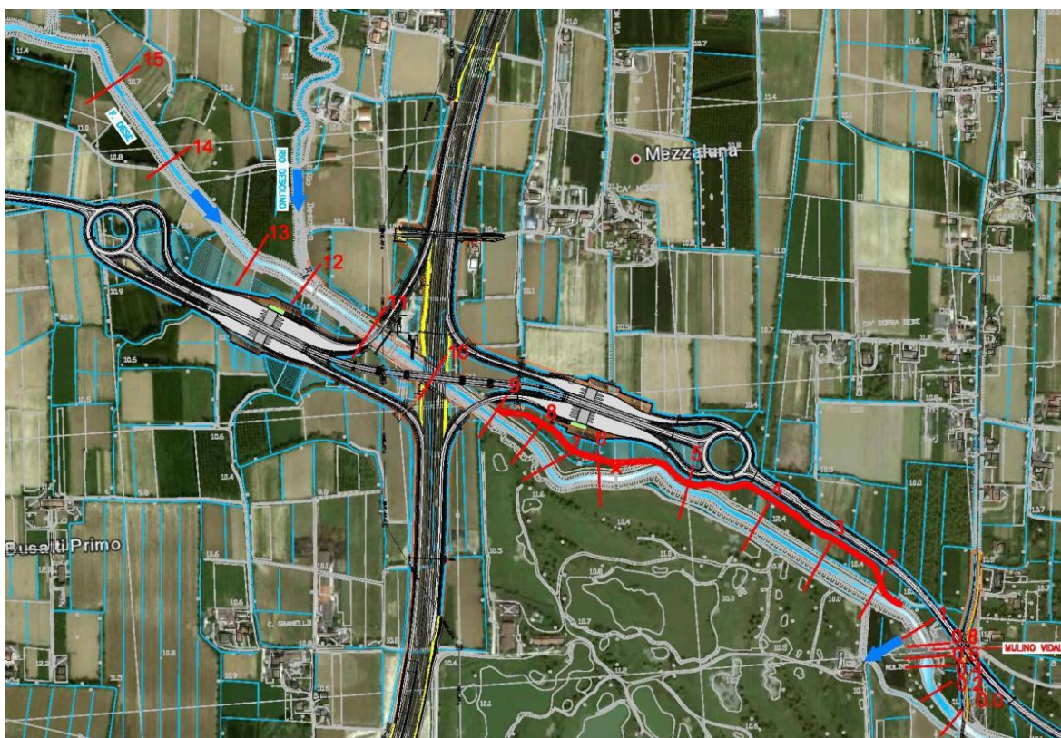
Figura 32- Stralcio di ortofoto con indicazione dei punti di sovrizzo arginale nella condizione di progetto del corso d'acqua con il nuovo argine in sinistra (sez. 2-9)
