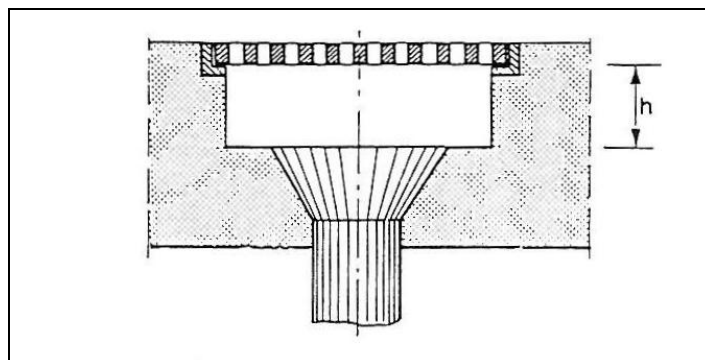
Figura 52: schema del sistema griglia-bocchettone per la raccolta delle acque dagli impalcati dei ponti e viadotti
