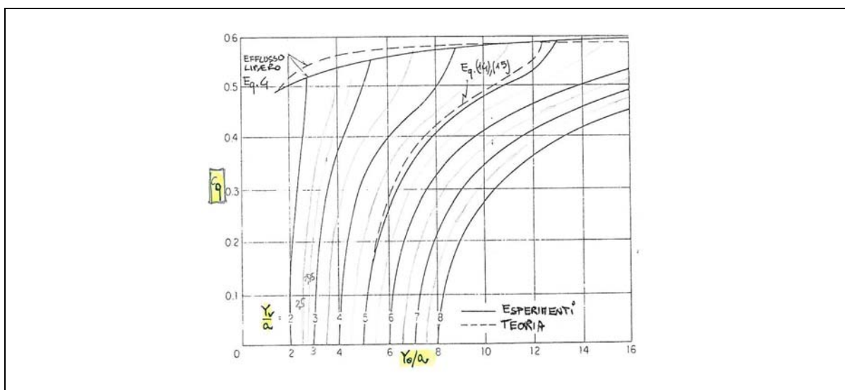
Figura 61 – Andamento del coefficiente di portata C_q in funzione del grado di apertura della paratoia y_0/a nel caso di efflusso rigurgitato. Confronto tra i dati sperimentali di Henry e i coefficienti di portata teorici.
