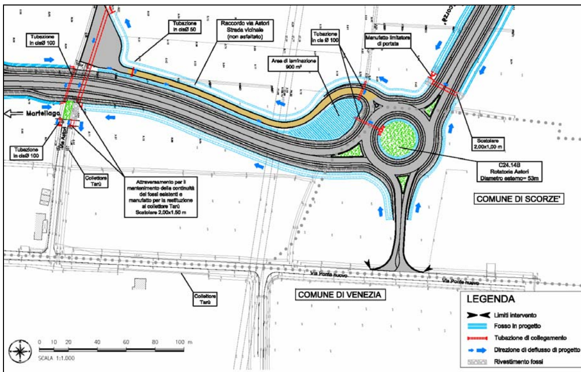
Figura 66 – Schema costruttivo nuova rotonda Via Astori e tombinamento collettore Tarù.
