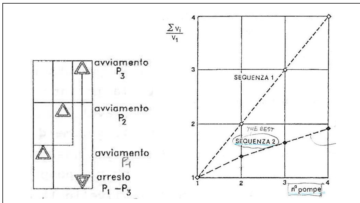
Figura 49 – Funzionamento pompe in “sequenza 2” e grafico dei volumi utili da assegnare alle vasche nel caso di pompe tutte uguali ( Q_i = Q_1 e T_{ci} = T_{c1} )
