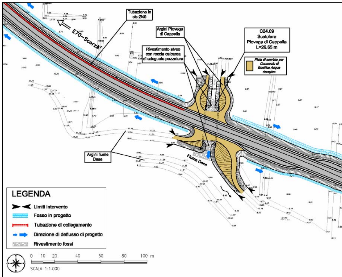
Figura 64 – Schema costruttivo nuovo ponte scatolare sul piovega di Cappella.
