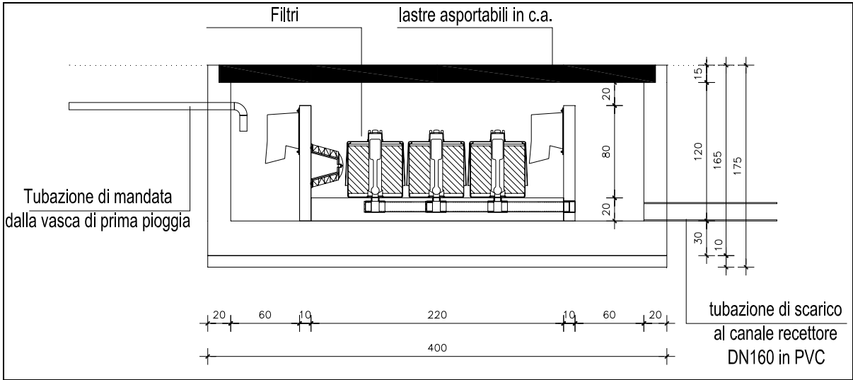
Figura 47- Schema tipo impianto trattamento acque prima pioggia con sistema a cartucce filtranti ricaricabili
