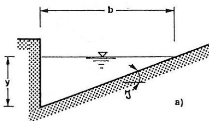
Figura 48: cunetta alla francese a sezione triangolare
