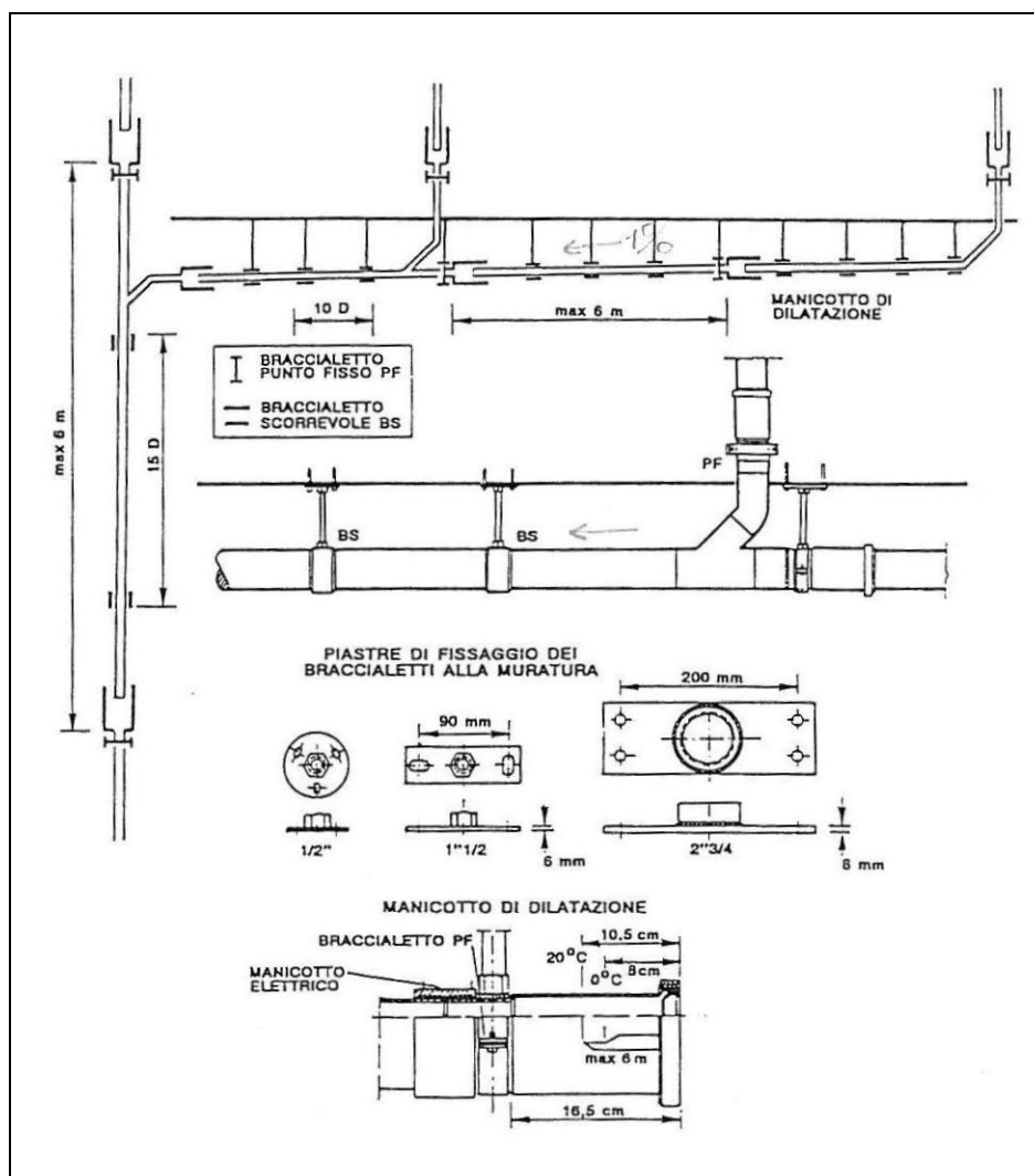
Figura 53: schema tipo di ancoraggio delle condotte di scarico alle travi ed alle pile dei viadotti.
