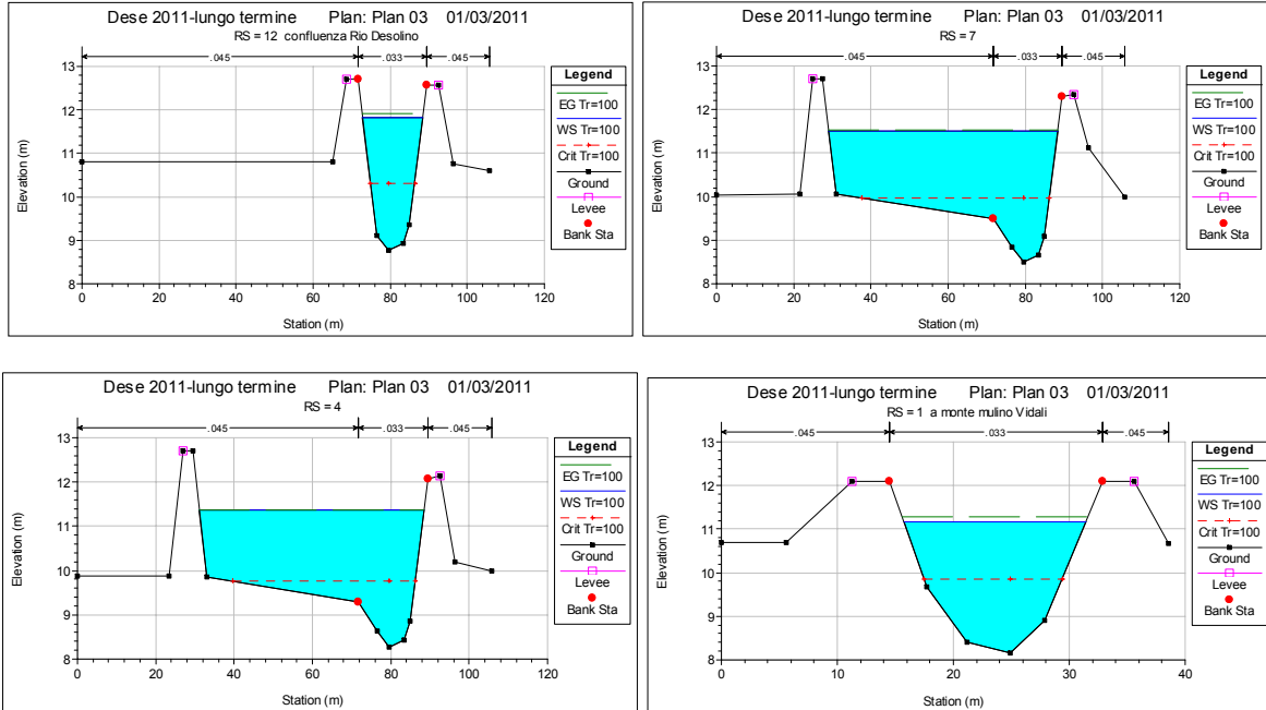
Figura 39- Sezioni idrauliche caratteristiche F. Dese a seguito del passaggio di un'onda di piena centenaria nelle condizioni di progetto e con l'operatività del manufatto di by-pass del mulino Vidali (si nota una diminuzione dei livelli di piena di circa 50-60 cm a valle della sez. 9; sparisce il passaggio in condizioni critiche in corrispondenza della strettoia del mulino e quindi anche il profilo di rigurgito a monte)
