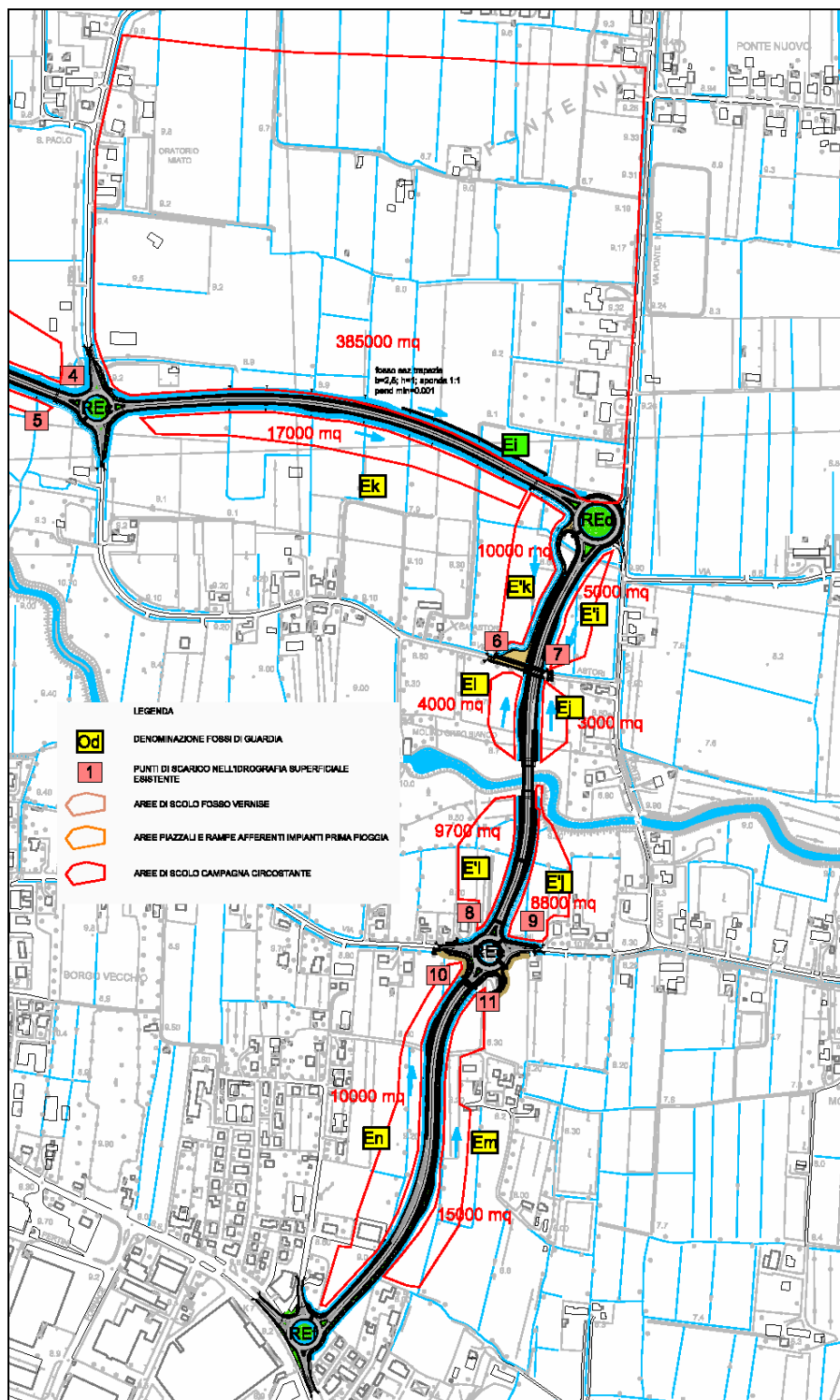
Figura 58- Tratto Est (2), schema identificativo fossi di guardia, aree campagna di pertinenza fossi guardia e punti di consegna nell'idrografia superficiale
