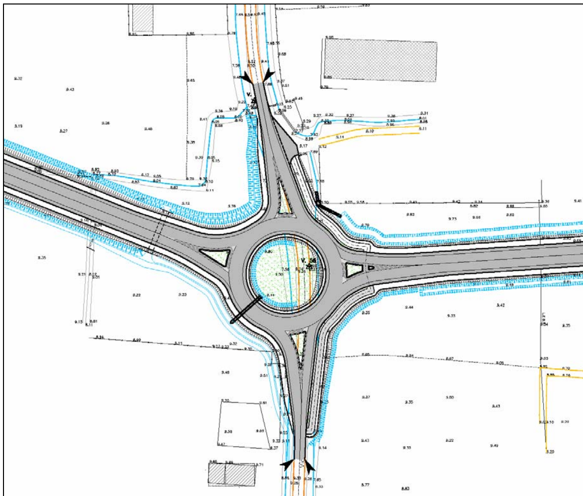
Figura 65 – Schema costruttivo nuova rotonda San Paolo e regimazione dei relativi fossati
