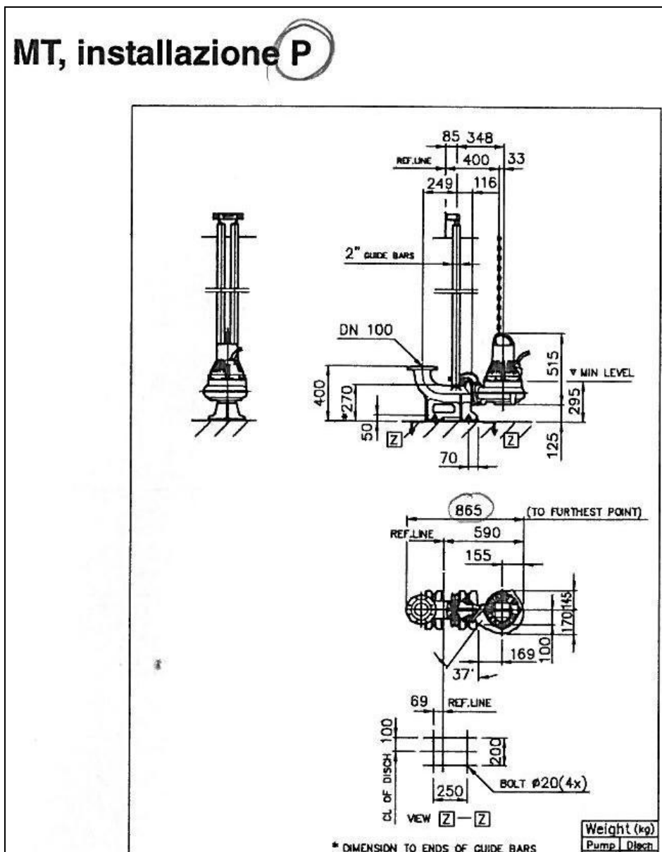
Figura 50 – Schema tipo per installazione di elettropompe in impianti di sollevamento per sottopassi stradali
