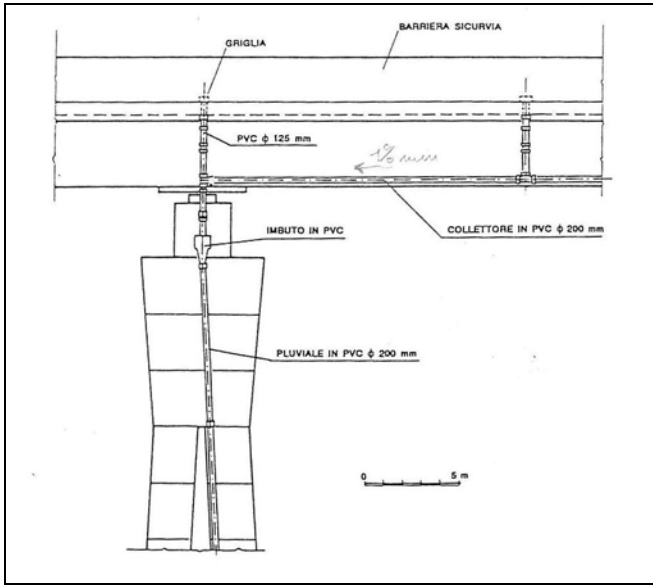
Figura 51: schema tipo smaltimento acque dai ponti e viadotti
