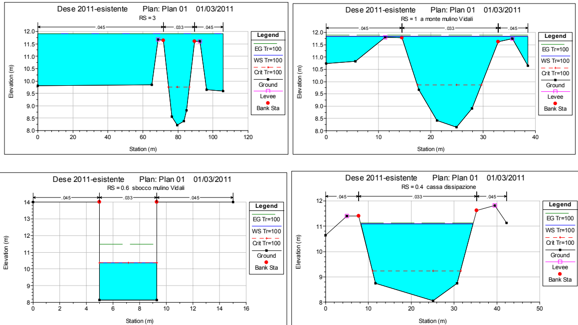
Figura 30- Sezioni idrauliche caratteristiche F. Dese a seguito del passaggio di un'onda di piena centenaria nelle condizioni attuali (si nota l'esonazione in sinistra a valle della sez.6; l'esonazione in destra a monte del mulino presso la sez.1-3; il passaggio in condizioni critiche in corrispondenza della strettoia del mulino ed il successivo risalto nella cassa di dissipazione di valle)
