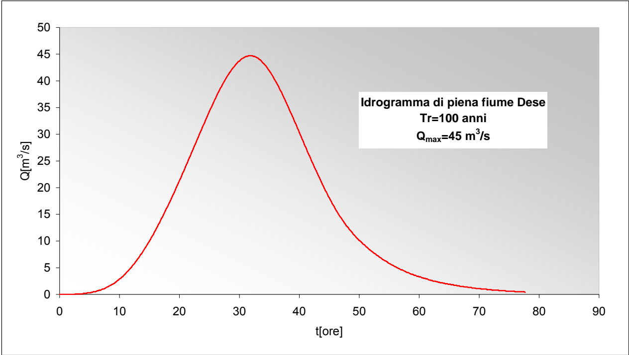
Figura 22 - Idrogramma di piena
