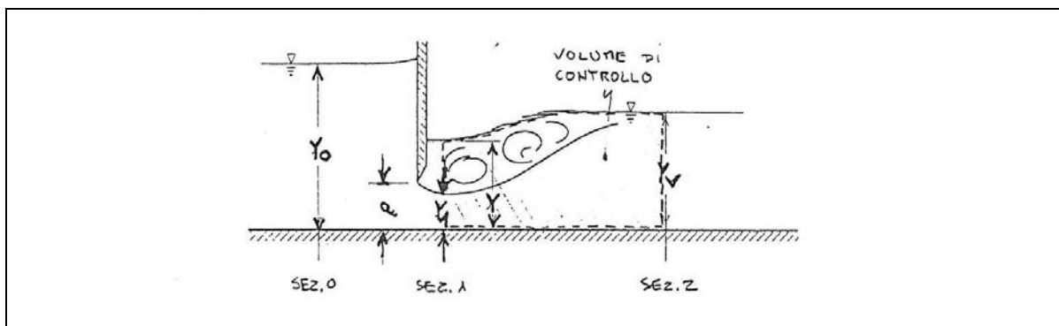
Figura 60 – Schema di una paratoia a funzionamento sotto battente rigurgitato
