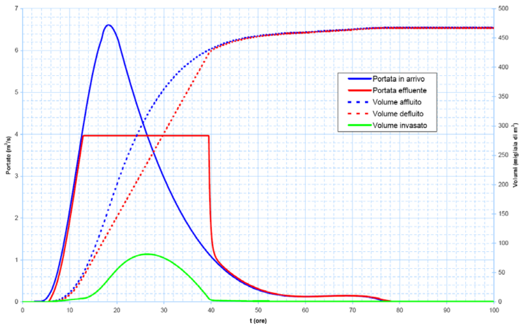
Figura 36 – Comportamento della cassa di espansione per un evento con T_R = 2 anni; invasando sino a 0,50 m dalla sommità arginale il colmo di piena risulta ridotto da 6,81 a 3,97 m^3/s .
