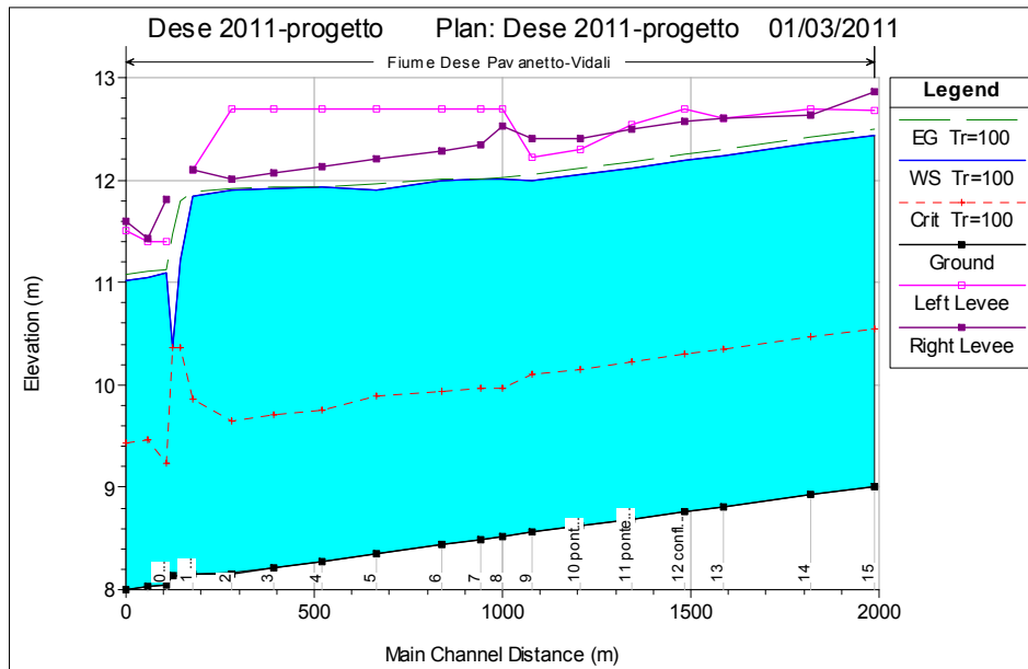
Figura 33- Profilo idraulico piena centenaria nelle condizioni di progetto (è ancora evidente il rigurgito causato dalla strettoia del mulino Vidali)
