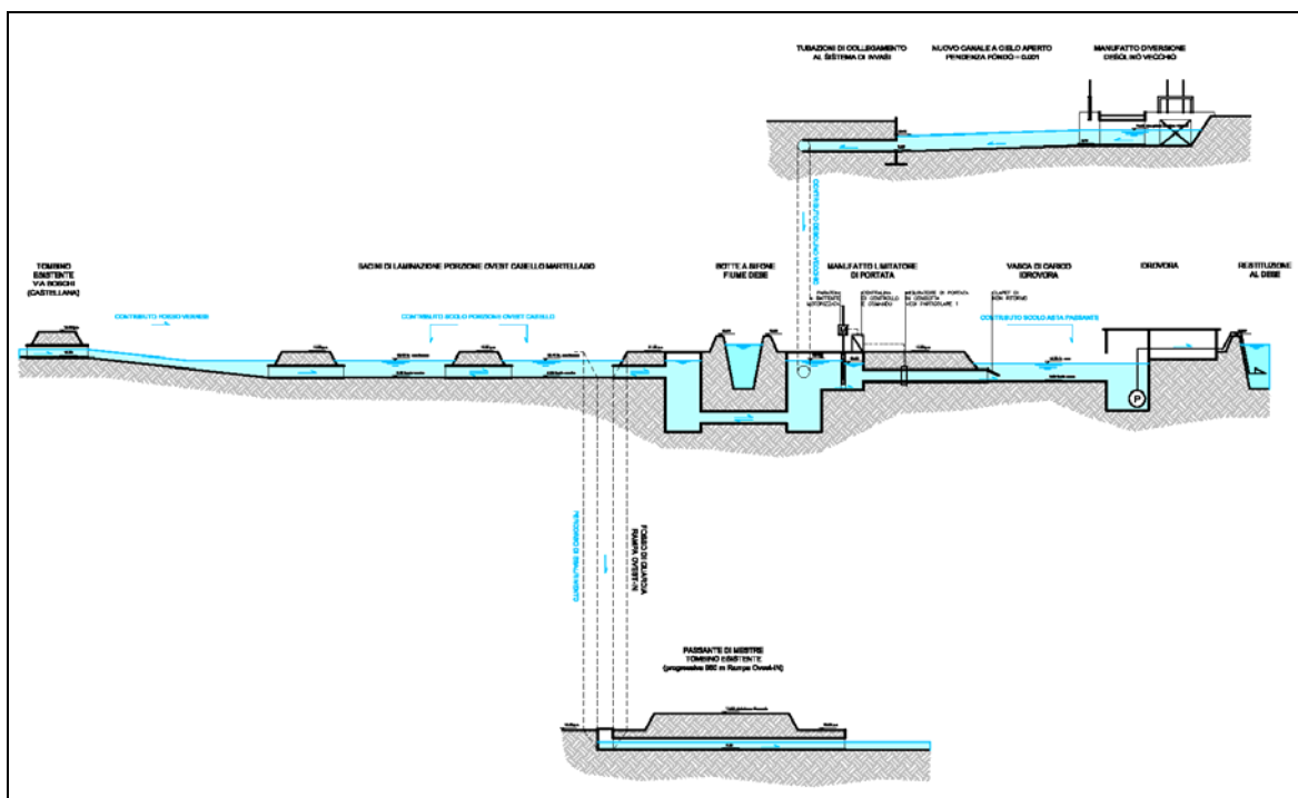
Figura 44 – Profilo idraulico schematico del sistema di invasi
