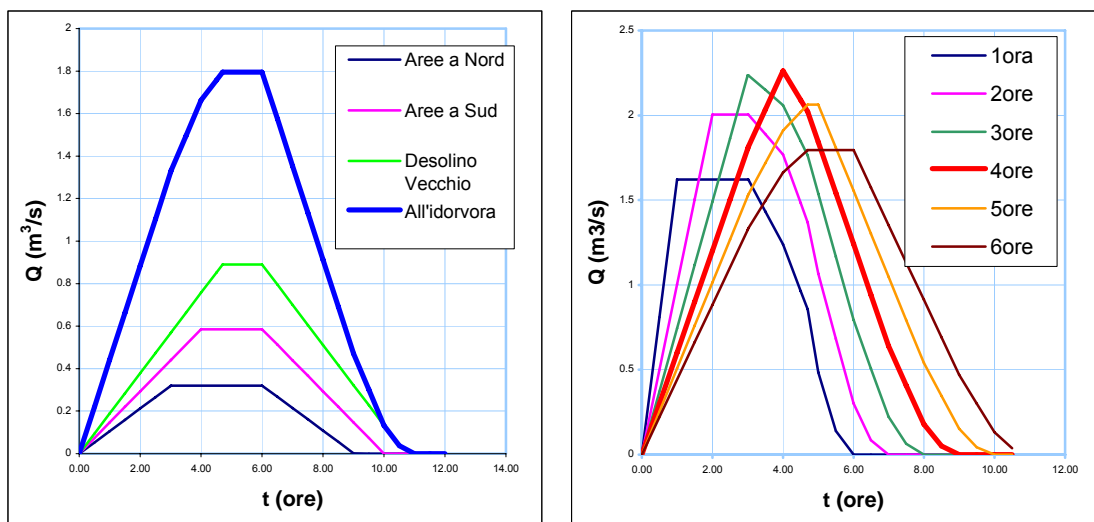
Figura 41 – Applicazione del metodo di Turazza per TR = 50 anni a: le curve di portata per ciascun sottobacino e la risultante dalla loro somma per un tempo di pioggia pari a 6 ore (a sinistra) e le curve di portata complessive per diverse durate dell'evento di pioggia (a destra)
