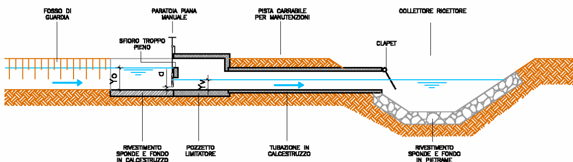
Figura 59 – Schema manufatto limitatore di portata allo scarico fossa di guardia Ek
