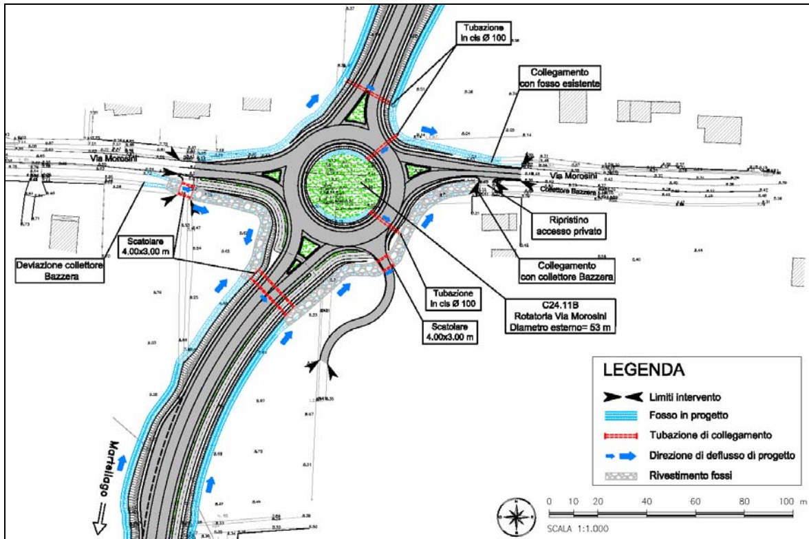
Figura 67 – Schema costruttivo nuova rotonda Via Morosini e deviazione collettore Bazzera.
