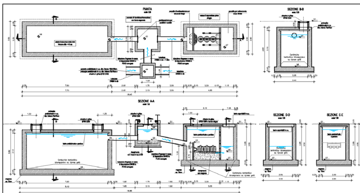
Figura 46- Schema costruttivo impianti di trattamento acque di prima pioggia
