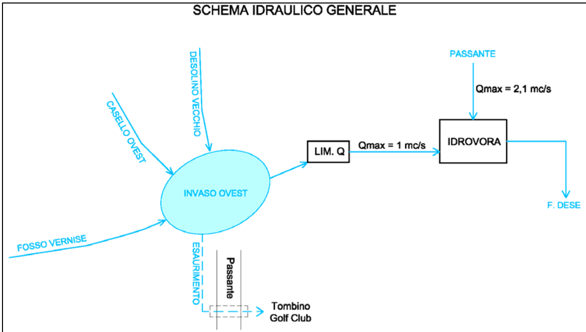
Figura 43 – Schema idraulico generale del sistema di invasi previsto a ovest del nuovo casello di Martellago
