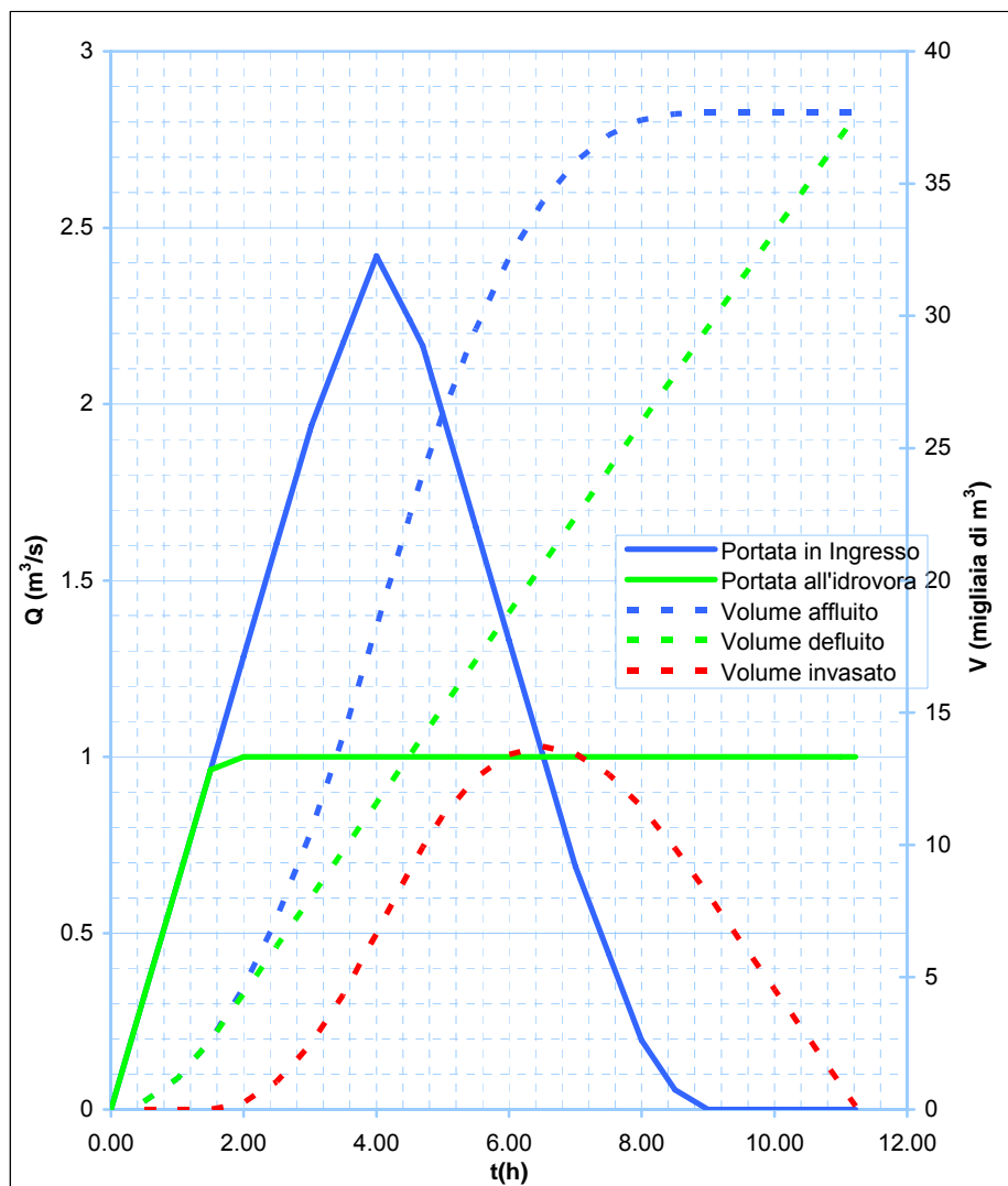
Figura 42 – Comportamento del bacino di laminazione per un evento di pioggia di durata 4 ore con TR 50 anni nelle ore successive all'inizio dell'evento di pioggia: in linea continua le portate in arrivo dal compressorio (blu) e avviata all'idrovora (verde), in linea spezzata le cumulate dei volumi in entrata, in uscita e la loro differenza, corrispondente al volume invasato
