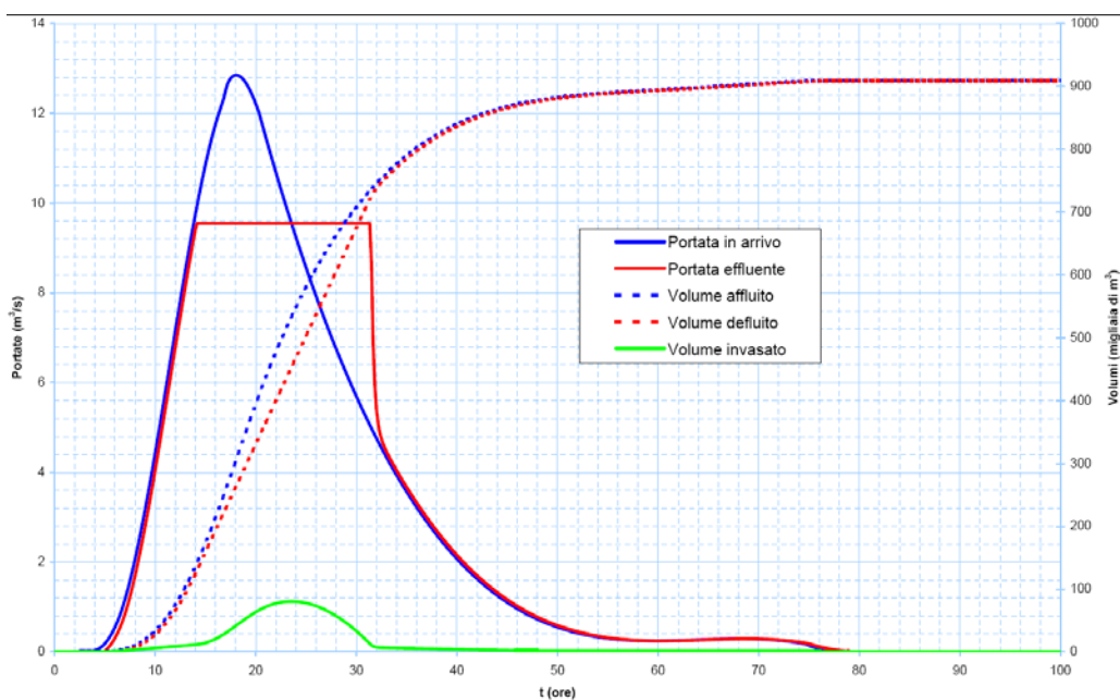
Figura 37 – Curve rappresentative del massimo abbattimento possibile con T_R = 5 anni; considerando un franco di 0,5 m dalla sommità arginale, il valore al colmo è ridotto da 12,85 a 9,85 m^3/s
