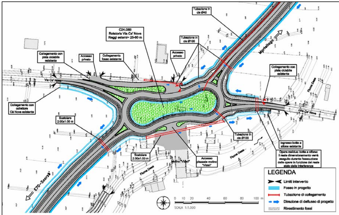
Figura 63 – Schema costruttivo nuova rotonda Cà Nove e deviazione collettore Cà Nove.
