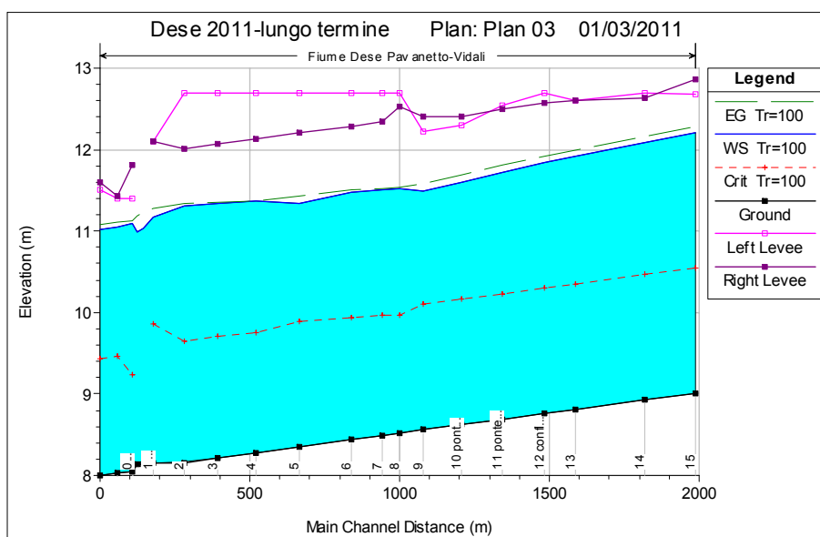
Figura 38- Profilo idraulico piena centenaria con l'opera di by-pass mulino Vidali (la corrente si mantiene sempre in condizioni subcritiche eliminando il rigurgito a monte del mulino)
