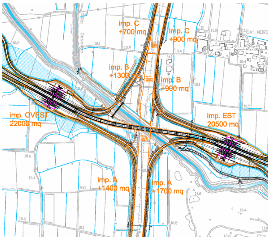
Figura 45- Aree di pertinenza impianti di prima pioggia esistenti (A,B,C) e di progetto (est; ovest)
