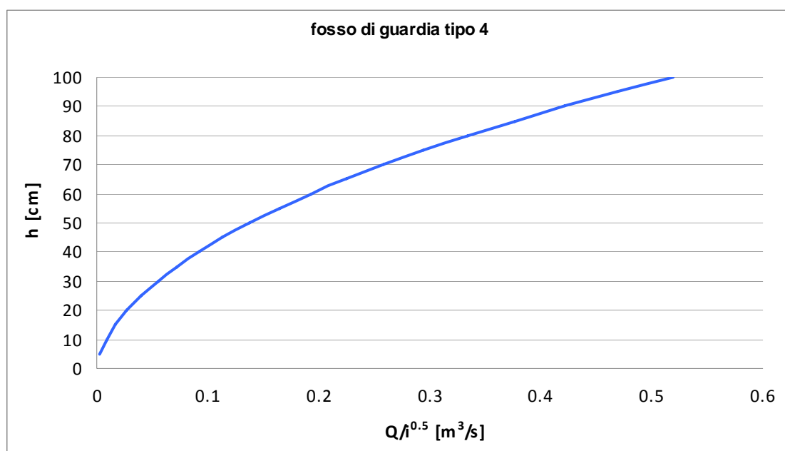
Figura 55- Scale di deflusso dei fossi di guardia
