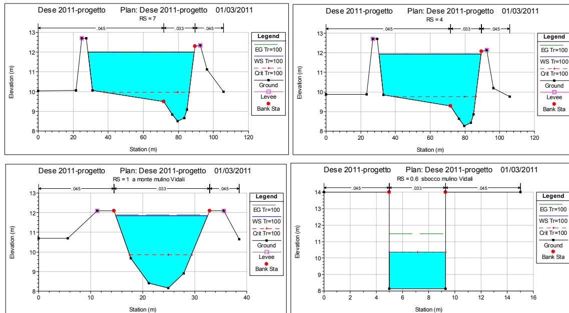
Figura 34- Sezioni idrauliche caratteristiche F. Dese a seguito del passaggio di un'onda di piena centenaria nelle condizioni di progetto (si nota che le golene in sinistra contengono l'onda di piena; resta il passaggio in condizioni critiche in corrispondenza della strettoia del mulino ed il successivo risalto nella cassa di dissipazione di valle)
