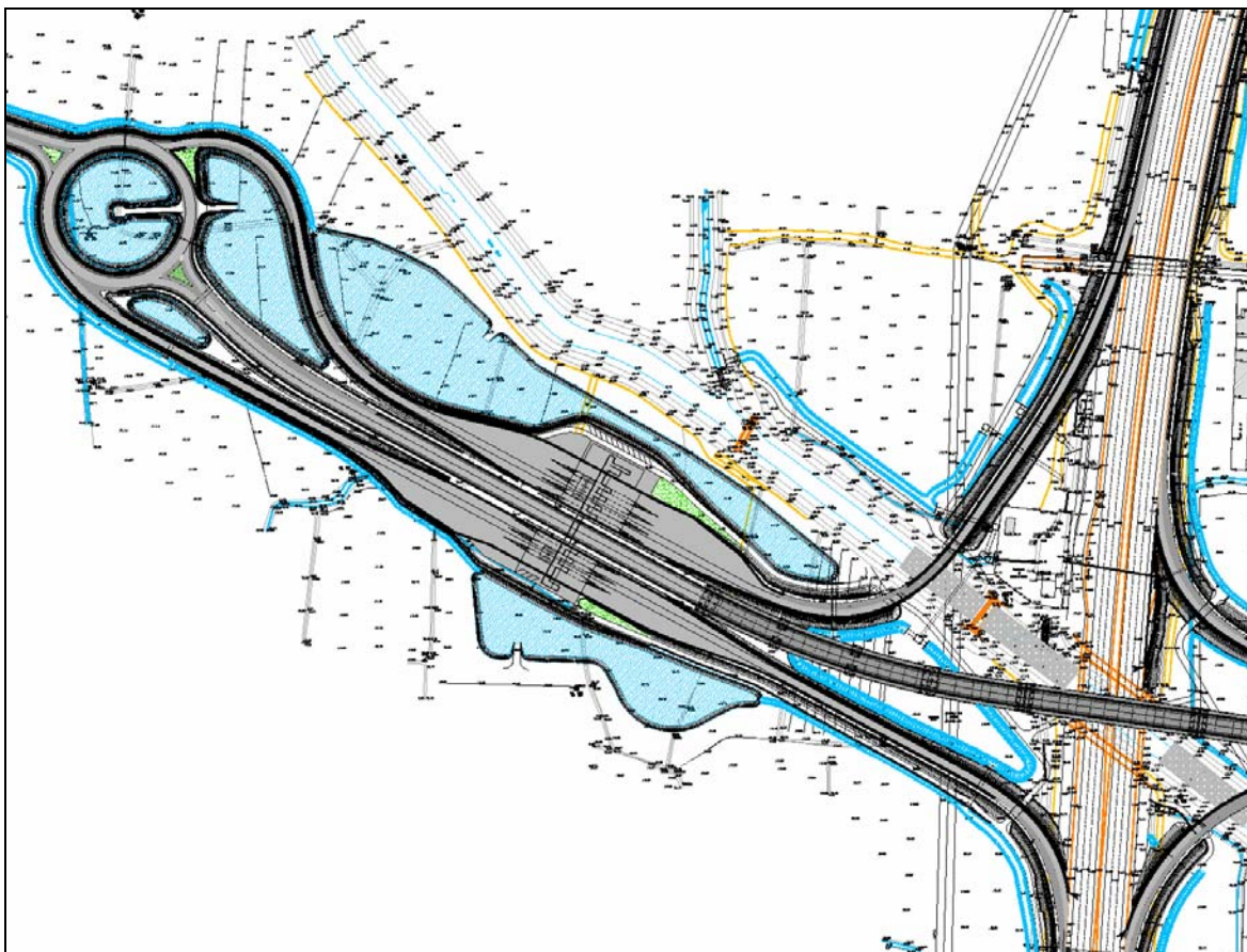
Figura 17-Area di laminazione alla destra idrografica del fiume Dese
