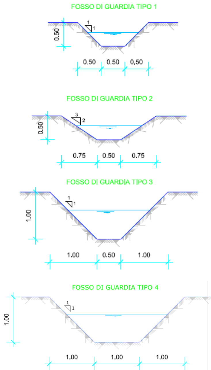
Figura 54- Sezioni tipo dei fossi di guardia
