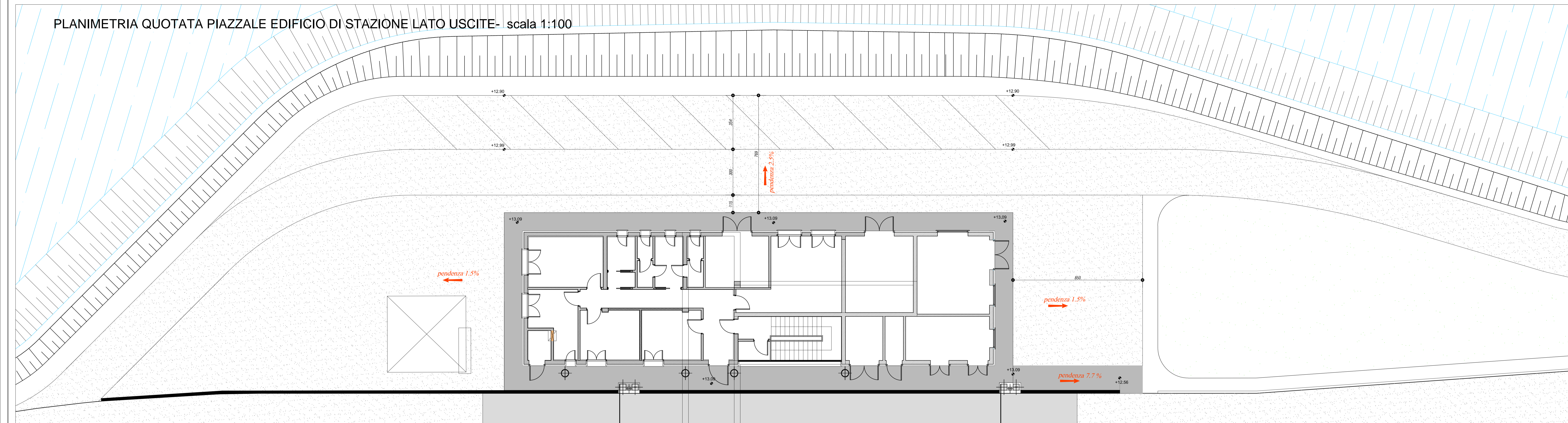
PLANIMETRIA QUOTATA PIAZZALE EDIFICIO DI STAZIONE LATO ENTRATE- scala 1:100
