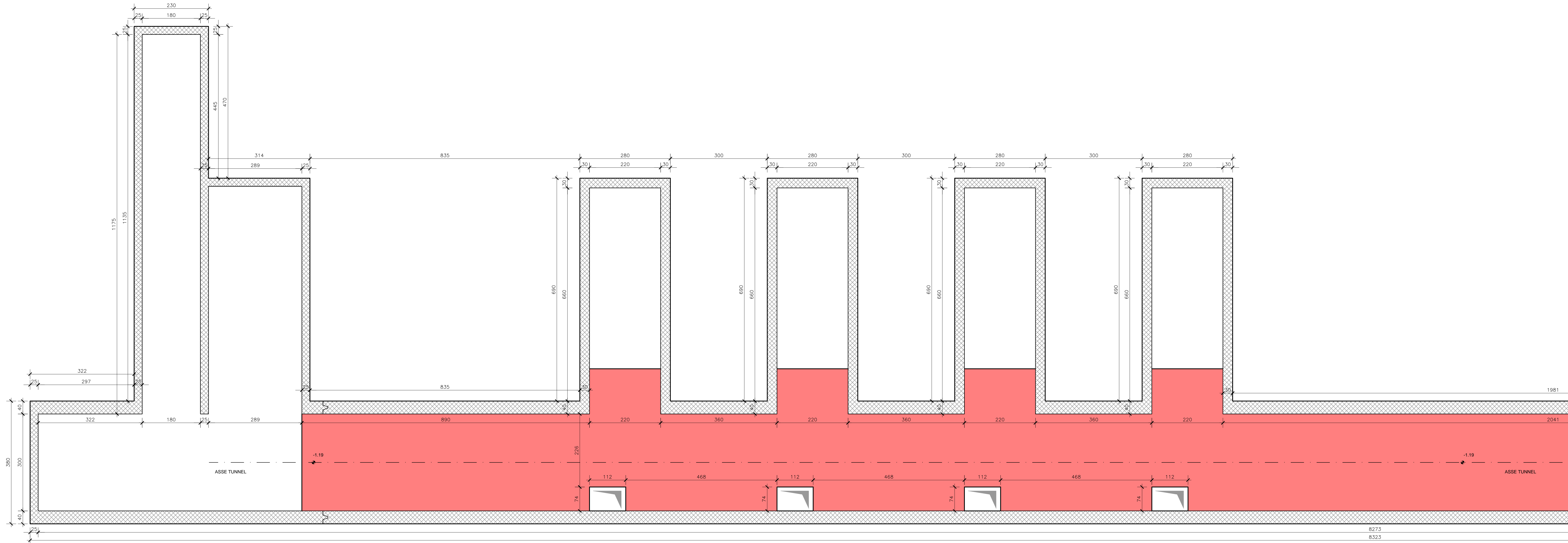
PIANTA 1° ORIZZONTAMENTO LATO USCITE - Scala 1:50
