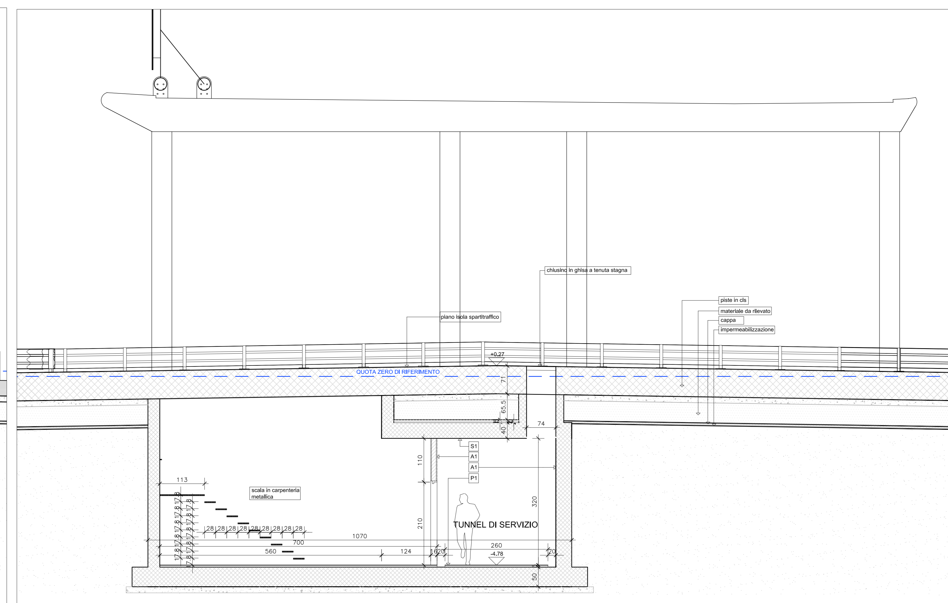
Sezione 2 - scala 1:50
