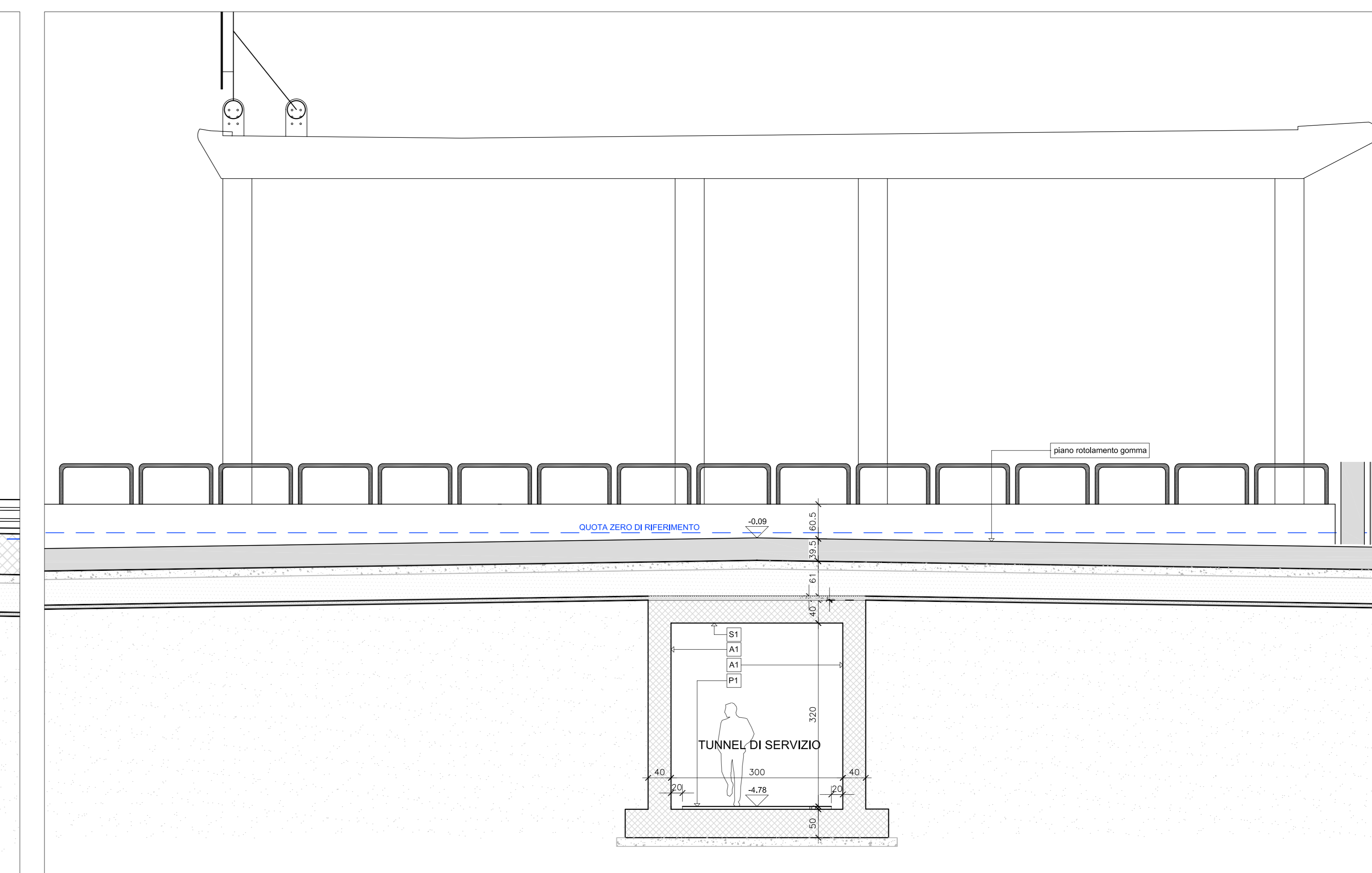
Sezione 6 - scala 1:50
