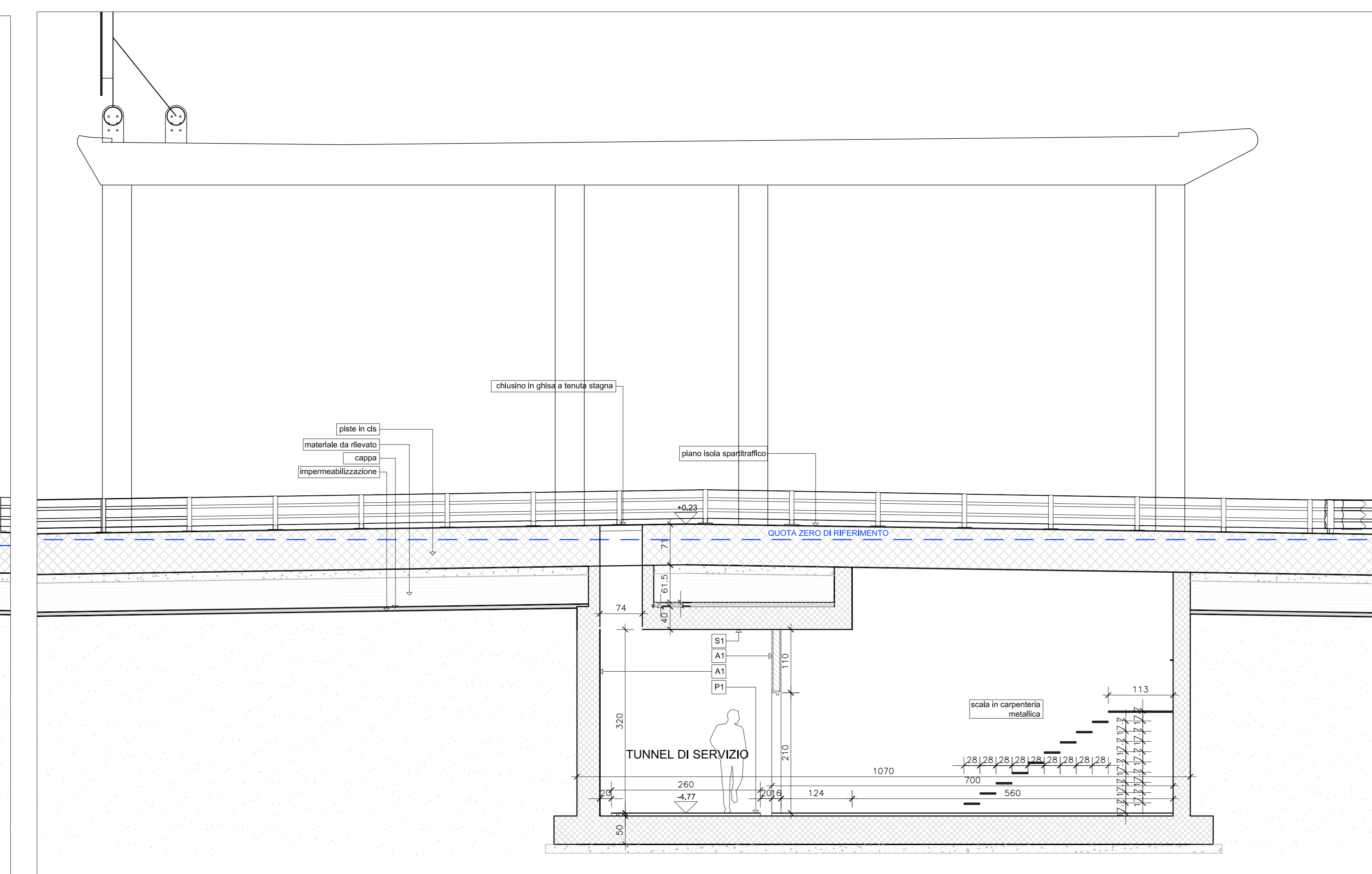
Sezione 5 - scala 1:50
