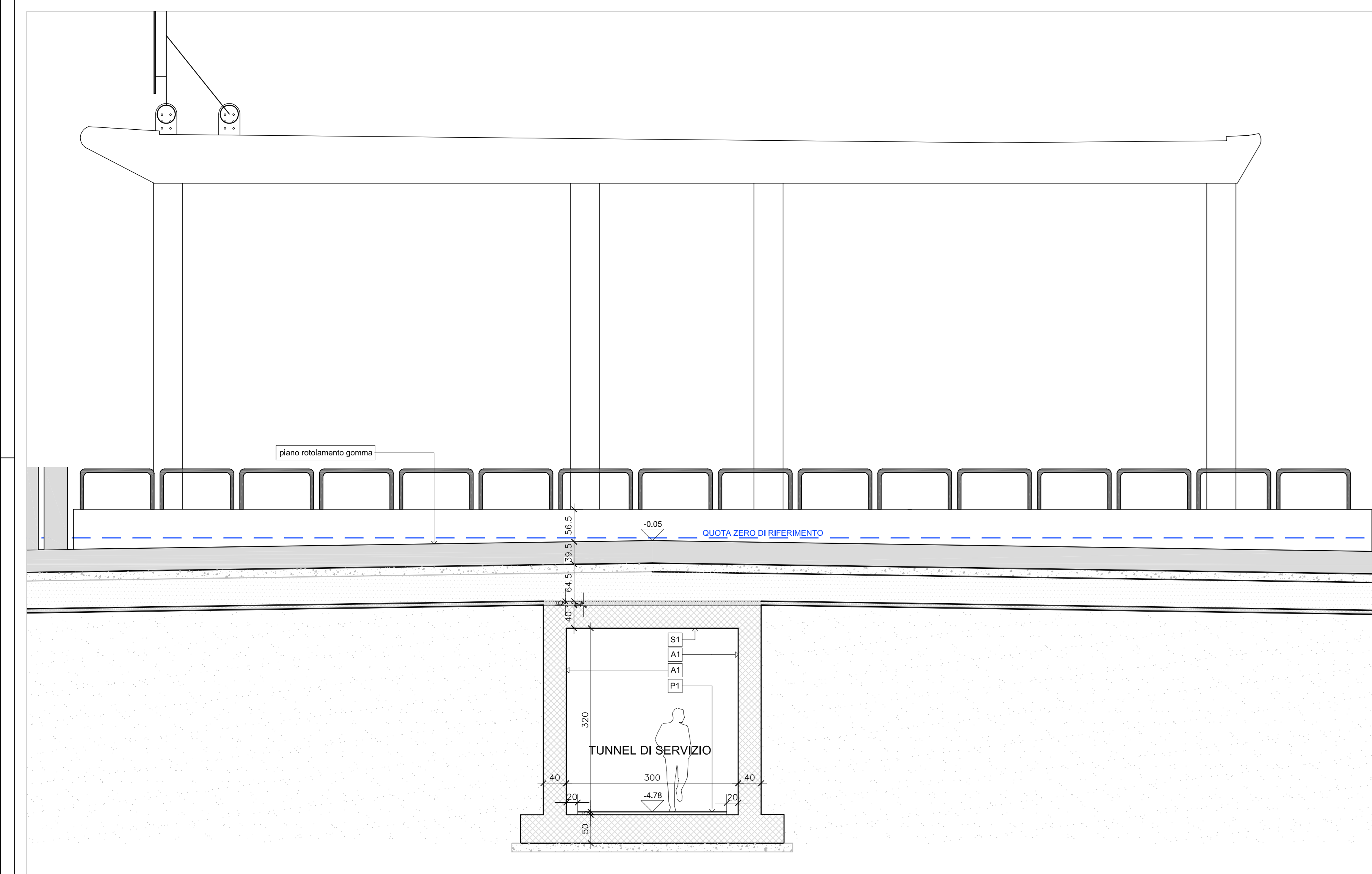
Sezione 1 - scala 1:50
