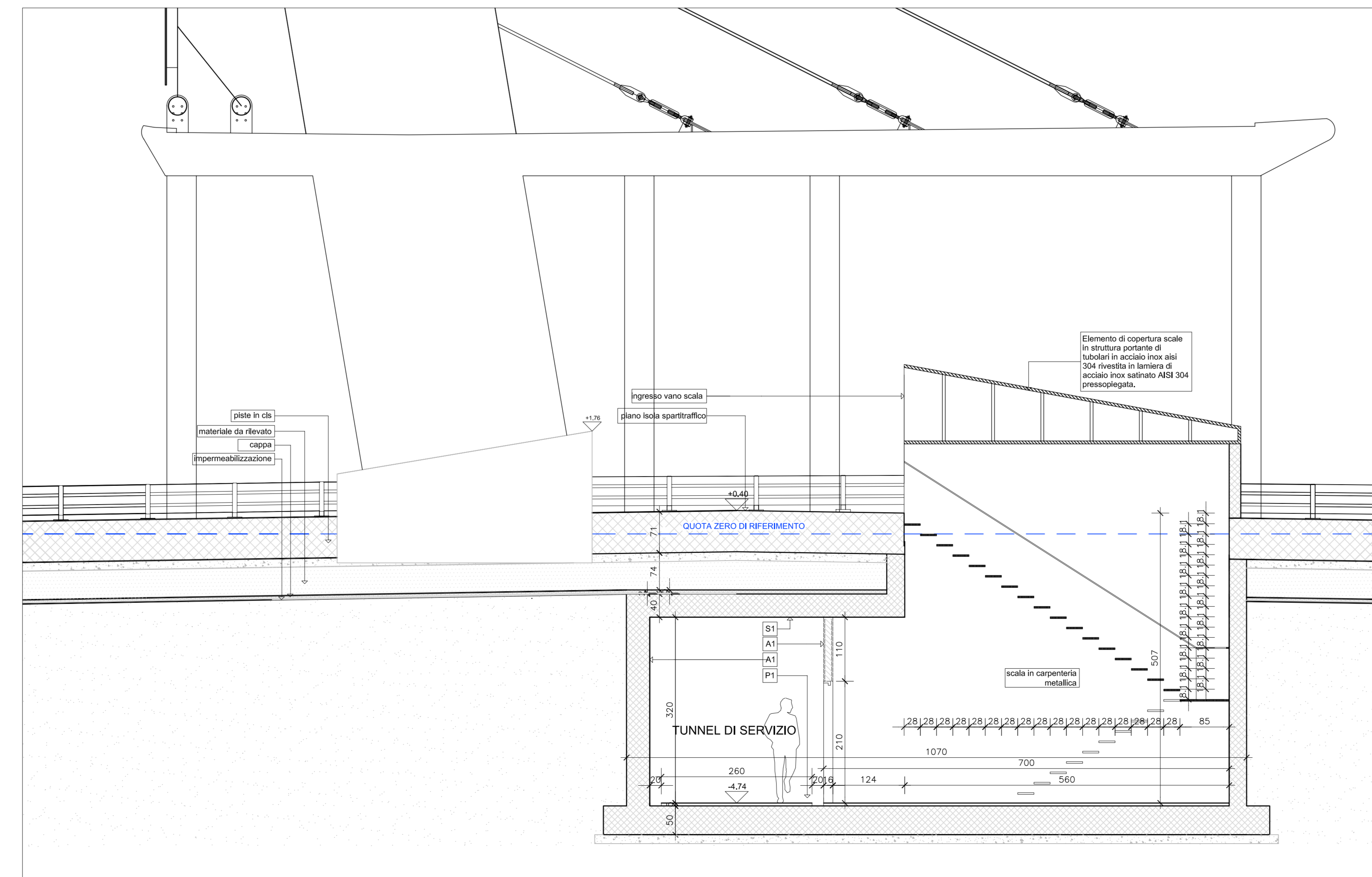
Sezione 4C - scala 1:50
