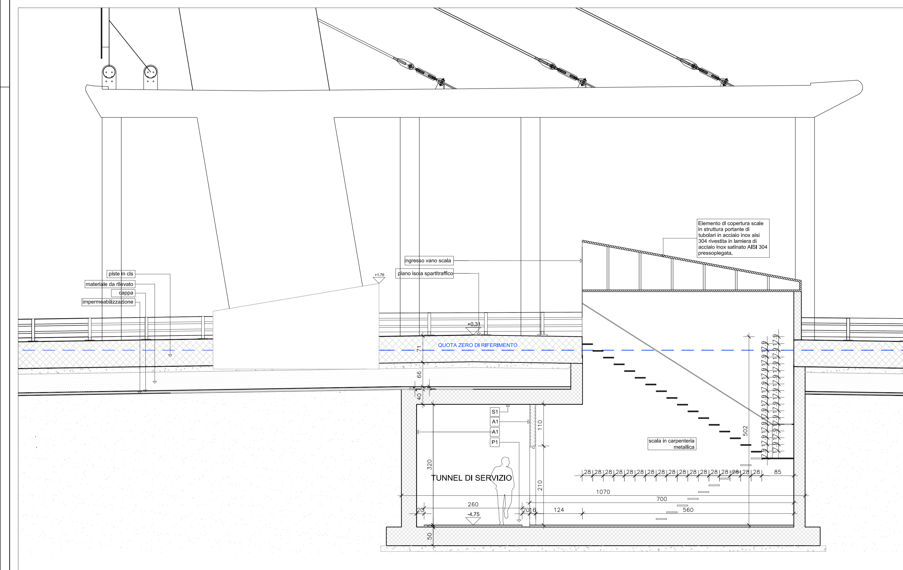
Sezione 4B - scala 1:50
