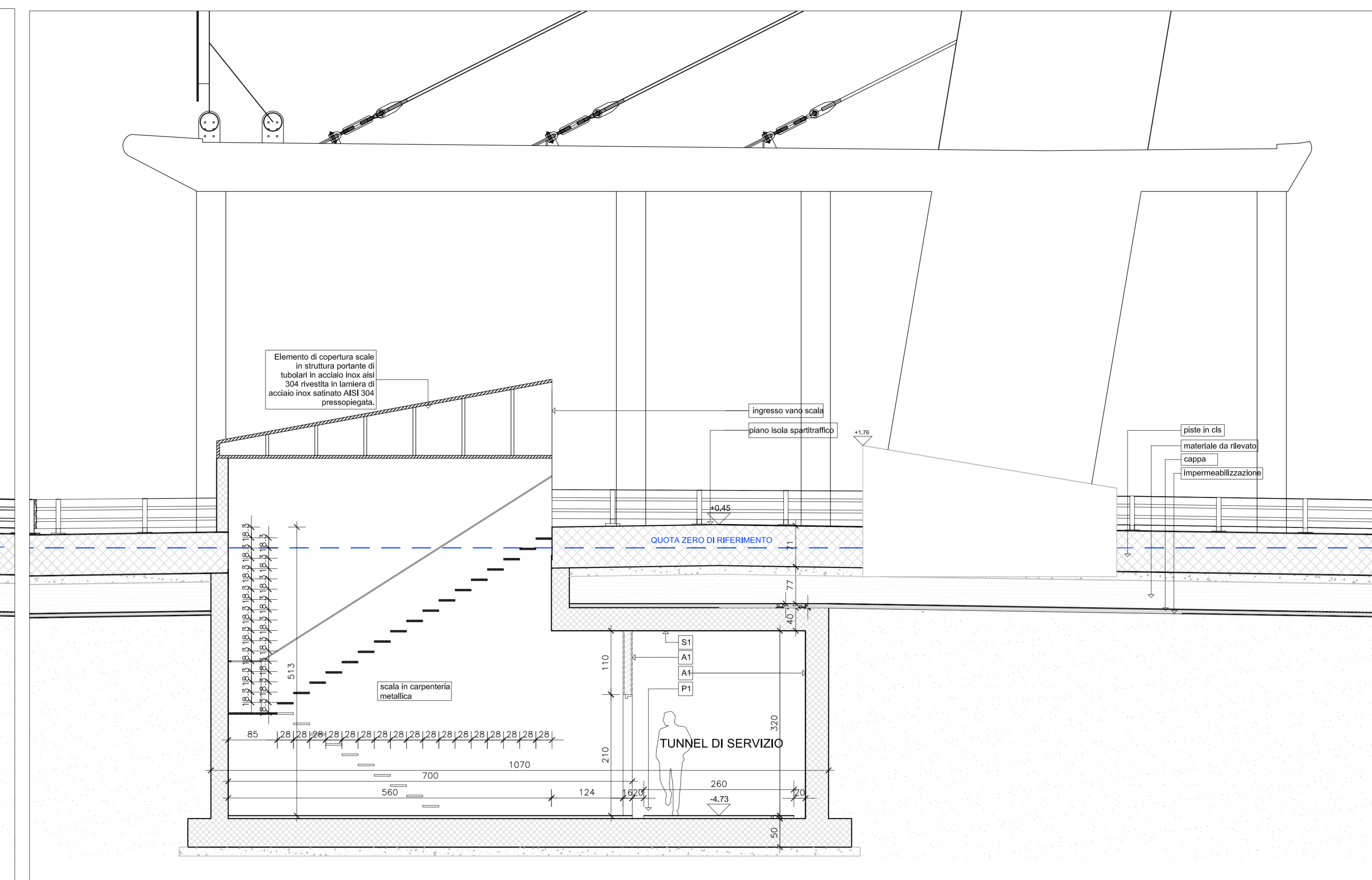
Sezione 3C - scala 1:50
