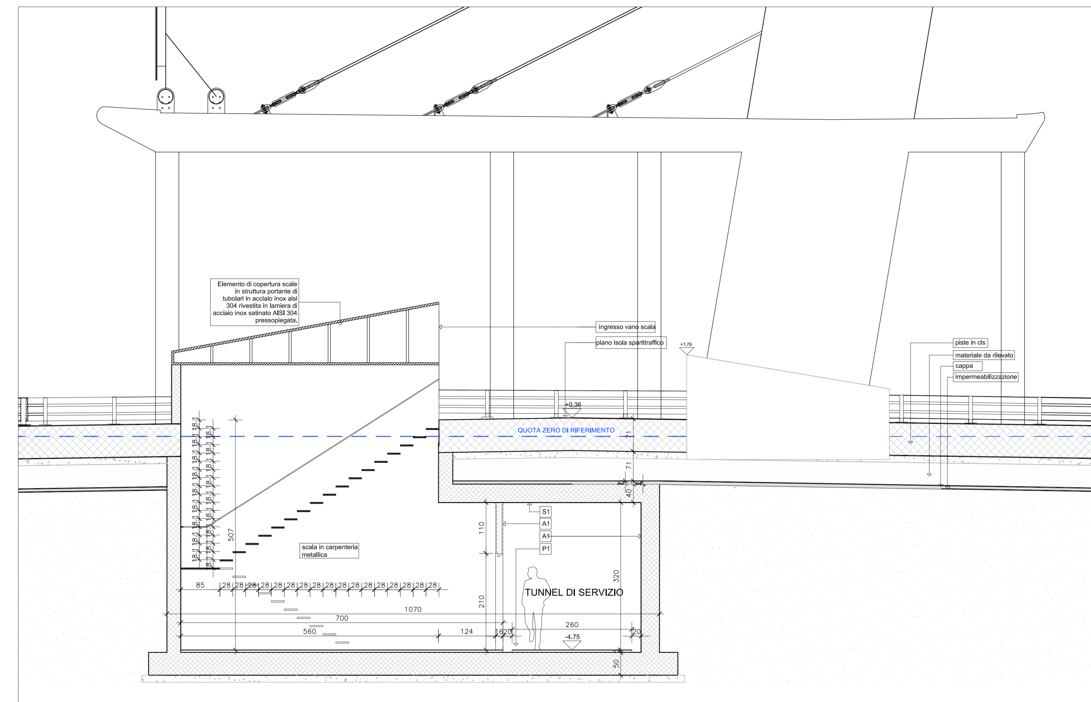
Sezione 3B - scala 1:50
