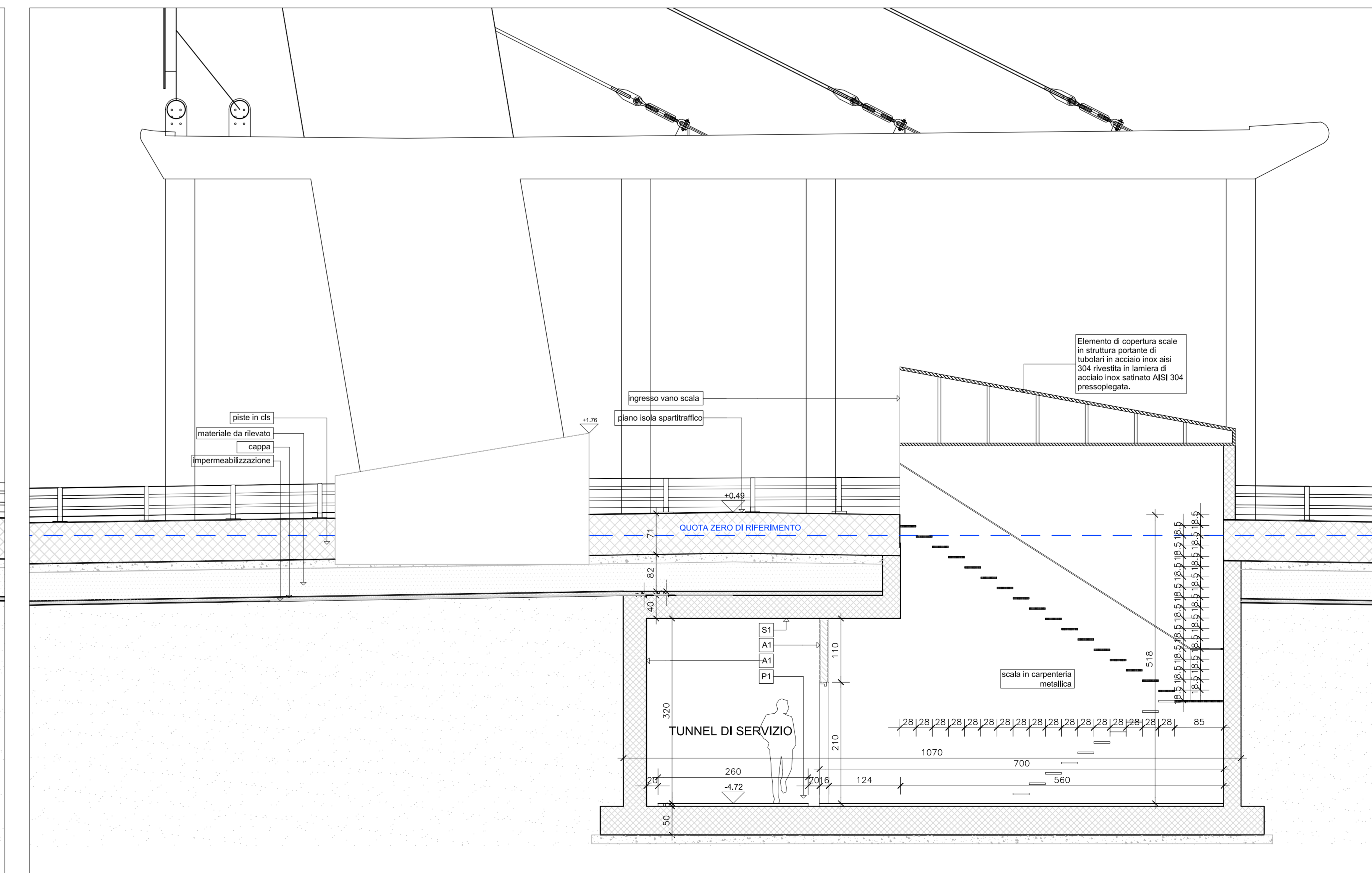
Sezione 4D - scala 1:50
