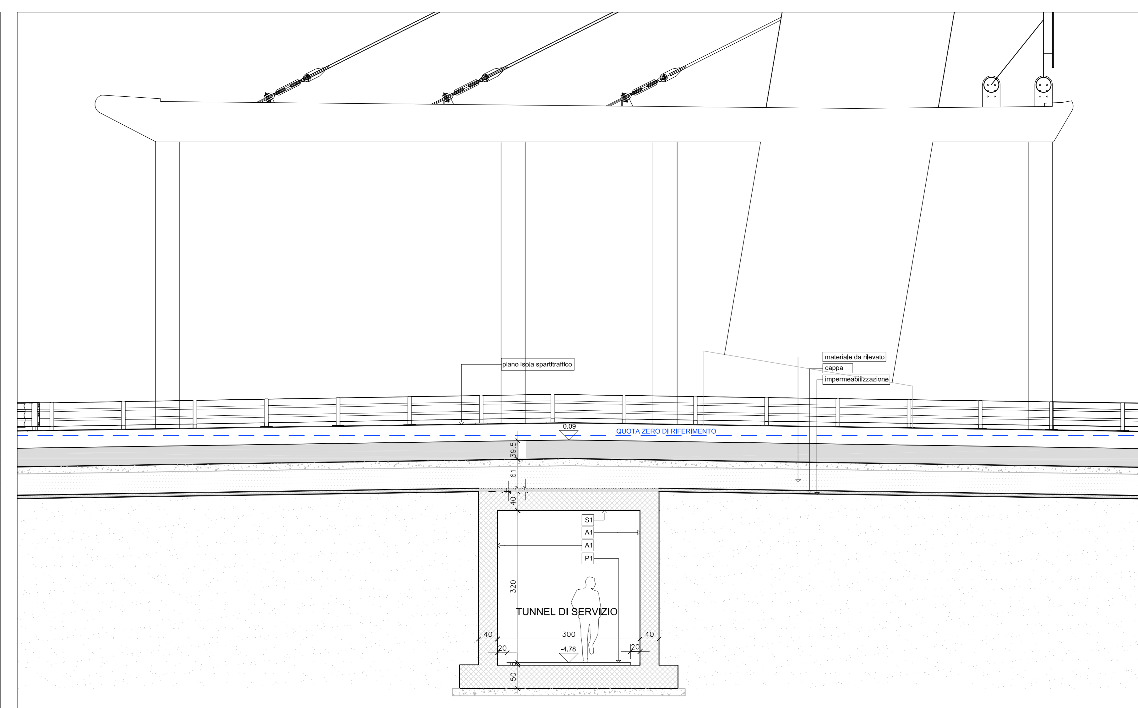
Sezione 12 - scala 1:50
