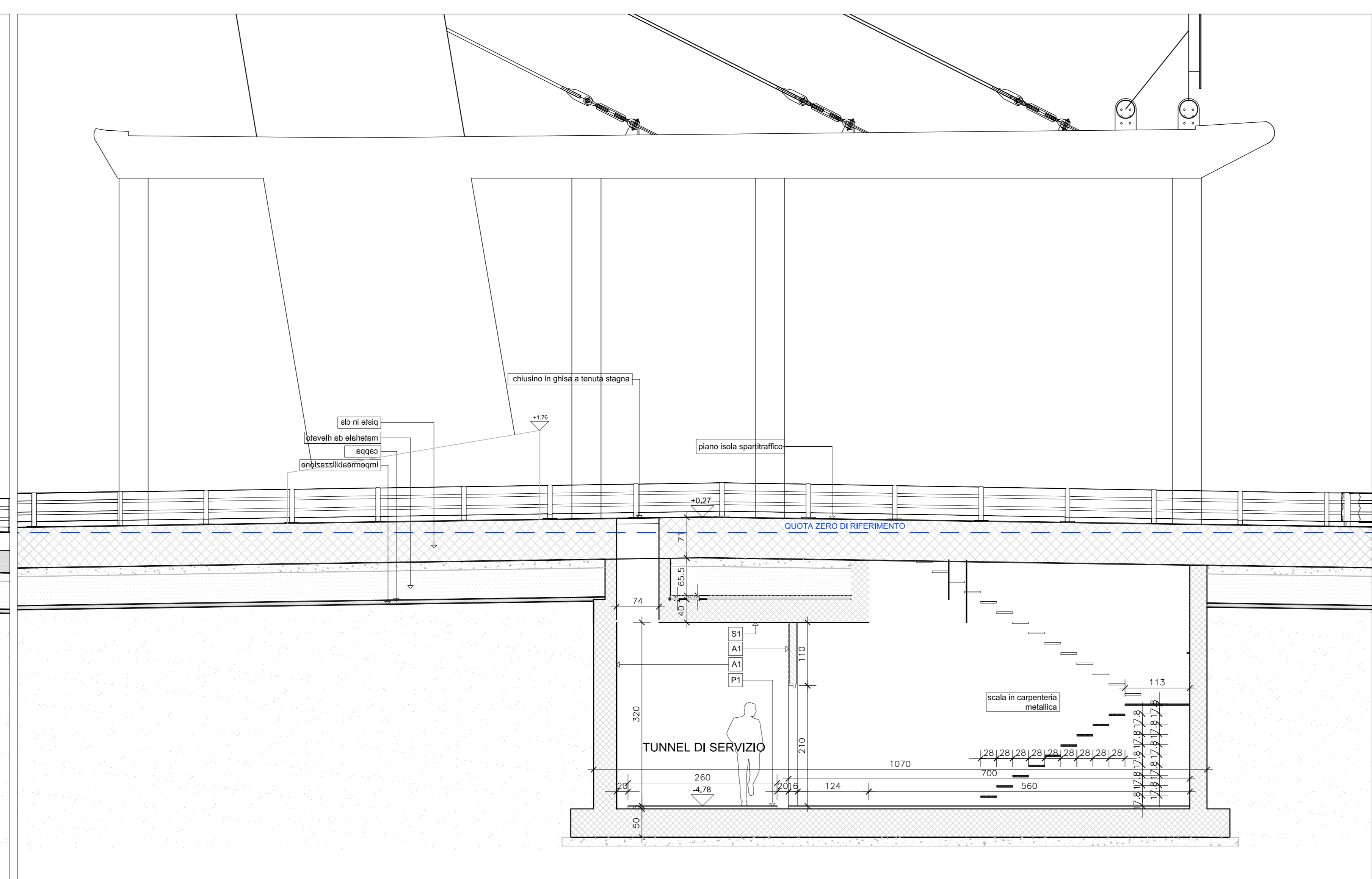
Sezione 8 - scala 1:50
