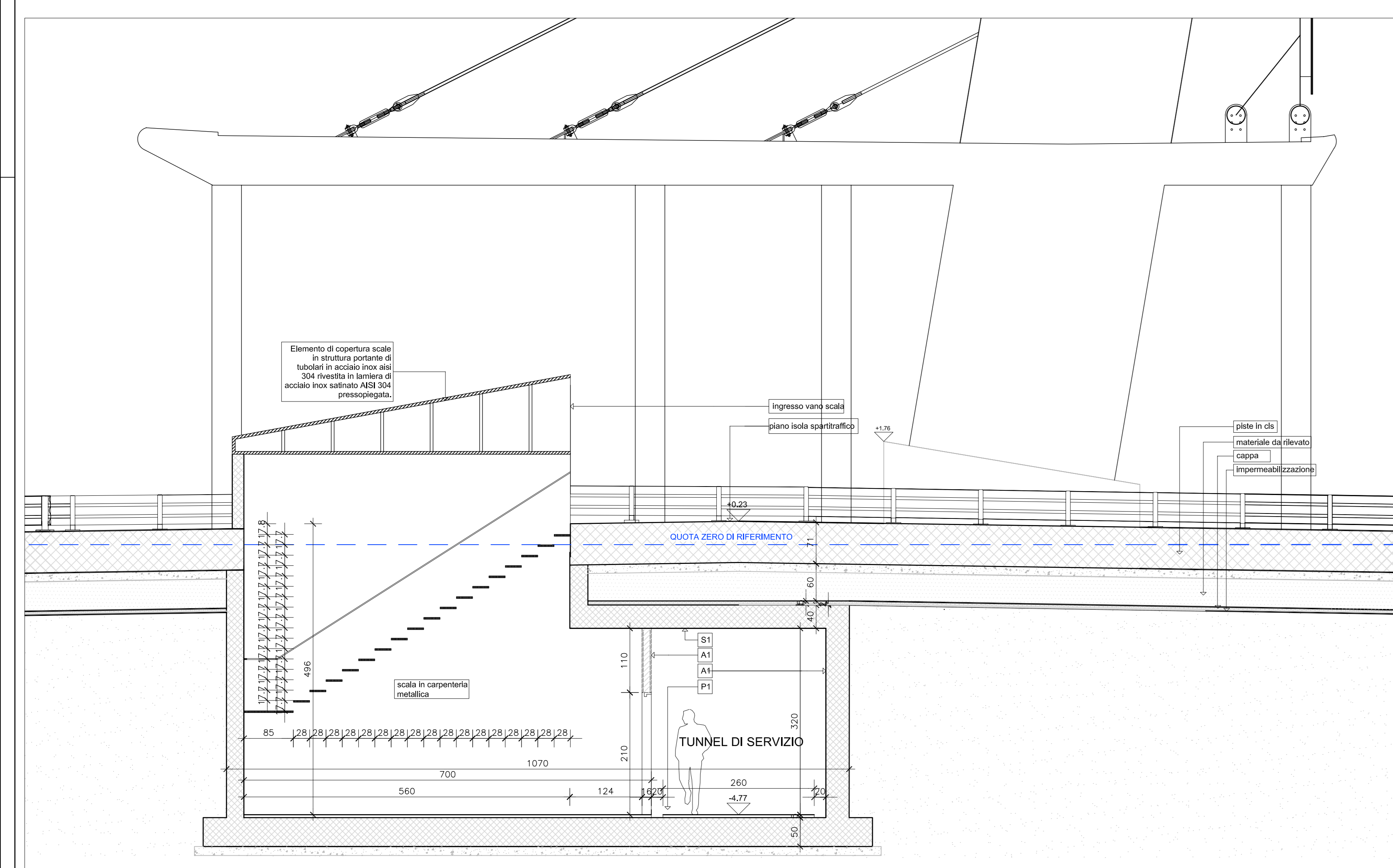
Sezione 10A - scala 1:50
