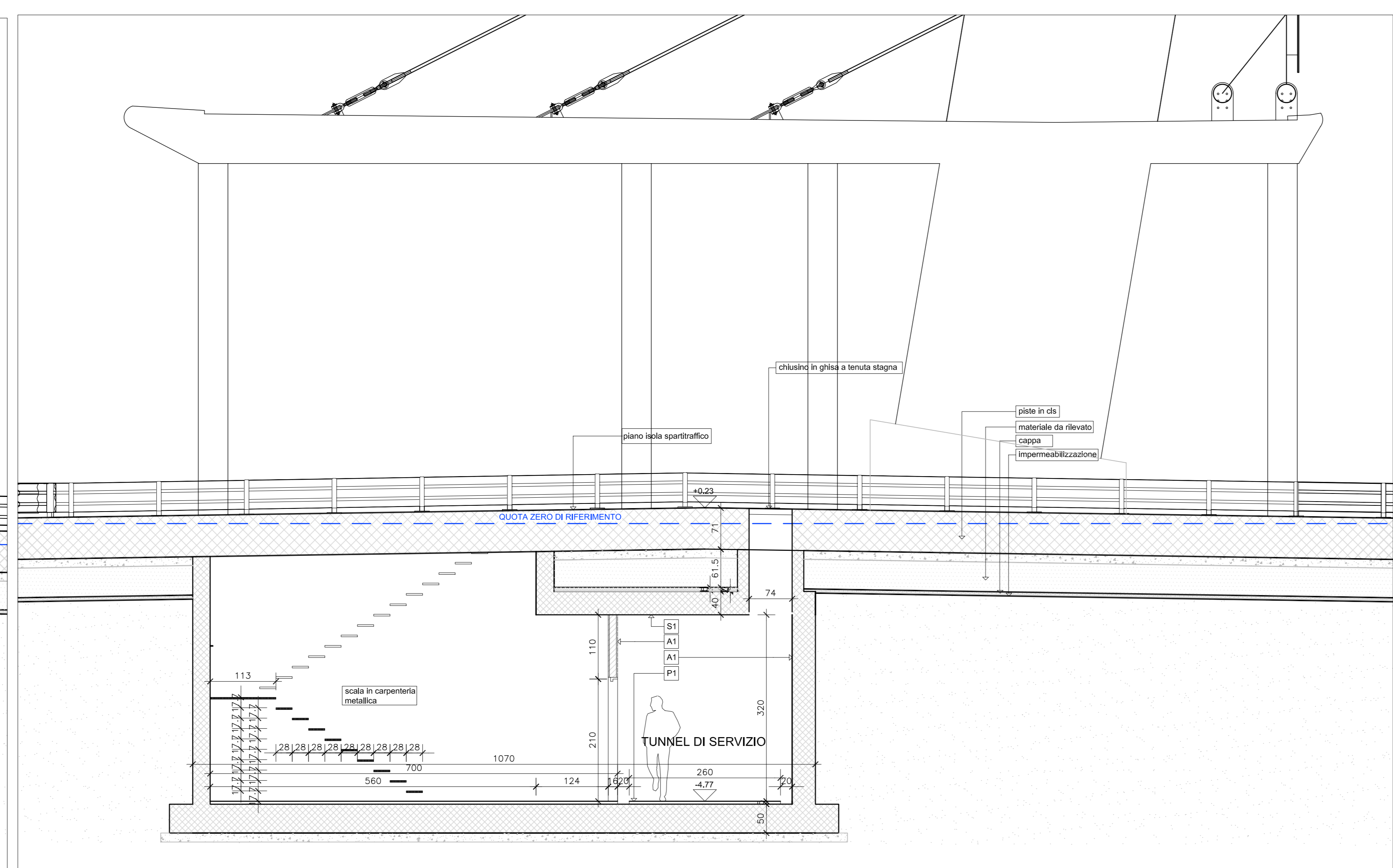
Sezione 11 - scala 1:50
