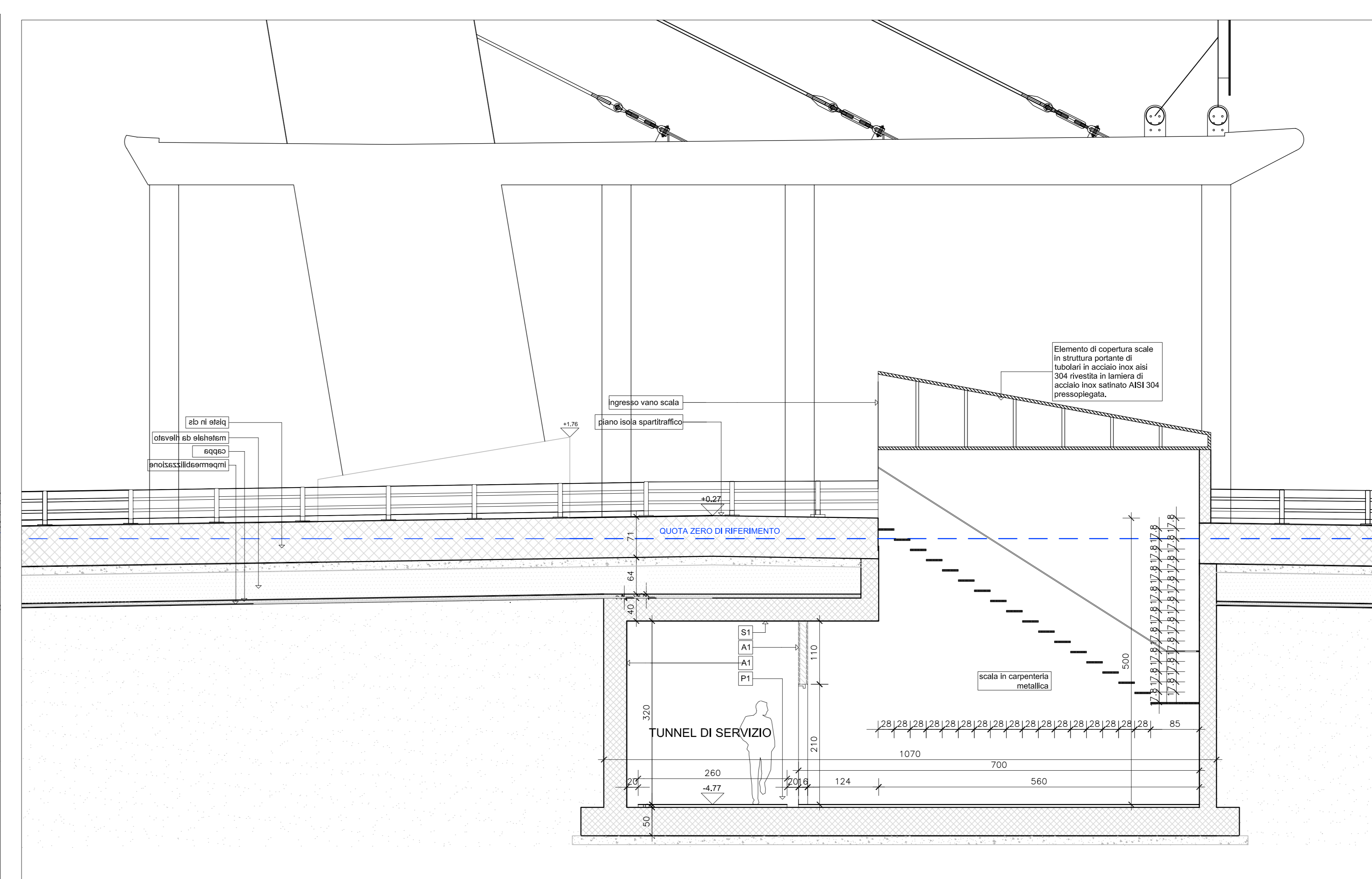
Sezione 9A - scala 1:50
