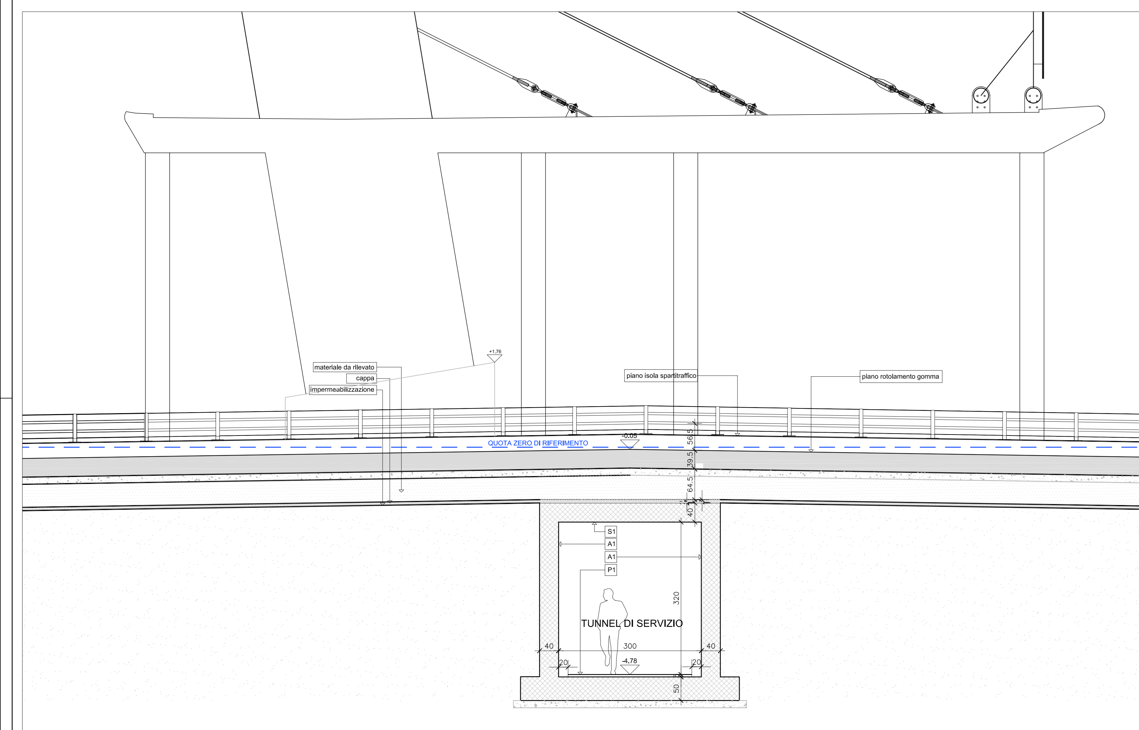
Sezione 7 - scala 1:50
