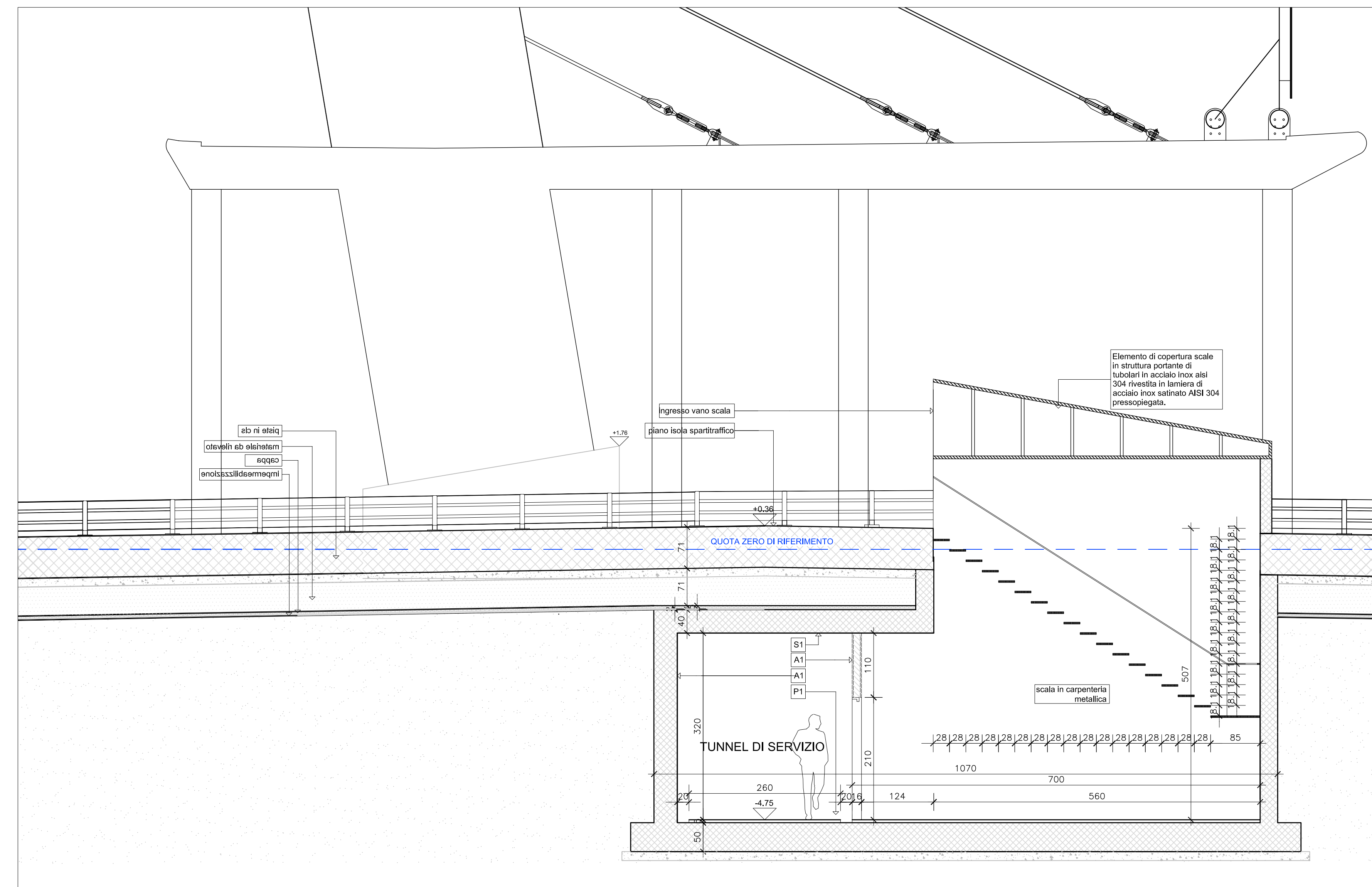
Sezione 9B - scala 1:50
