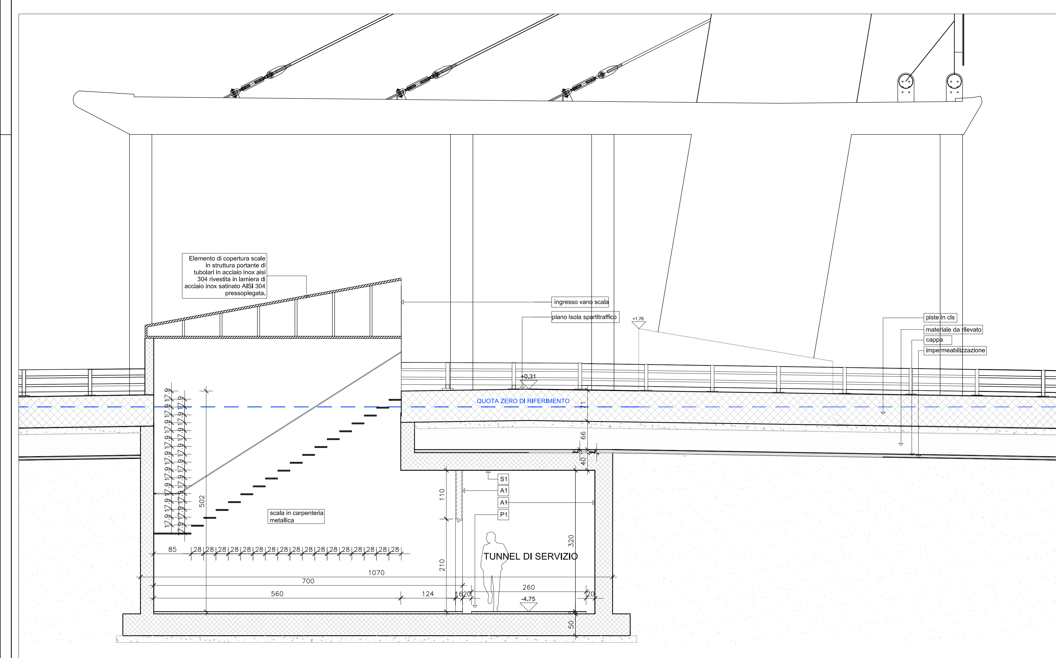
Sezione 10B - scala 1:50
