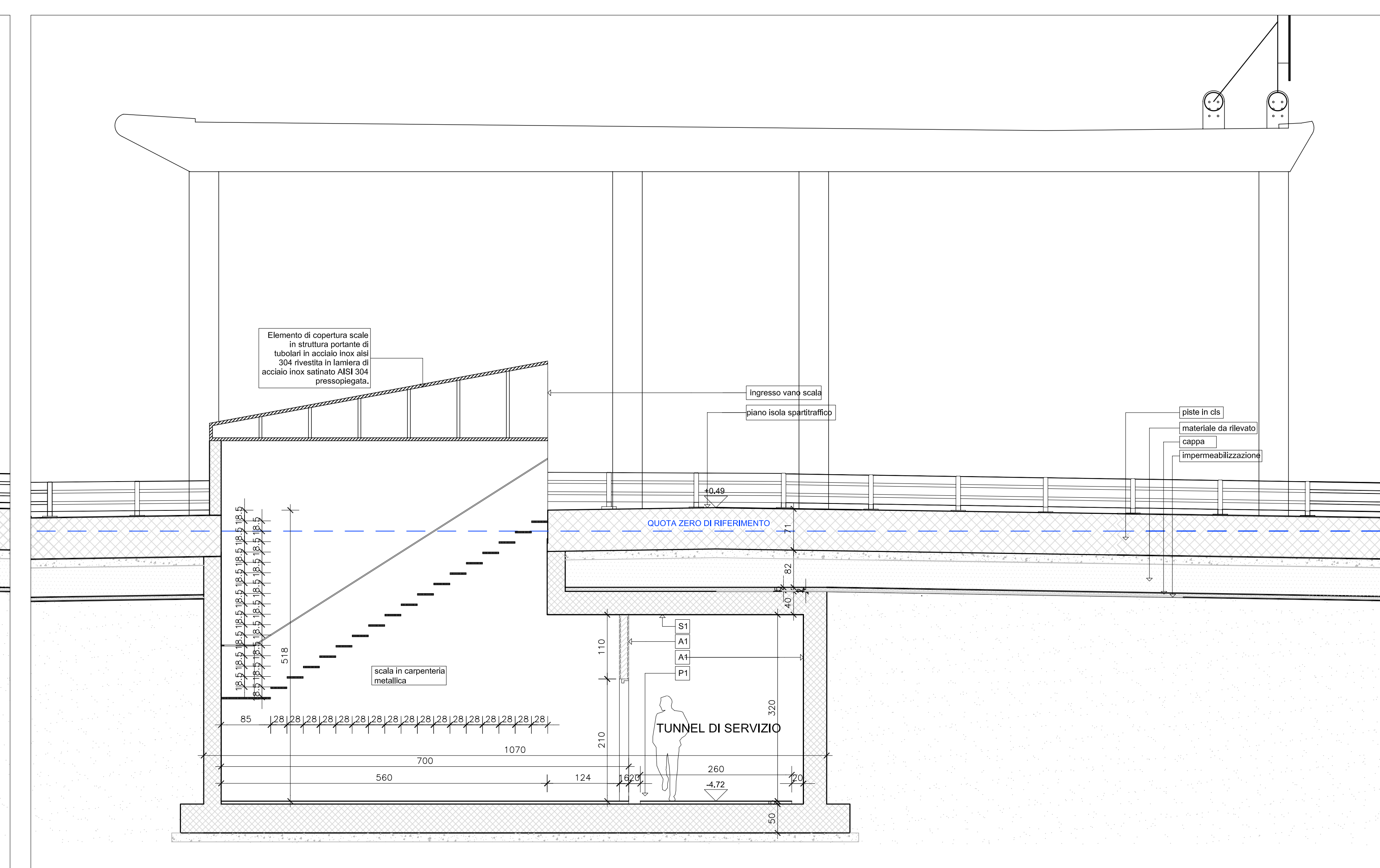
Sezione 10D - scala 1:50
