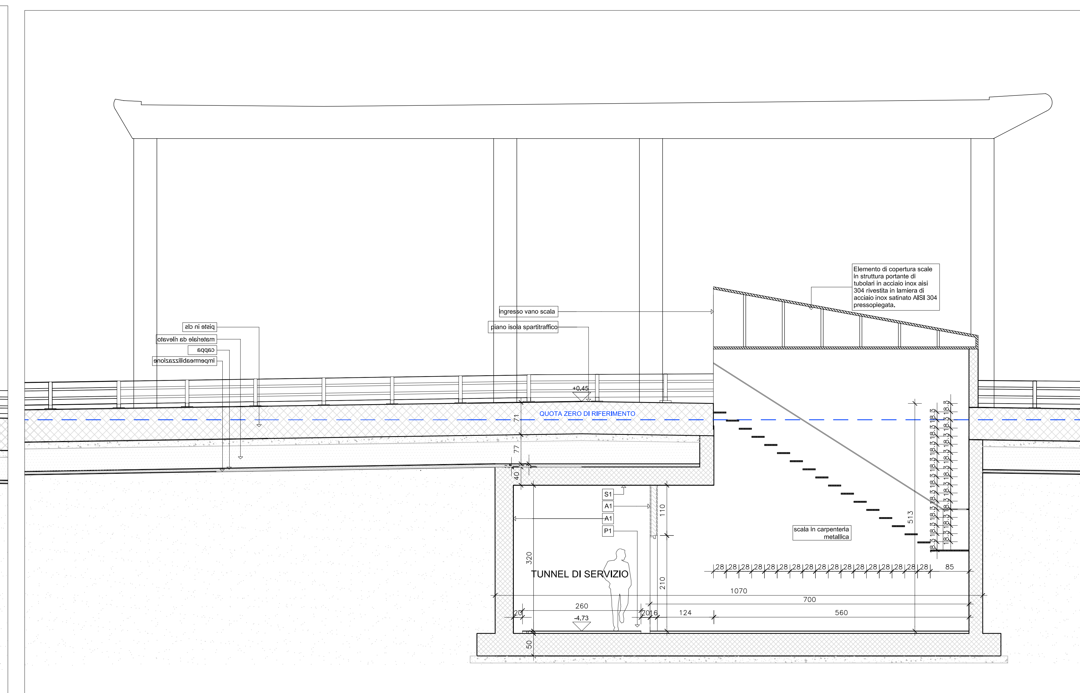
Sezione 9C - scala 1:50
