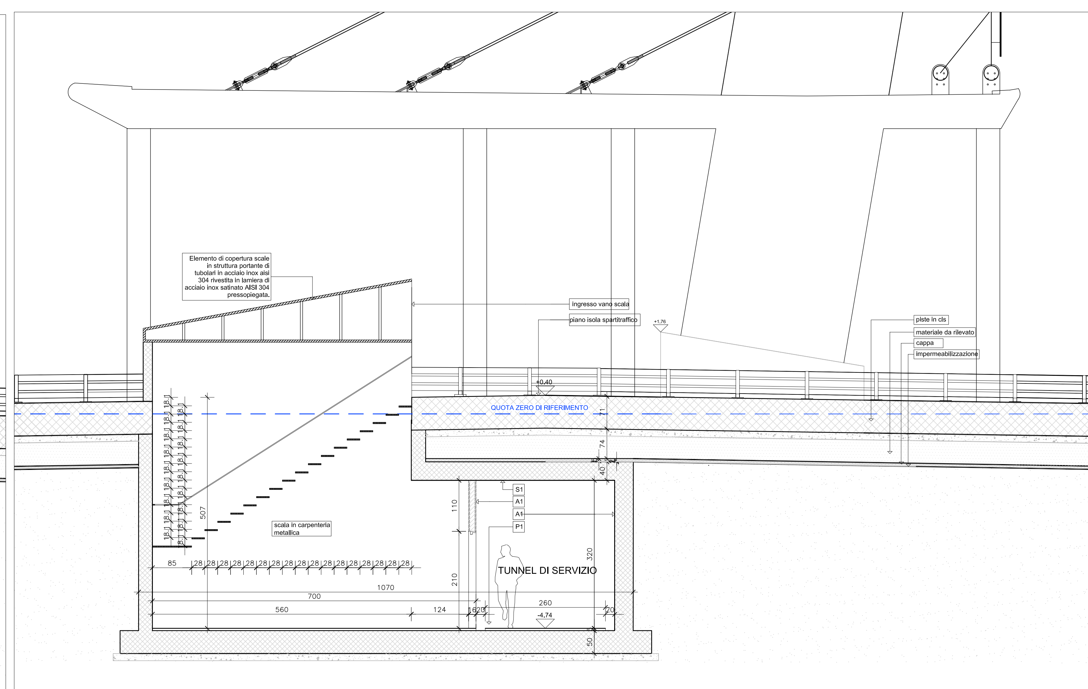
Sezione 10C - scala 1:50
