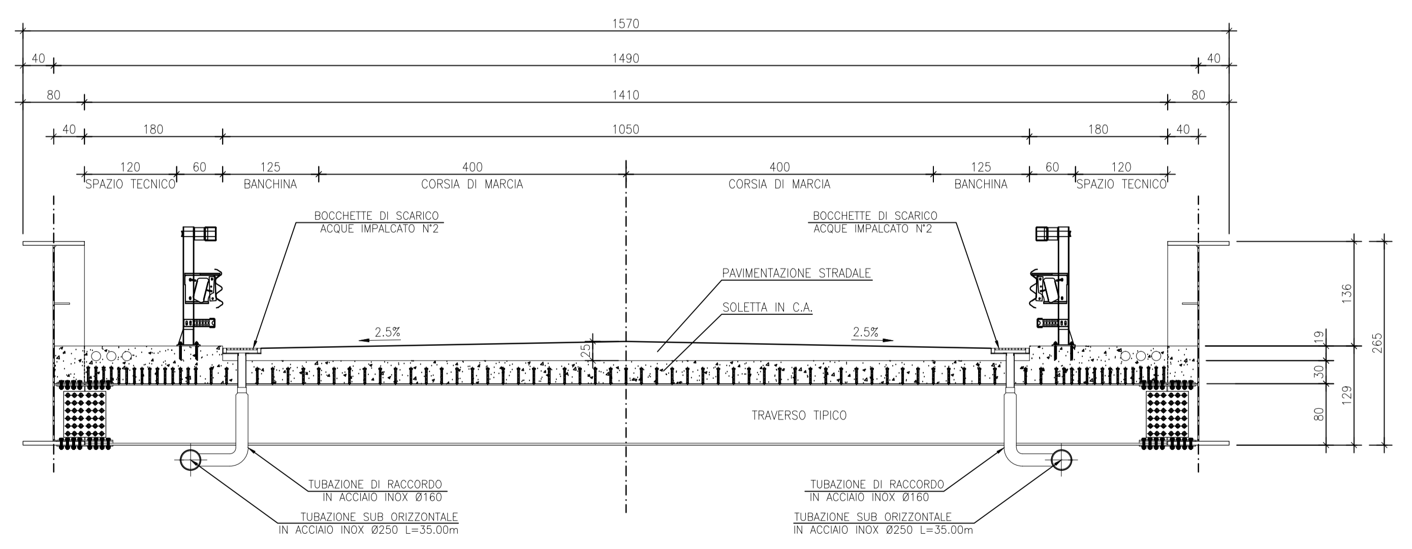
SEZIONE TIPO scala 1:50
