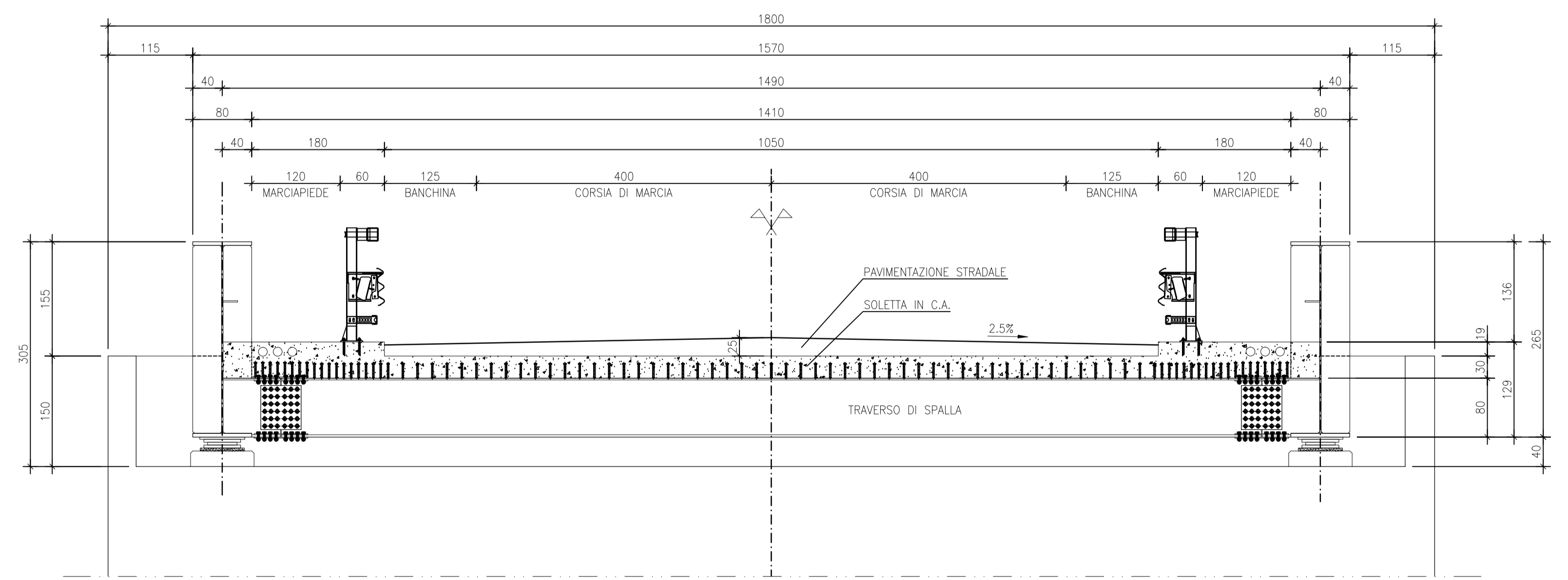
SEZIONE IN SPALLA scala 1:50
