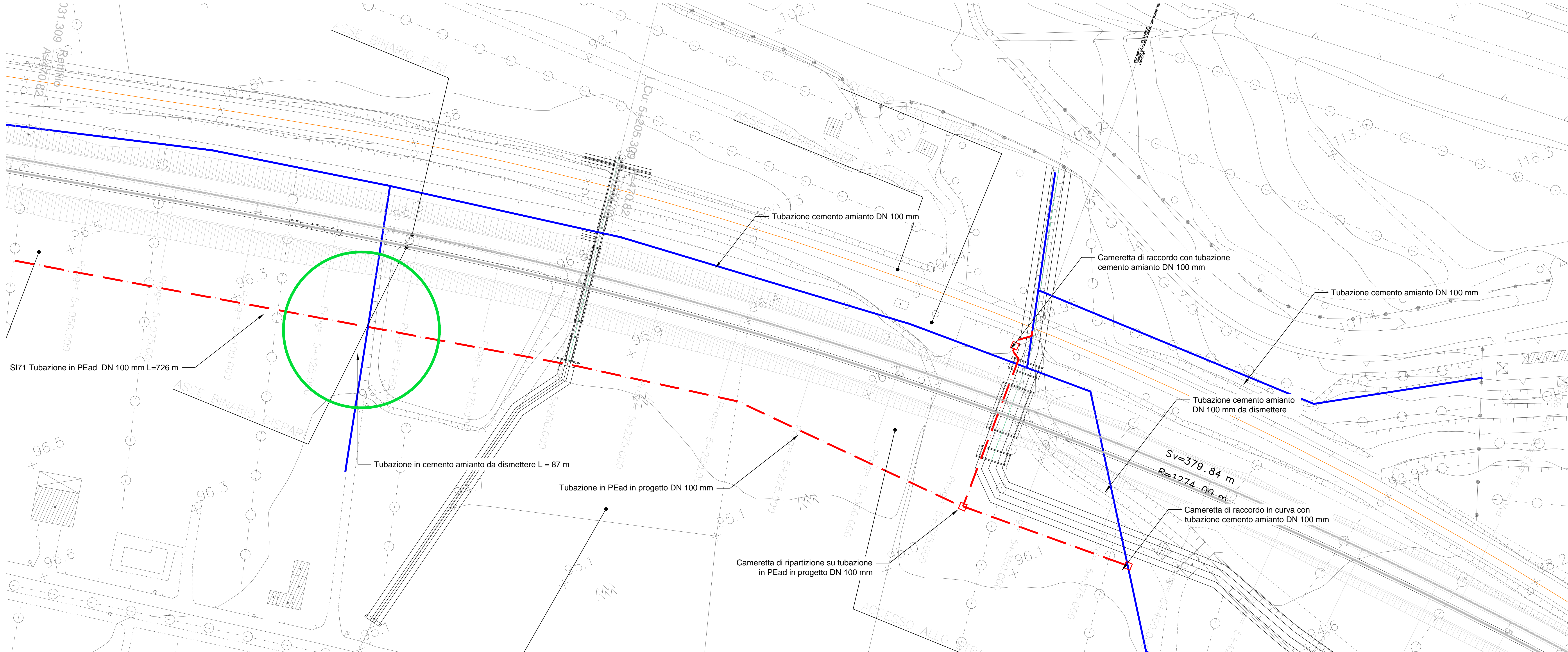
STRALCIO PLANIMETRICO 'INTERFERENZA' Consorzio di Bonifica 9 al Km 5+150- scala 1:500
